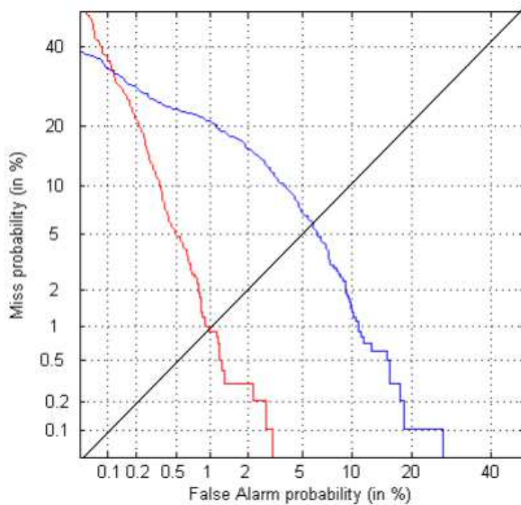
FIGURE 4.16 – Courbes DET pour les séries Min , Max , avec 47 hommes (987 comparaisons cible et 45 402 comparaisons imposteur) et des enregistrements de 2 minutes 30 de trames sélectionnées en apprentissage et de 30 secondes de trames sélectionnées en test, testées sur le système ALIZE/SpkDet : fluctuation de performance de 1.0% à 5.8%
