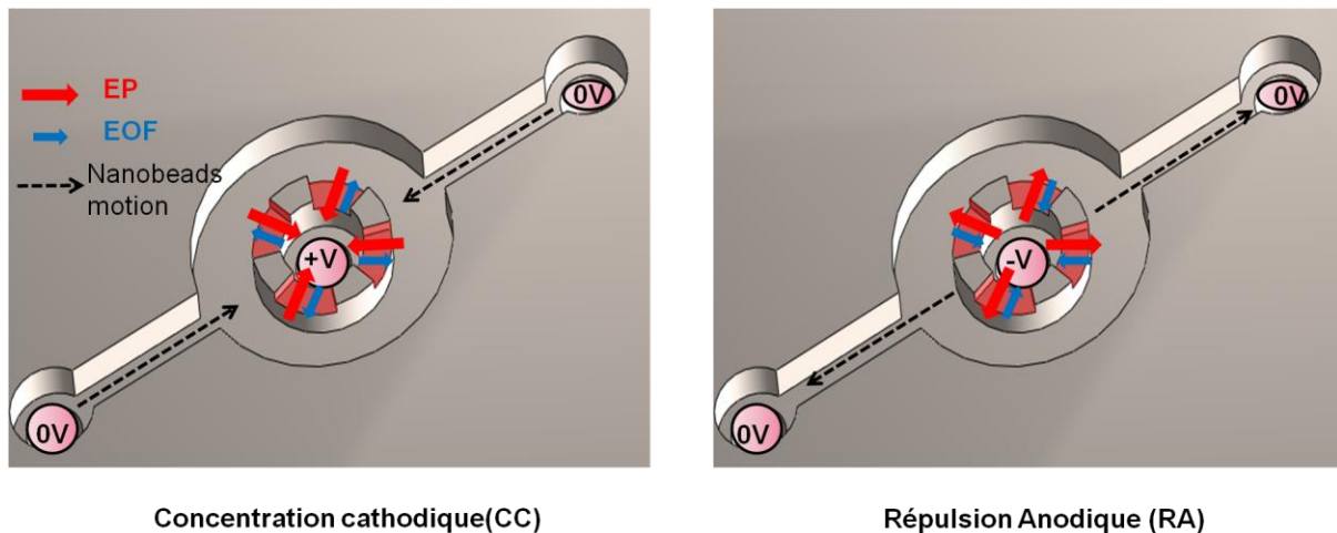
Figure 73 : Représentation 3D du système radial dans les régimes de Concentration Cathodique (CC) et de Répulsion Anodique (RA). (a) En régime CC l'entrée centrale est connectée à l'anode tandis que les deux entrées périphériques sont connectées à la masse. (b) En régime RA l'entrée centrale est connectée à la cathode tandis que les deux entrées périphériques sont connectées à la masse. Les flux électrophorétique (EP) et électroosmotique (EOF) sont représentés par les flèches rouges et bleus, respectivement. Les flèches en pointillées représentent le déplacement des particules résultant de la compétition entre ces deux flux.
