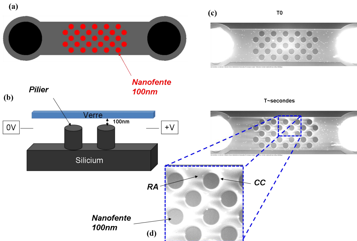
Figure 83 : Microsystème à pilier non scellés pour la préconcentration localisée. (a) Schéma du composant. (b) Vue en coupe du composant. Des tensions V supérieures à 100V sont générées. (c) Microscopie par fluorescence de l'effet de répulsion et de concentration de fluorescéines. (d) Zoom sur une région où plusieurs zones RA et CC sont générées au niveau de chaque pilier.
