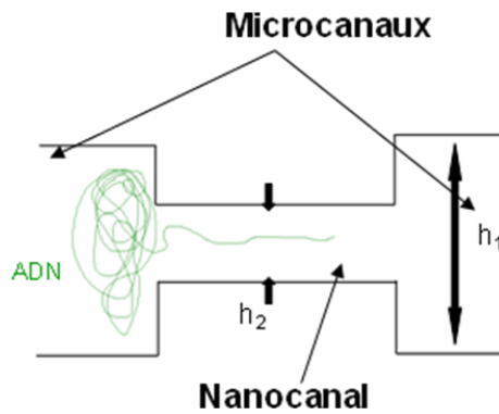
Figure 14: Schéma décrivant le phénomène de confinement entropique.
