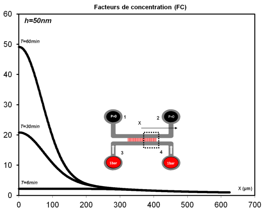
Figure 55: Modélisation du profil de la concentration normalisée C/C_0 (Facteur de concentration FC) dans la direction x dans le système bypass de référence B0 pour h=50\text{nm} et pour une pression de 1bar.
