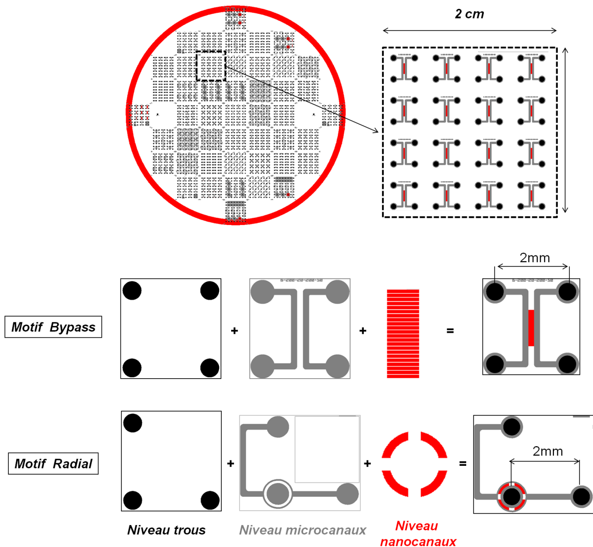
Figure 31 : Superposition des trois niveaux de masques 200mm dessinés sur le logiciel AUTOCAD. Ce sont la reproduction exacte des masques physiques Chrome/Quartz utilisés lors des étapes de photolithographie. Sur un wafer de 200mm sont gravées 47 puces en silicium, de 2cm 2 chacune, comprenant chacune en moyenne 16 composants de motifs identiques ou différents. Les deux principaux composants (bypass et radial) sont décomposés selon leur trois niveaux de gravure.
