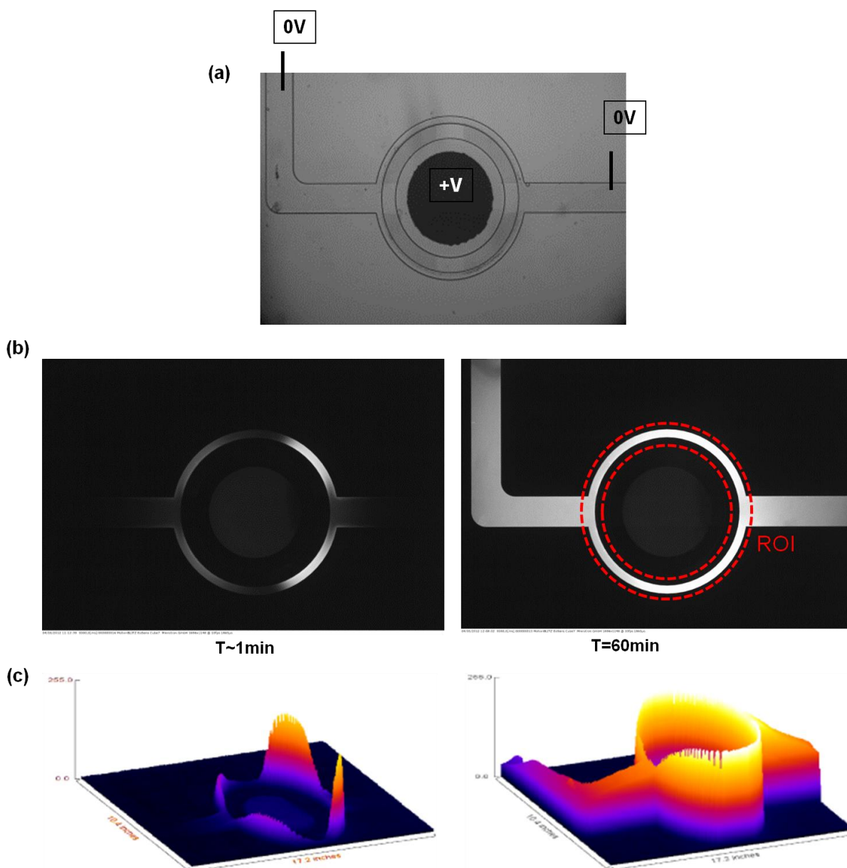
Figure 74: Electropréconcentration cathodique de nanobilles de polystyrènes de 50nm diamètre dans le système micro-nanofluidique radial. (a) Description du mode d'actionnement électrocinétique du dispositif dans le régime CC. (b) Imagerie par fluorescence aux instants T=1\text{min} et T=60\text{min} . En pointillé la zone de mesure ROI. La surface de la ROI est sensiblement la même que celle utilisée dans le cas des mesures du facteur de concentration dans le système bypass actionné dans le mode Symétrique électrocinétique. (c) Représentations 3D, obtenues grâce au logiciel image J, de l'intensité de fluorescence dans le système.
