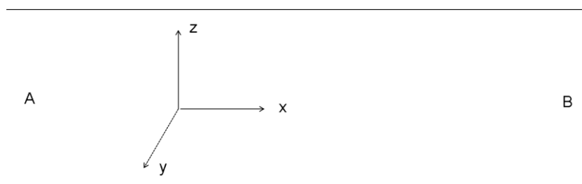
Figure 1 : Schéma simple représentant l'orientation des trois directions de l'espace dans un canal orienté suivant la direction x . En A (entrée du canal) et B (sortie du canal) des pressions P_A et P_B ou des tensions V_A et V_B peuvent être appliquées.
