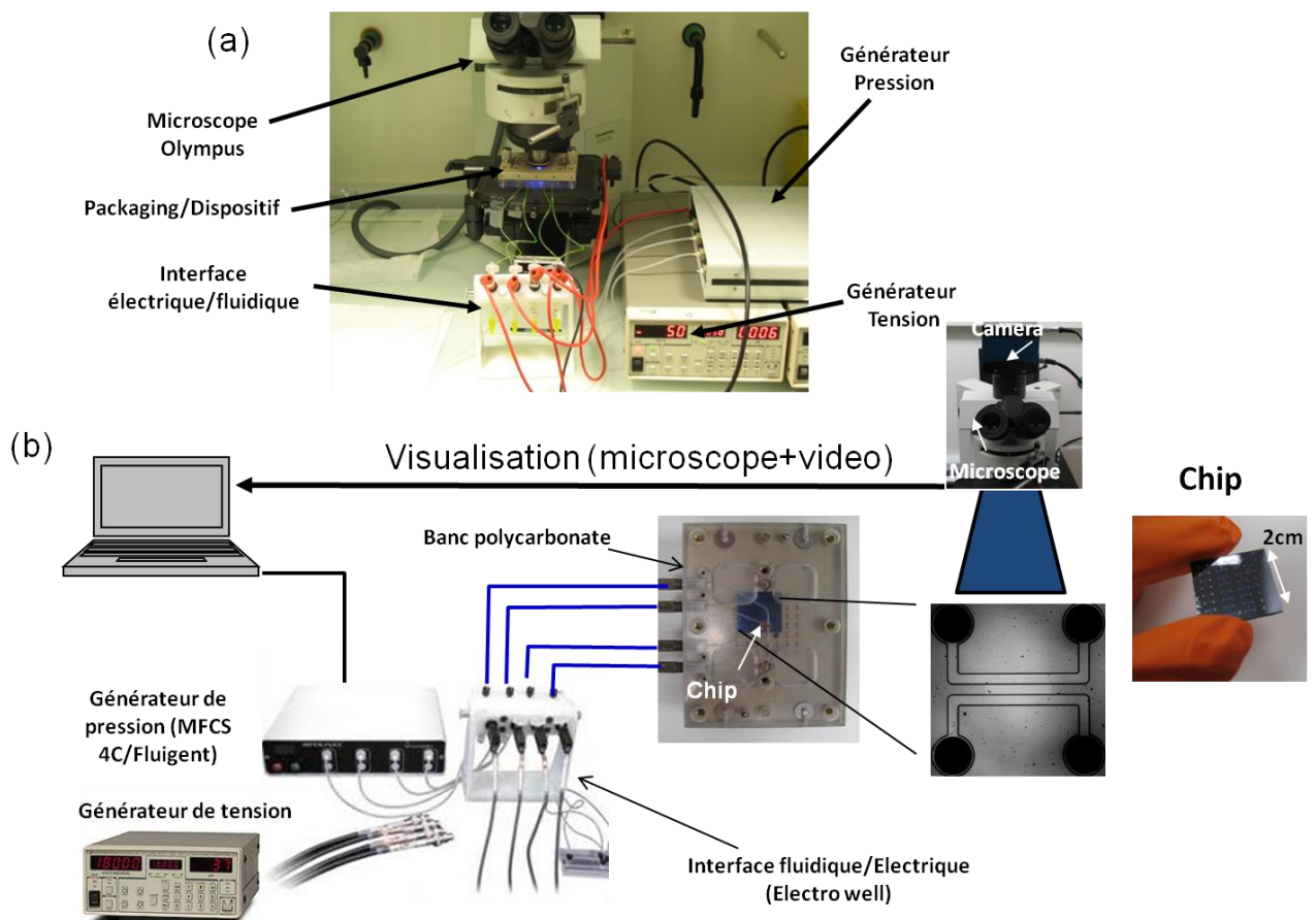
Figure 39 : (a) Photographie du montage expérimental. (b) Schéma du montage expérimental avec les accessoires principaux.
