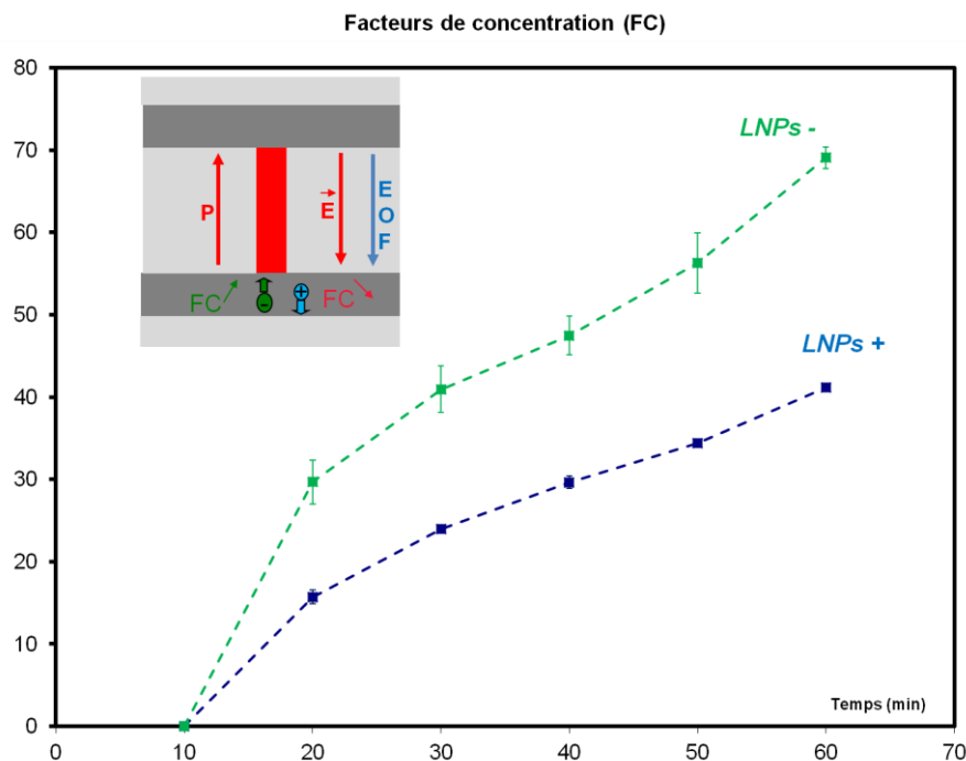
Figure 62: Mise en évidence d'un potentiel d'écoulement. La pression génère un champ électrique E à travers la rangée de nanocanaux. La mesure du facteur de concentration pour des particules lipidiques cationiques est représentée par la courbe rouge et des particules anioniques par la courbe bleu. L'augmentation du facteur de concentration (FC) est favorisée pour les particules négatives qui sont attirées vers la nanojonction grâce à l'électrophorèse et à l'écoulement hydrodynamique. En revanche, dans le cas des particules positives, les forces électrophorétiques et l'écoulement hydrodynamique s'opposent, réduisant ainsi les FC.
