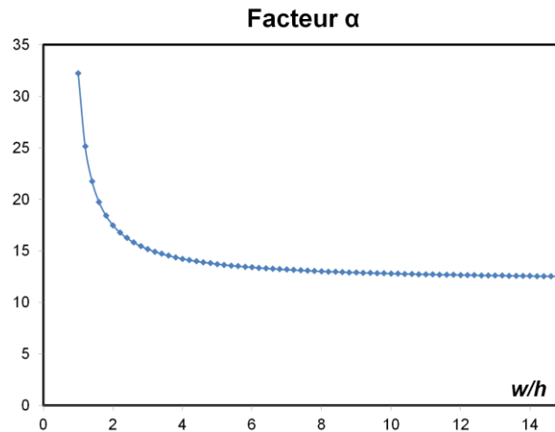
Figure 2 : Evolution du facteur de forme \alpha = \frac{12}{1 - 0.63(\frac{h}{w})} en fonction du rapport entre la largeur w et la hauteur h du canal considéré. Lorsque la largeur est très grande devant la hauteur on retrouve la valeur limite du facteur \alpha = 12 .
