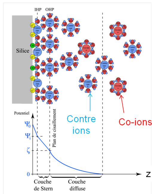
Figure 3: Illustration de la double couche électrique à la paroi d'une interface de \text{SiO}_2 d'après le modèle de Stern et schématisation de l'évolution du potentiel électrique au voisinage de la surface le long de l'axe z . 12
