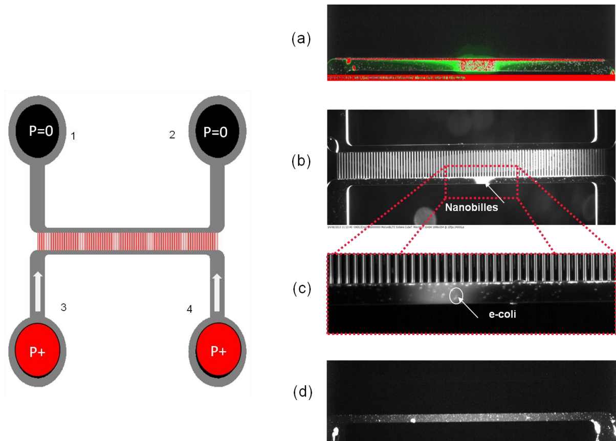
Figure 80 : Actionnement Symétrique hydrodynamique d'un système bypass pour la colocalisation de deux populations de particules de tailles différentes. L'objectif est de l'utiliser à terme, comme un module d'optimisation d'une étape de transfection cellulaire. (a) Préconcentration visualisée par microscopie de fluorescence. Les nanobilles en polystyrène de 50nm émettent dans le vert et les microbilles de 1 \mu m dans le rouge. (b) Colocalisation, visualisée en fond noir, de nanobilles de polystyrène de 50nm et de bactéries e-coli. (c) Même image à temps d'exposition plus faible pour visualiser les bactéries dans la zone de concentration. (d) Effet d'enrichissement de nanobilles de 50nm dilué dans du plasma sanguin total.
