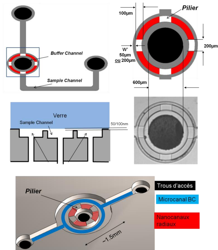
Figure 37: (a) Vue de dessus du composant micro-nanofluidique radial et détail des dimensions caractéristique 2D de la micro-nanojonction. (b) Vue en coupe et (c) représentation 3D du composant.
