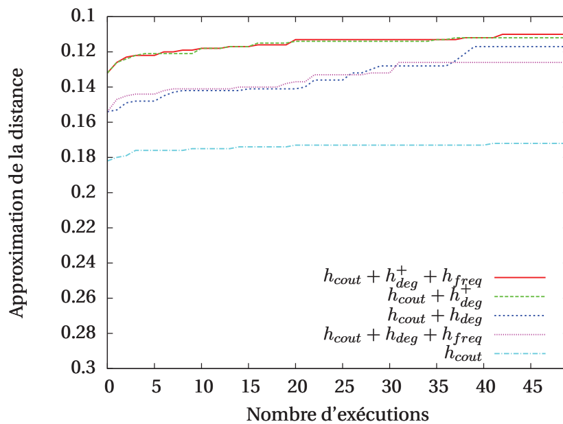
FIGURE 5.16 – Évaluation des heuristiques pour approximer la distance d_{mcs}^{p,1,1} sur le jeu de données Noyau 2500 , soit un noyau de 50%. Pour chaque nombre d'exécutions x \in [1; 50] , les courbes donnent la plus petite approximation calculée sur les x exécutions (en moyenne pour les 50 couples de 3G-cartes du jeu de données.)
