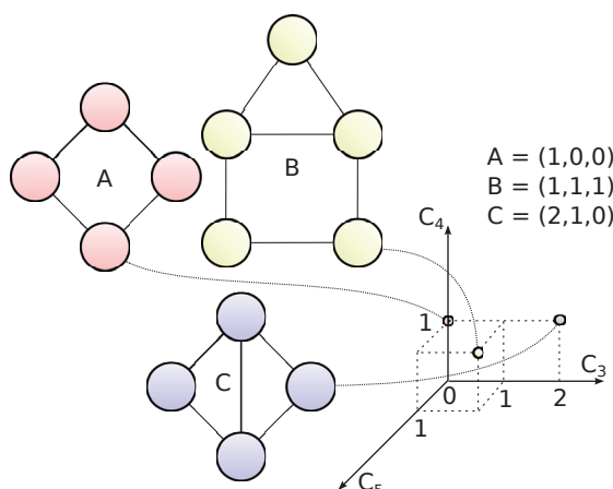
FIGURE 2.8 – Illustration de plongement de graphes dans un espace 3D, sur les trois axes. Nous représentons le nombre de cycles élémentaires de taille 3, 4 et 5 des graphes. Le vecteur pour chaque graphe est donc G = (C_3, C_4, C_5) ou C_i est le nombre de cycles élémentaires de taille i .
