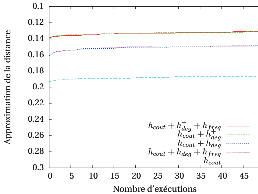
FIGURE 5.15 – Évaluation des heuristiques pour approximer la distance d_{mcs}^{p,1,1} sur le jeu de données Noyau 1000 , soit un noyau de 20%. Pour chaque nombre d'exécutions x \in [1; 50] , les courbes donnent la plus petite approximation calculée sur les x exécutions (en moyenne pour les 50 couples de 3G-cartes du jeu de données.)
