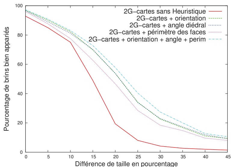
FIGURE 6.25 – Proportion de brins bien appariés en fonction du taux de dégradation (en pourcentage de brins) de la 2G-carte modélisant le maillage. Les courbes représentent les résultats obtenus en fonction des différentes étiquettes considérées pour les 2G-cartes.
