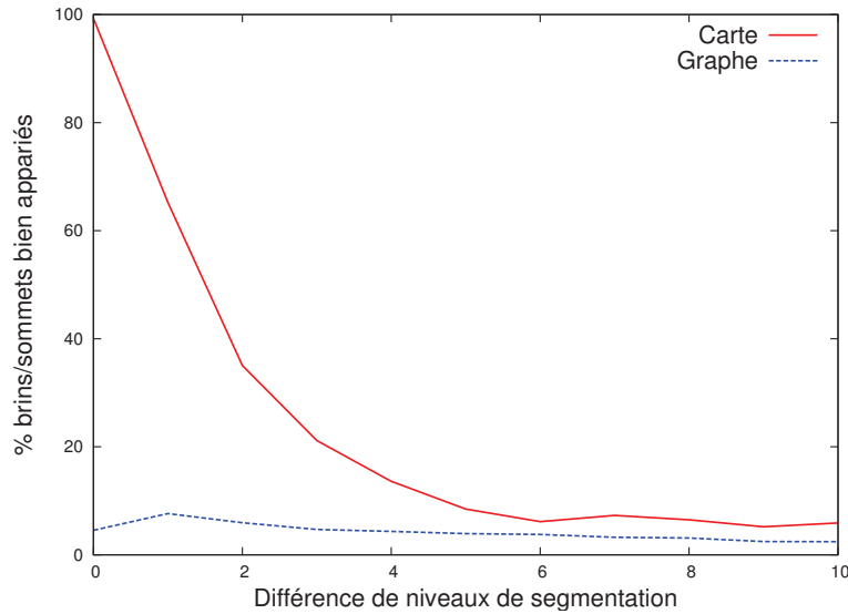
FIGURE 6.10 – Taux de brins/sommets appariés de façon cohérente par rapport au nombre de segmentation existant entre les deux images segmentées comparées. On compare la segmentation i et la segmentation i + j , j étant représenté en abscisse.
