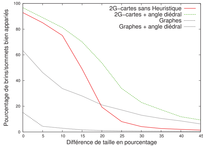
FIGURE 6.24 – Proportion de brins et sommets bien appariés en fonction du taux de dégradation (en pourcentage de brins) de la 2G-carte modélisant le maillage. Les courbes représentent les résultats obtenus en fonction des différentes étiquettes considérées avec les graphes et les 2G-cartes.
