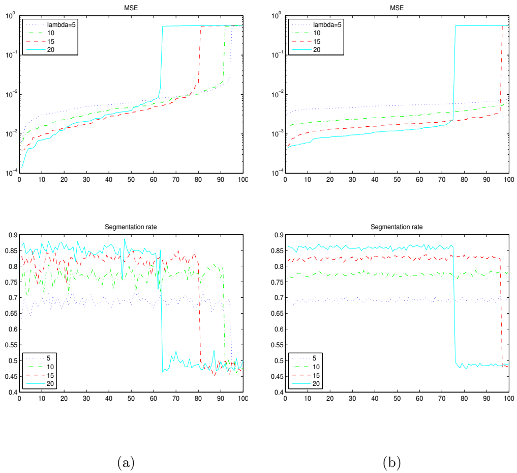
FIGURE 4.5 – Valeurs de l'EQM présentés en incrémentant les réalisations Monte-Carlo et taux de bonne segmentation correspondant. Avec \lambda = 0.5 , (a) T = 1000 et (b) T = 10000 .
