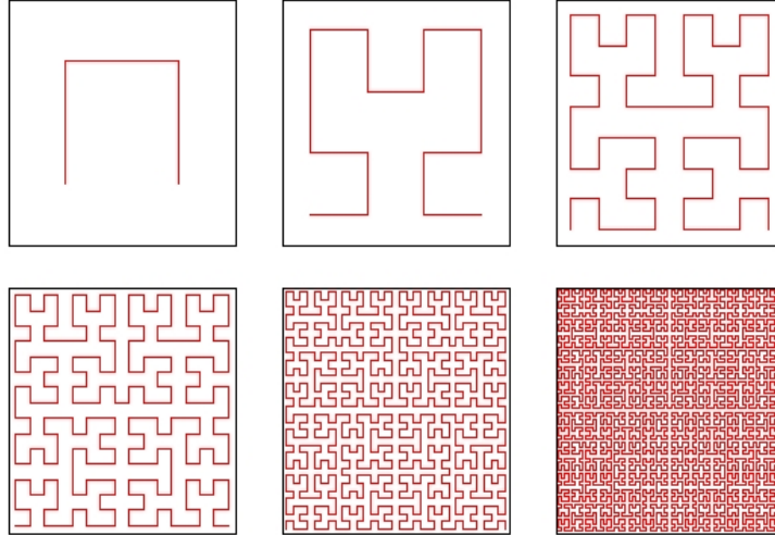
FIGURE 3.1 – Parcours Hilbert-Peano
