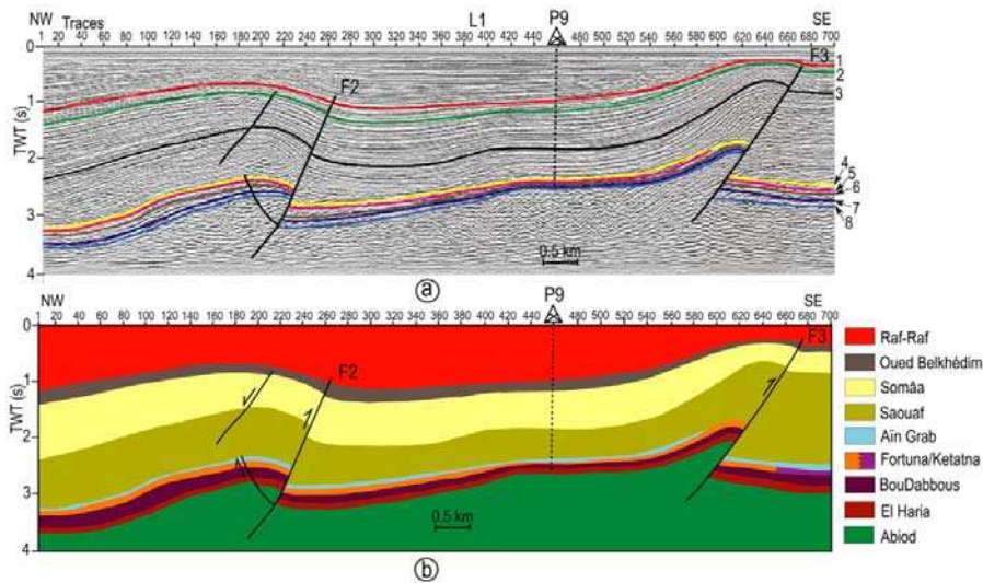
Fig. 5: Ligne sismique L1 de direction NW-SE. (a) Profil sismique montrant les toits des différents horizons: (1) Oued Belkhédim (Messinien), (2) Somâa (Tortonien), (3) Saouaf (Serravalien), (4) Ain Grab (Langhien inférieur), (5) Fortuna (Oligocène), (6) Bou Dabbous (Eocène), (7) El Haria (Paléocène), (8) Abiod (Crétacé), P9: Puits de calage, TWT(s): Temps double en seconde. (b) Coupe géosismique interprétée. Seismic line L1, NW-SE oriented. (a) Seismic line showing the various top of roof: (1) Oued Belkhédim (Messinian), (2) Somâa (Tortonian), (3) Saouaf (Serravalian), (4) Ain Grab (Early Langhian), (5) Fortuna (Oligocene), (6) Bou Dabbous (Eocene), (7) El Haria (Paleocene), (8) Abiod (Cretaceous), P9: Cross-cutting well, TWT(s): Two way time in second. (b) Geoseismic interpreted section.
