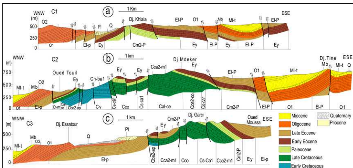
Fig.5.3. Coupes géologiques (C1-C3) dans la région d'Enfidha. Cv: Valenginien, Ch-ba1: Hauterivien-Barrémien supérieur, Cba2-ap: Barrémien supérieur-Aptien, Cal-ce: Albien-Cénomaniens, Cce2-co: Cénomaniens supérieur- Coniacien, Cs-ca1: Santonien- Campanien inférieur, Cco: Coniacien, Ct-m: Turonien- Maastrichtien, Cca2-m1: Campanien supérieur- Maastrichtien inférieur, Cm2-P: Maastrichtien supérieur-Paléocène, Ey: Yprésien, El-p: Lutétien-Priabonien, O1: Oligocène inférieur, O2: Oligocène supérieur, Mb: Burdigalien, MI-t : Langhien-Tortonien, M-Pl: Mio-pliocène, Q: Quaternaire.
