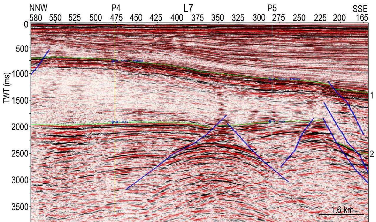
Fig.7.19. Profil sismique L7 de direction NNW-SSE montrant l'inversion des bassins dans le golfe de Hammamet. 1: horizon Aïn Grab, 2: Horizon Oued Belkhédim.
