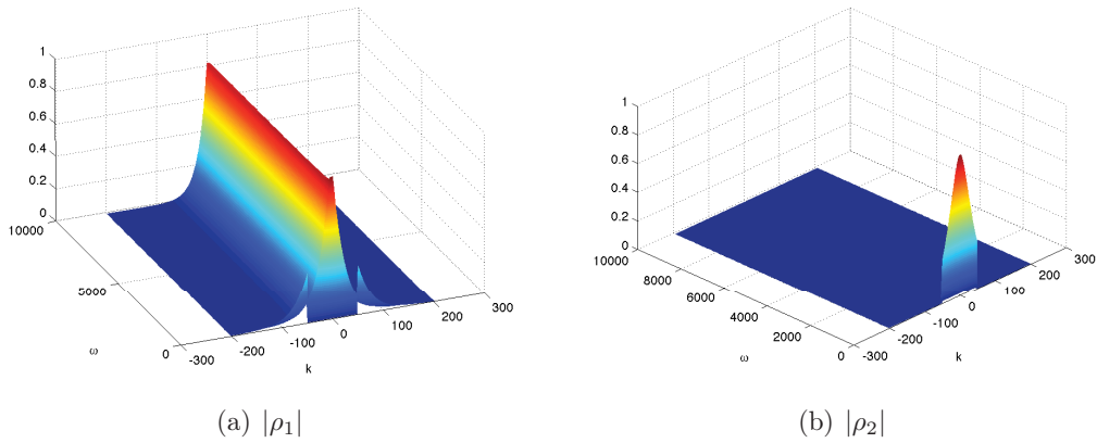
FIGURE 9.1 – Valeurs propres de la matrice d’amplification des erreurs pour le système (9.9). Les graphes ont été tracés avec les valeurs numériques suivantes : Re = 10^3 , \Delta t = 10^{-4} , \Delta z = 1/64 et deux mailles de recouvrement ( L = 2\Delta x ).
