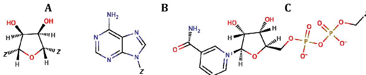
Figure 6 - Structure chimique des 3 fragments les plus présents dans la base de données. A : le (3R,4S)-oxolane-3,4-diol (n=1375) ; B : l'adénine (n=1112); C : Nicotinamide β-D-ribose diphosphate (n=342).
