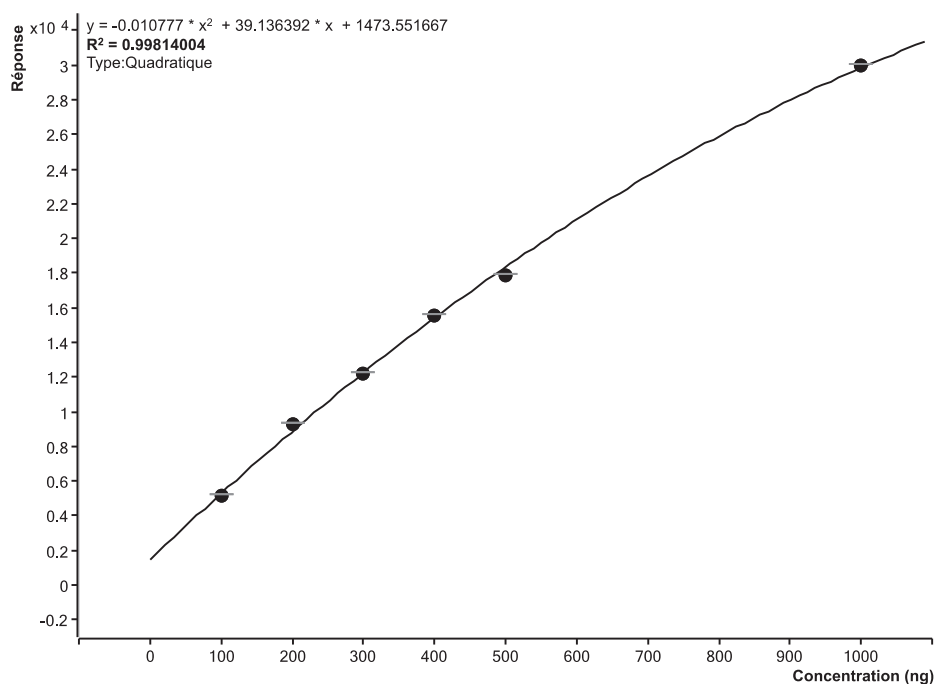
Figure III:33: Courbe de calibration du vandatéroside II ( R^2=0,99814 ).
