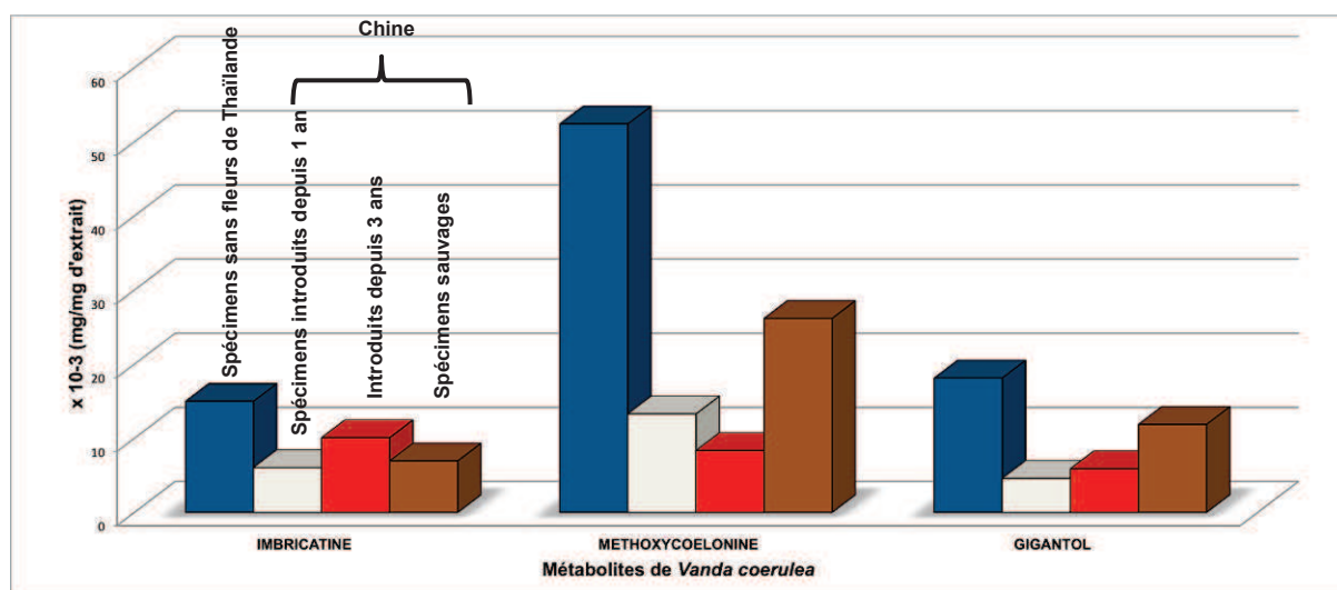
Figure III:41: Les teneurs des marqueurs dans les échantillons de Vanda coerulea prélevés dans leur milieu sauvage en Chine comparées aux spécimens sans fleurs de Thaïlande.
