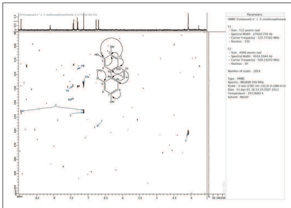
Figure II:31. Spectre RMN bidimensionnel 1 H/ 13 C HMBC de l'aérosanthrène (500 MHz, CD 3 ODCD 3 ).
