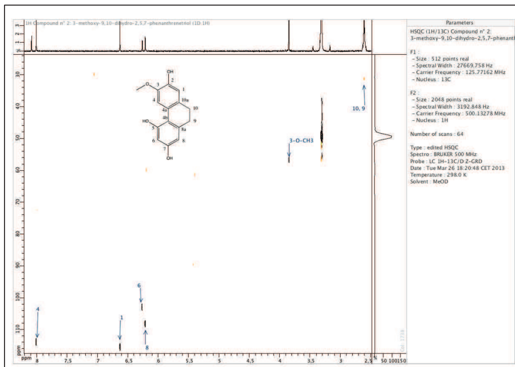
Figure II:32. Spectre RMN bidimensionnel ^1\text{H}/^{13}\text{C} HSQC de l'aërosine (500 MHz, \text{CD}_3\text{ODCD}_3 ).
