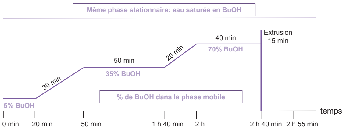
Figure III:4: Représentation schématique du gradient d'éluant utilisé pour fractionner l'extrait standard de Vanda teres 1801-07/612. La même phase stationnaire est maintenue tout au long de l'éluant, la composition de la phase mobile varie en fonction du temps. L'extrusion est réalisée après 2h40 d'éluant.
