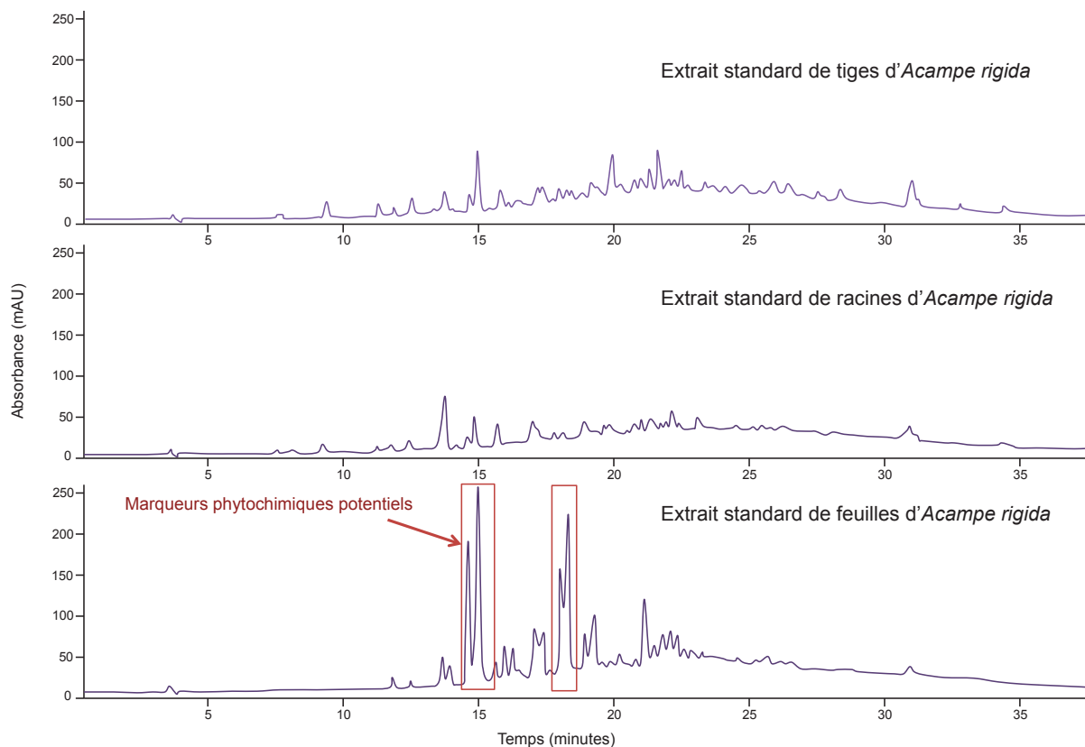
Figure II:37: Comparaison des profils chromatographiques des tiges, feuilles et racines d' Acampe rigida . Les composés encadrés en rouge ont été repérés comme marqueurs phytochimiques potentiels des feuilles d' A. rigida . Phase stationnaire : Nucleodur C18 250 x 4,6 mm i.d. 5 \mu m. Phase mobile eau+0,1%A.F. (A) et MeOH +0,1% A.F. (B) Gradient d'éluion (temps : %B) : 0 min, 2% ; 30-35 min, 100%. Détection à 60 nm.
