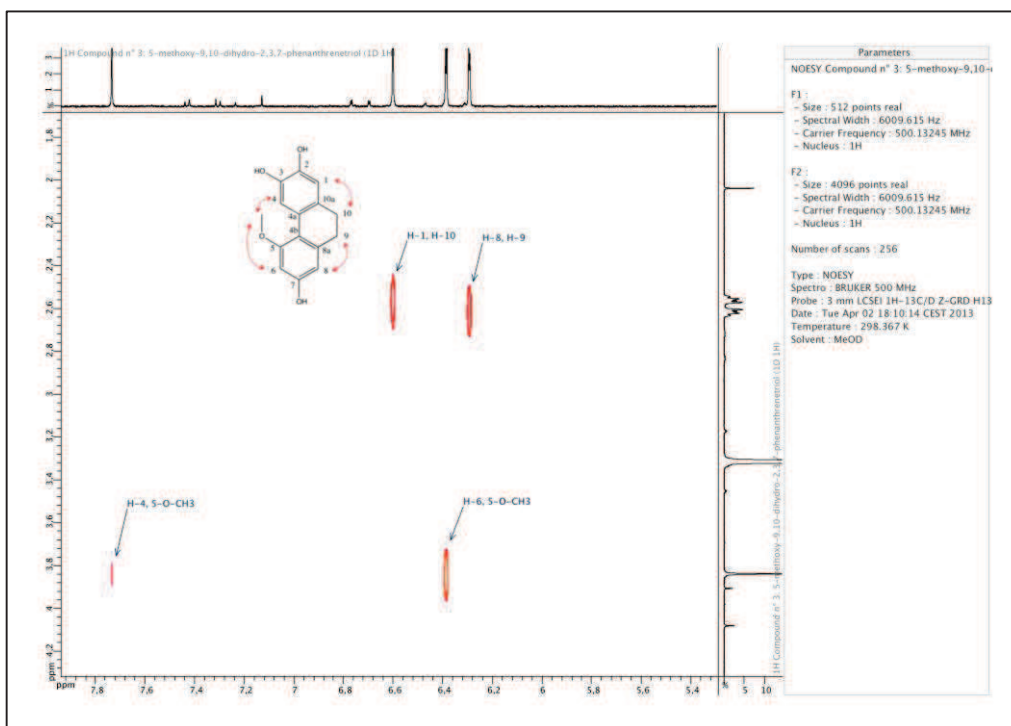
Figure II:24. Spectres RMN bidimensionnel 1 H/ 1 H NOESY du 5-méthoxy-9,10-dihydro-2,3,7-phénanthrènetriol (3) (500 MHz, CD 3 OD).
