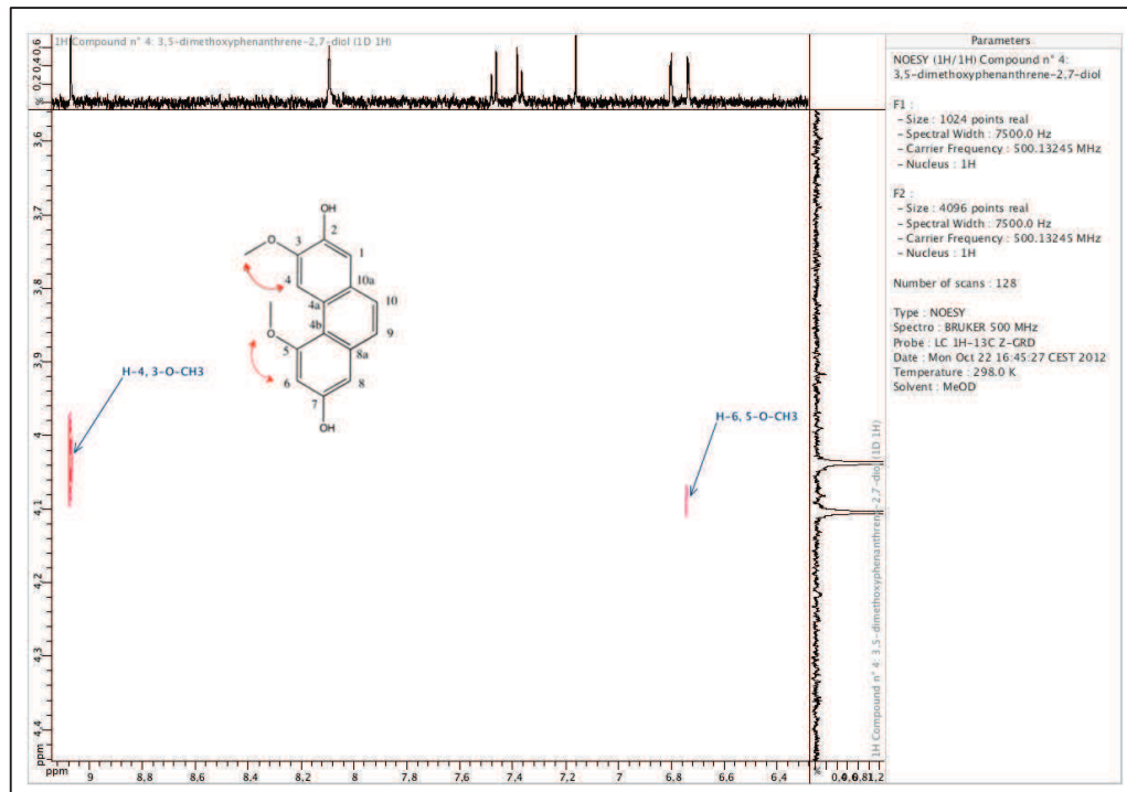
Figure II:25. Spectres RMN bidimensionnel 1 H/ 1 H NOESY du 3,5-diméthoxyphénanthrène-2,7-diol (4) (500 MHz, CD 3 OD).
