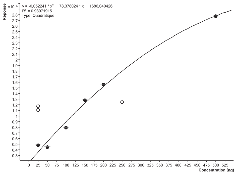
Figure III:28: Courbe de calibration de la flavindine ( R^2=0,98972 ).
