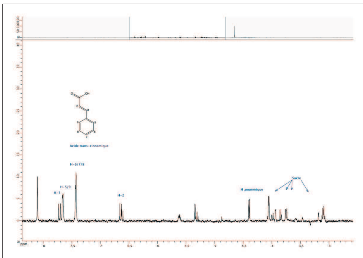
Figure II:56: Spectre ^1\text{H} du composé C ( \text{CD}_3\text{CN} , 500 MHz).
