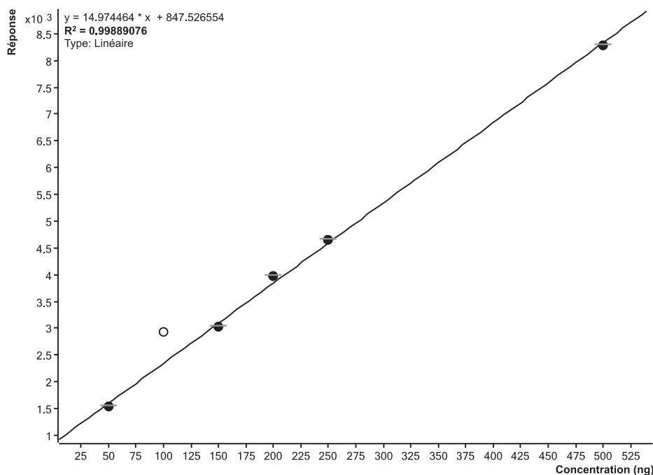
Figure III:34: Courbe de calibration du vandatéroside III ( R^2=0,99889 ).
