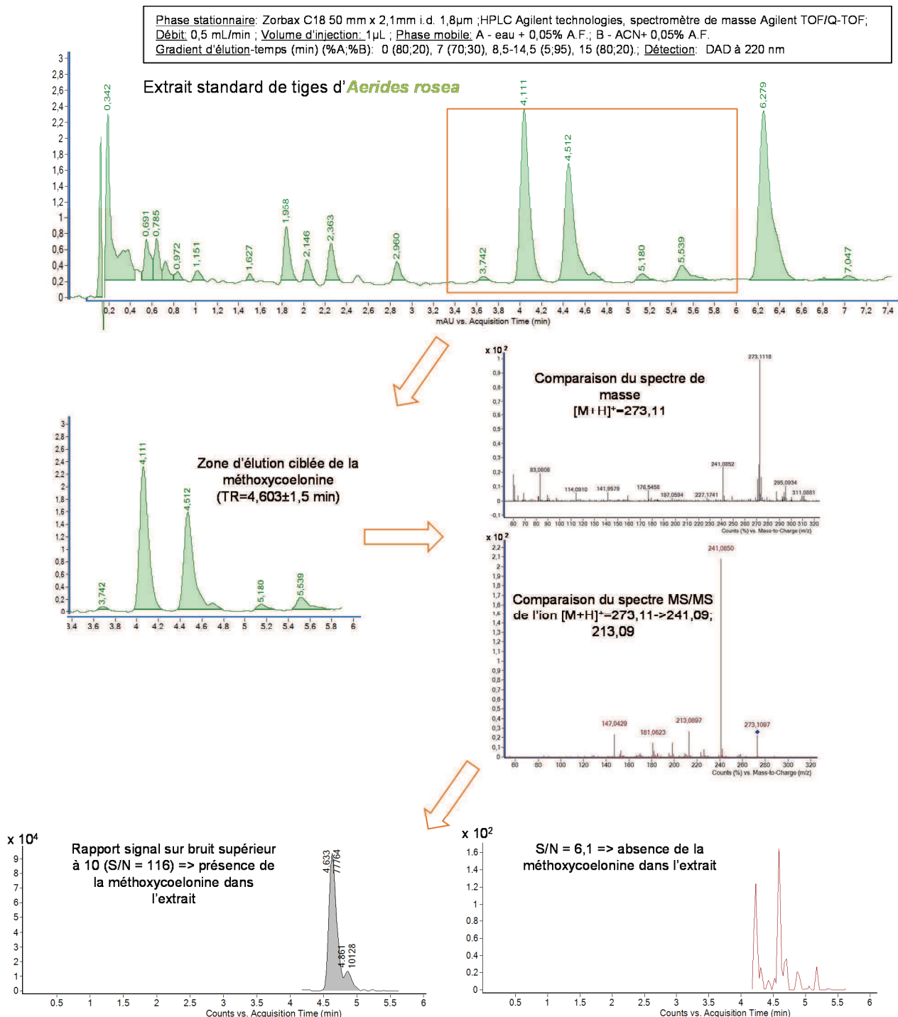
Figure II.2. Schéma de la méthode de déréplication développée en illustrant l'exemple de la méthoxycoelonine.
