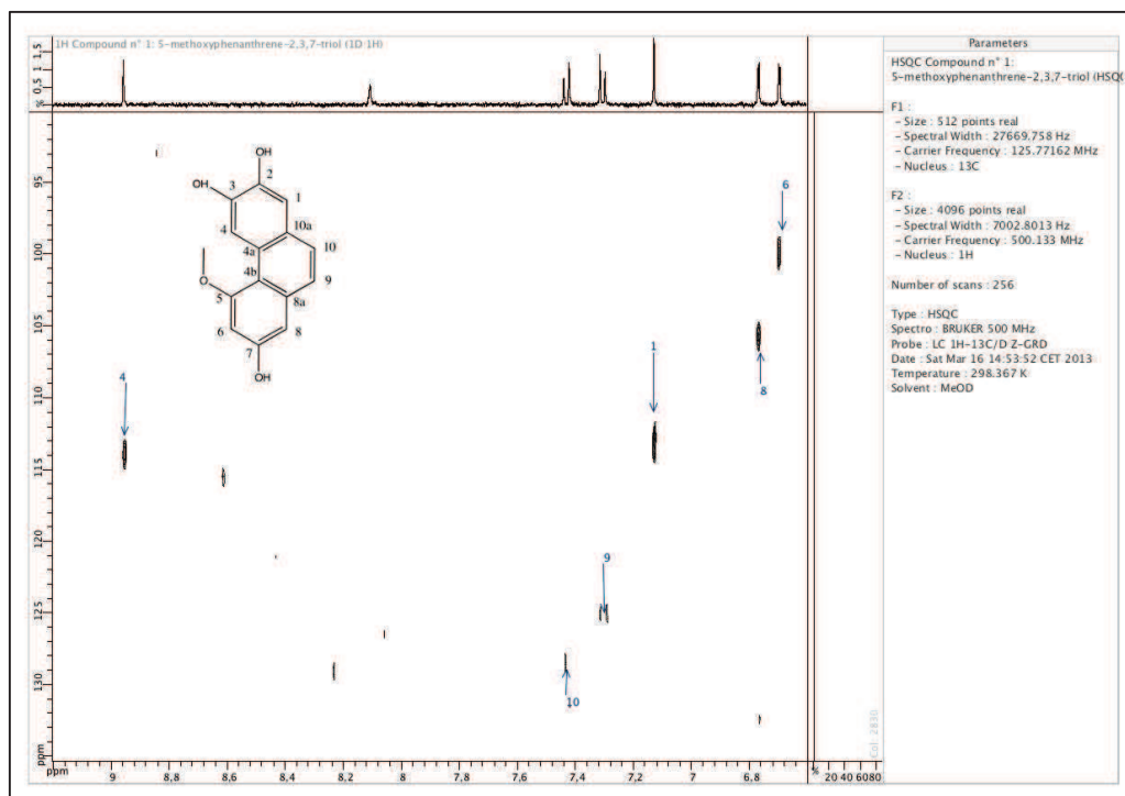
Figure II:30. Spectre RMN bidimensionnel 1 H/ 13 C HSQC de l'aérosanthrène (500 MHz, CD 3 ODCD 3 ).
