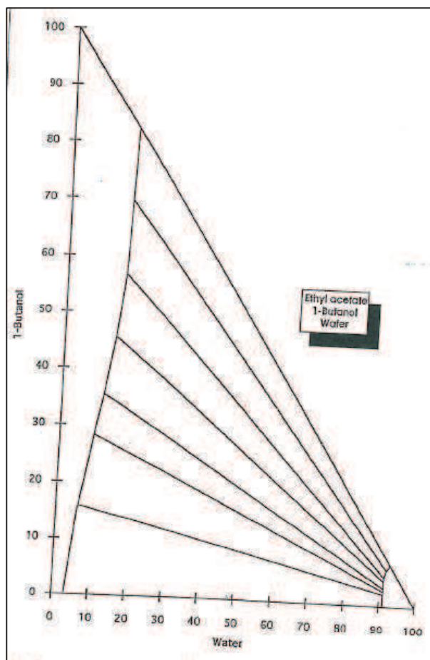
Figure III:3. Diagramme ternaire du système biphasique constitué d'acétate d'éthyle-1-butanol-eau (document fourni par Armen instrument).
