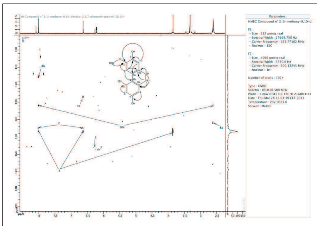
Figure II:33. Spectre RMN bidimensionnel ^1\text{H}/^{13}\text{C} HMBC de l'aërosine (500 MHz, \text{CD}_3\text{ODCD}_3 ).
