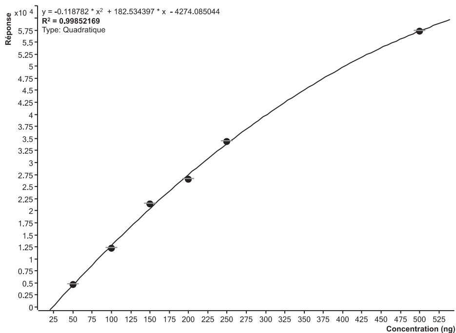
Figure III:32: Courbe de calibration du vandatéroside I ( R^2=0,99852 ).
