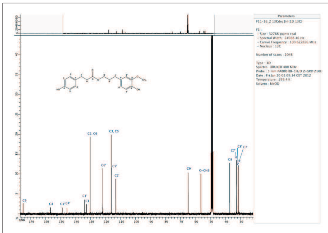
Figure II:13. Spectre RMN monodimensionnel ^{13}\text{C} de l'acide dihydroconiféryll dihydro- p -coumarique (400 MHz, \text{CD}_3\text{OD} ).
