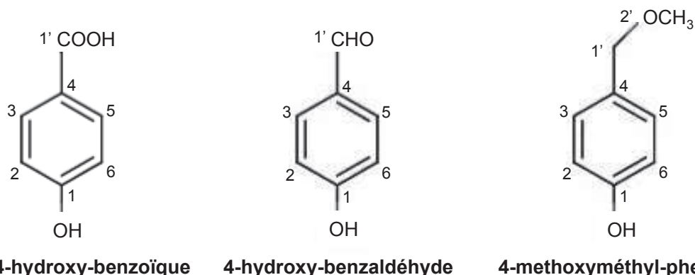
Figure II:48: Structures et numérotation des atomes de carbone des trois métabolites des feuilles d' Acampe rigida .
