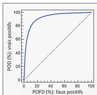
Figure 84 – Courbe de ROC tracée à partir des valeurs de POD en fonction du POFD pour plusieurs seuils.
