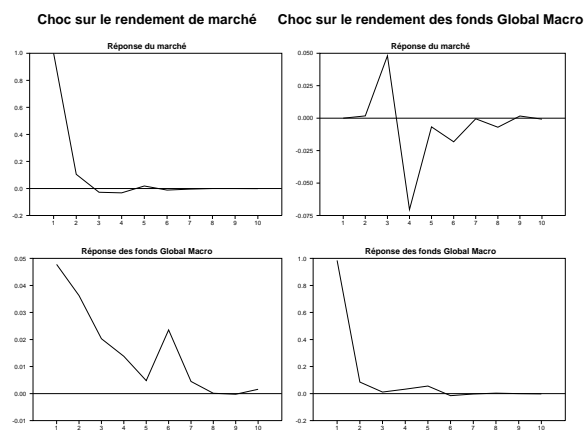
Figure 1.2 – Fonctions de réponse impulsionnelle - VAR R^{la} - R^{hf}
