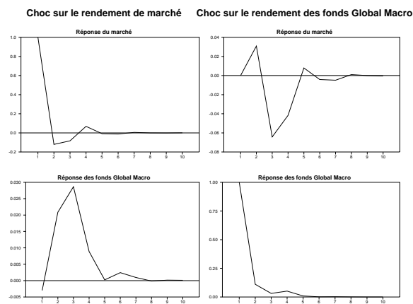
Figure 1.1 – Fonctions de réponse impulsionnelle - VAR R^{us} - R^{hf}
