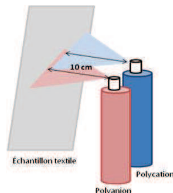
Figure 13 Technique de nébulisation de polyélectrolytes sur un substrat plan vertical 168
