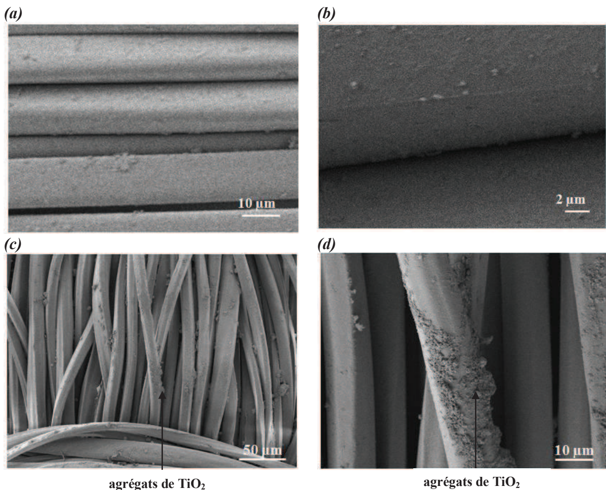
Figure 104 Images MEB du textile polyester sans prétraitement à KOH et non fonctionnalisé (nu), échelle de 10 µm (a) et de 2 µm (b).
