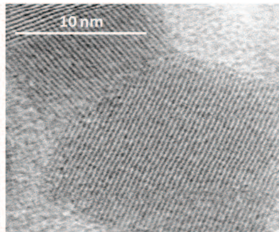
Figure 22 Cliché HRTEM du TiO 2 P25
