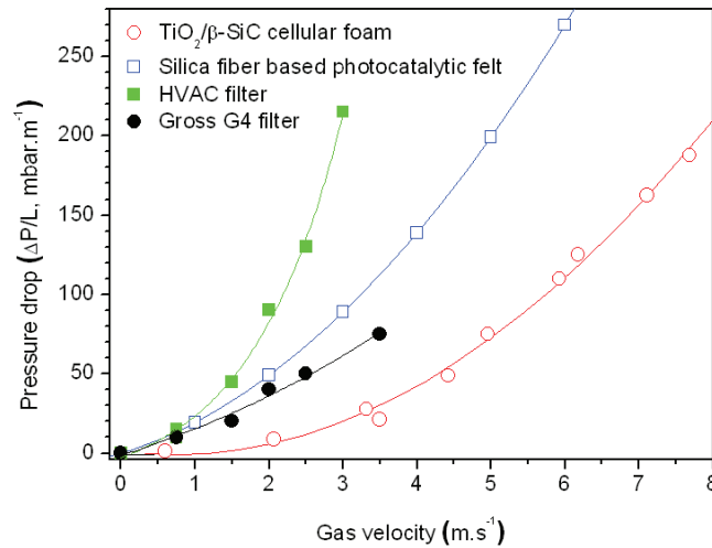
Figure 89 Comparaison des pertes de charge en fonction de la vitesse de passage de l'air pour une mousse alvéolaire de taille moyenne d'alvéole 5400 \mu\text{m} , le média photocatalytique Quartzel® et des filtres de type G4 et HVAC. Remarque : les données des filtres G4 et HVAC sont des données « Saint-Gobain ». Celles du média Quartzel®, fournies par Saint-Gobain, ont été vérifiées à l'ICPEES.
