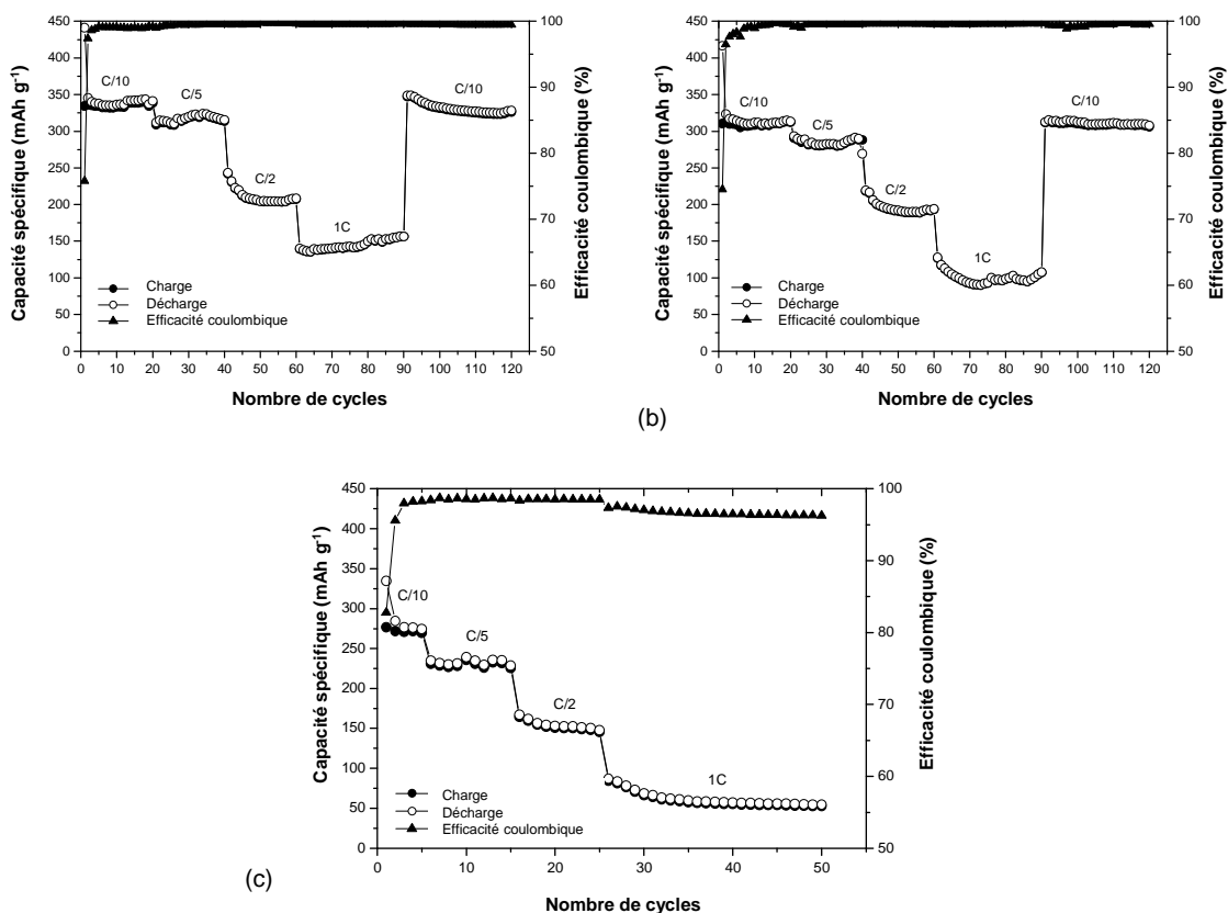
Figure I. 9 Tests de cyclage décharge/charge à température ambiante à différents régimes de courants constants. (a) Anode papier 90%GP/10%FB avec CMC, (b) anode papier 90%GP/10%FB sans CMC et (c) anode de référence 90%GP/10%PVdF.
