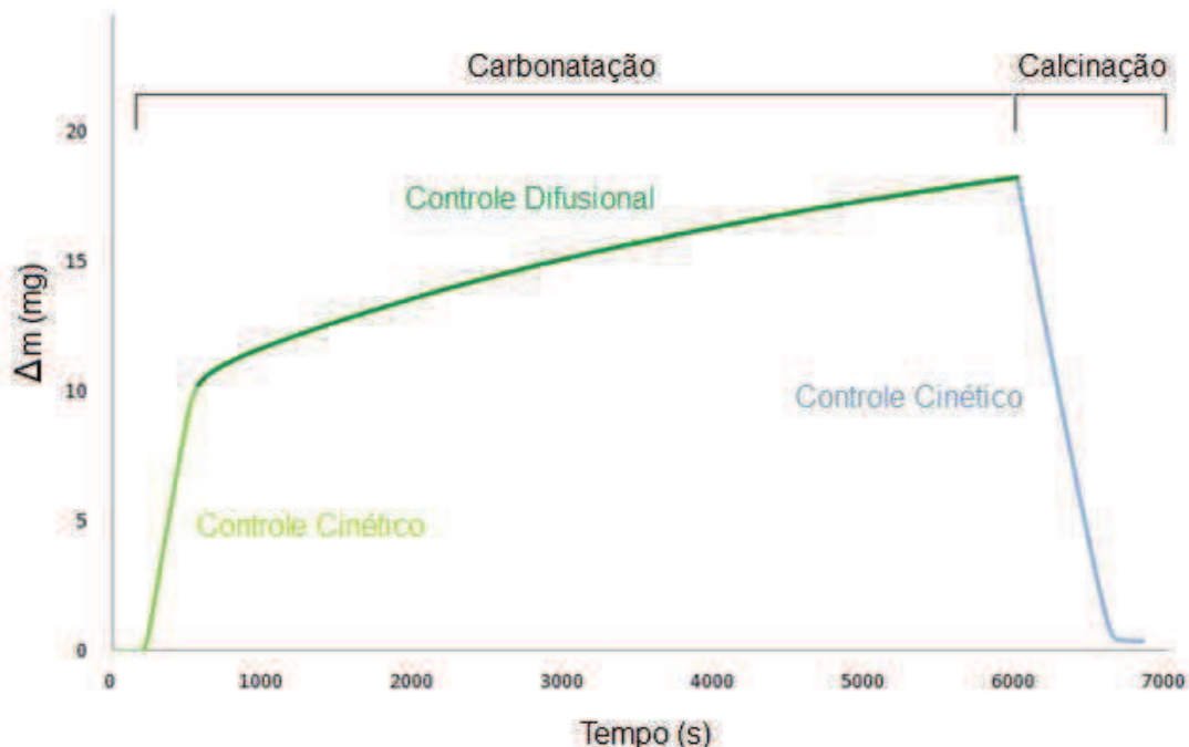
Figure 3 - Aperçu des différents mécanismes de contrôle dans un cycle complet de carbonatation- décarbonatation de CaO (adapté de la référence 9).
