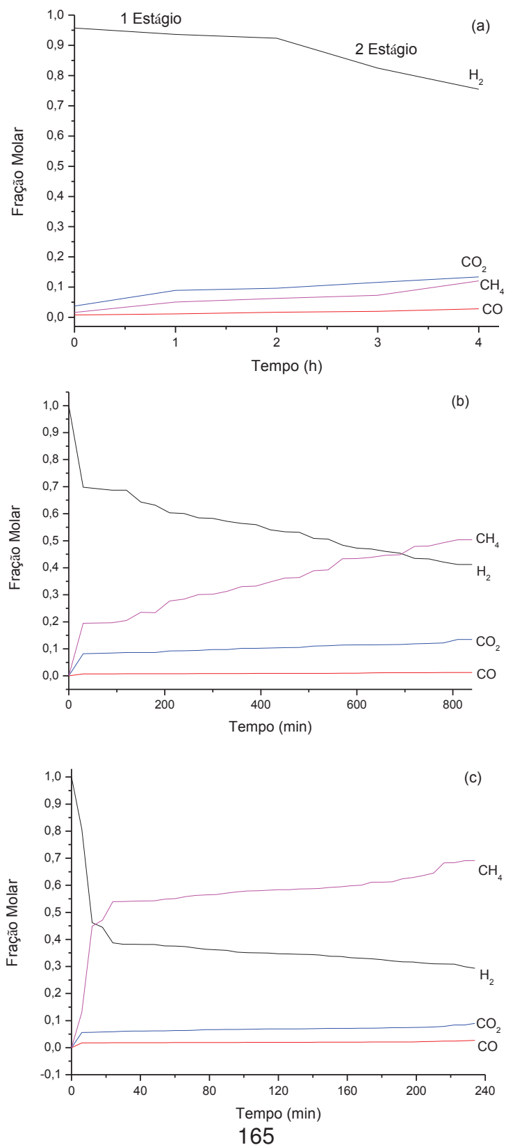
Figura 4.49 - Testes de reforma a vapor do metano otimizada por absorção de CO 2 do catalisador I-Ni-CA75L em função do tempo: (a) primeira etapa bis, (b) segunda etapa após o 1° ciclo de carbonatação-calцинаção e (c) terceira etapa após o 2° ciclo de carbonatação-calцинаção. Condições de Reação (CR3): Taxa de fluxo (Ar = 26 mL min -1 , CH 4 = 1,0 mL min -1 , H 2 O = 3,0 mL min -1 ); massa do catalisador = 1,0 g, razão molar H 2 O/CH 4 = 3; temperatura = 650 °C.
