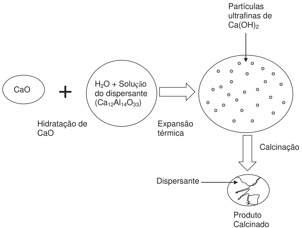
Figura 2.12 - Diagrama esquemático de preparação do absorbente.
