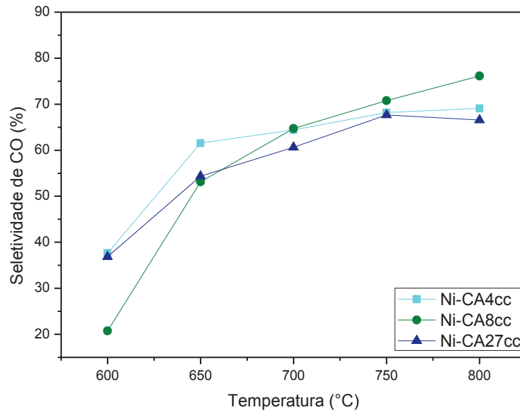
Figura 4.9 – Seletividade em CO como função da temperatura de reação.
