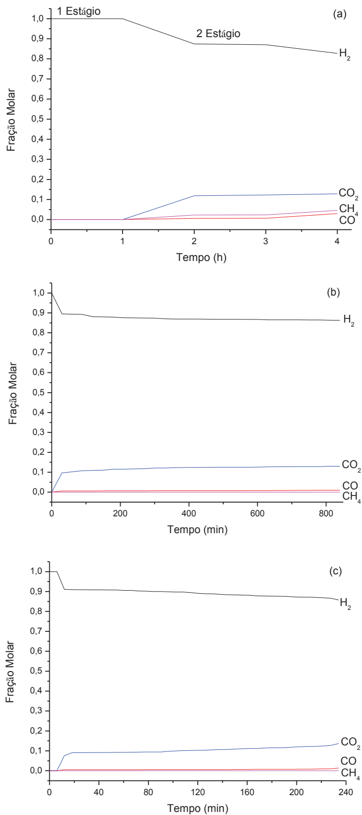
Figura 4.28 - Testes de reforma a vapor do metano otimizada por absorção de CO 2 do catalisador M-Ni10-CA75M em função do tempo: (a) primeira etapa bis, (b) segunda etapa após o 1° ciclo de carbonatação-calcinação e (c) terceira etapa após o 2° ciclo de carbonatação-calcinação. Condições de Reação (CR3).
