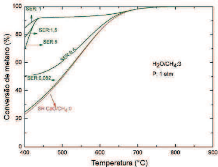
Figura 2.10 - Efeito da temperatura e da razão molar absorvente/metano sobre o equilíbrio de conversão de metano no caso de reforma a vapor (do inglês steam reforming – SR) e reforma a vapor otimizada por absorção (sorption enhanced steam reforming – SER). Razão molar H_2O/CH_4 = 3 em 1,0 atm.
