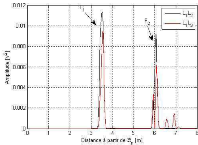
Figure IV.29 – Détection des deux défauts inductifs, localisés à 3.5m et 6m du point d'injection \mathfrak{S}_p dans la branche L_2 et L_3 respectivement.
