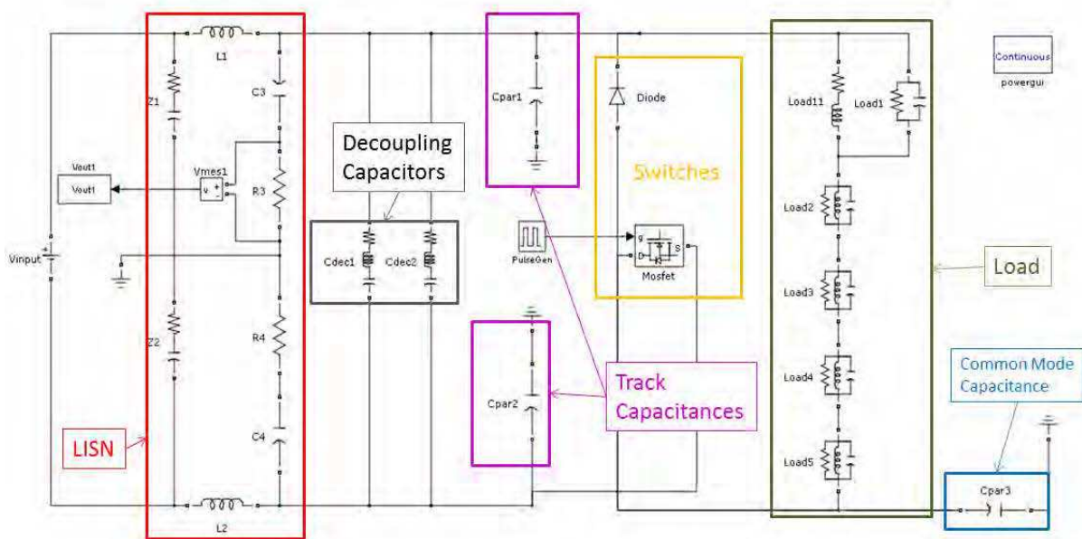
Figura 5 - 11 – Diagrama esquemático preciso de um conversor buck.
