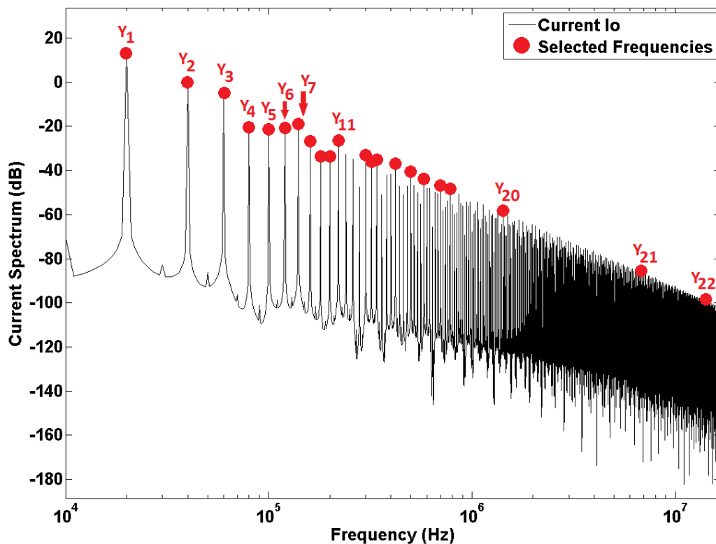
Figura 5 - 3 – Corrente de saída I_o vs. Frequência. Frequências selecionada marcadas em vermelho (Redução da saída).
