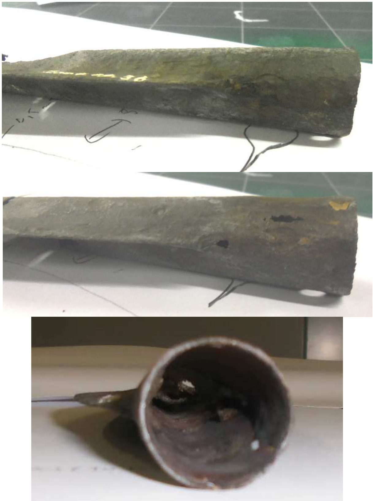
Fig. 172 : Douille.
