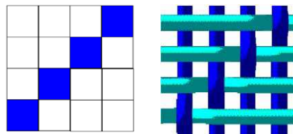
Figure 19. La mise en forme du Sergé
