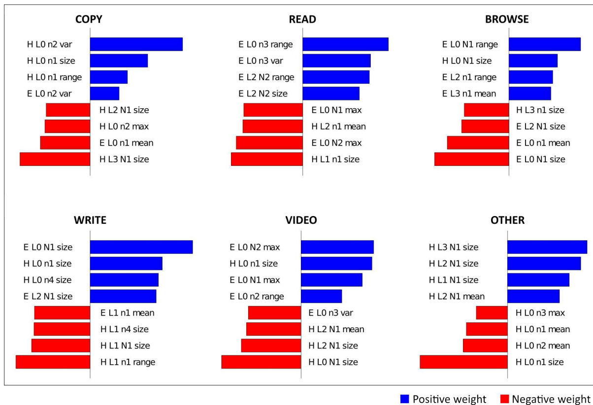
Figure 5.13 – Contribution relative des poids dominants positifs (en bleu) et négatifs (en rouge) pour chaque classe. Une description de chaque caractéristique est donnée dans le tableau 5.5.
