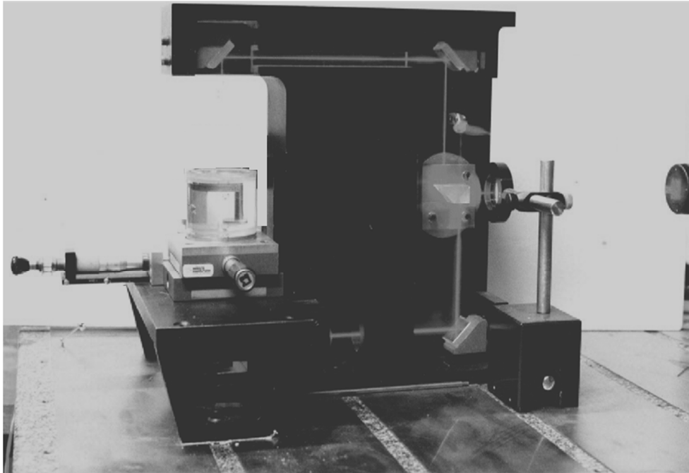
Figure II.9 : Montage interférométrique.
