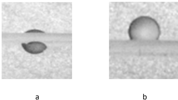
Figure P.2 : Bille de polystyrène (de type PS6) en équilibre à l'interface : a) avant rupture du film : équilibre dynamique b) après rupture du film : équilibre statique.
