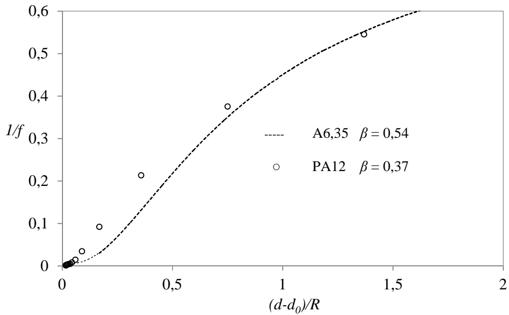
Figure IV.24 : Variations de l'inverse du coefficient de frottement 1/f en fonction de l'écart à la position d'équilibre (d - d_0)/R : effet de \beta . Bo_p \cong 1,55 et \lambda \cong 0 .
