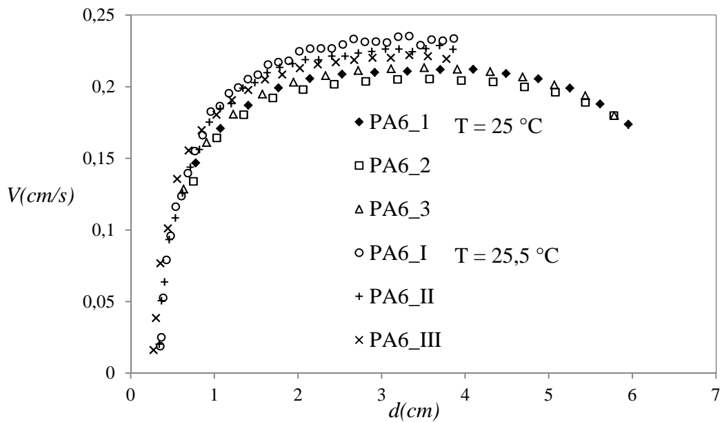
Figure A1.2 : Billes de type PA6, \lambda = 0,01 .
