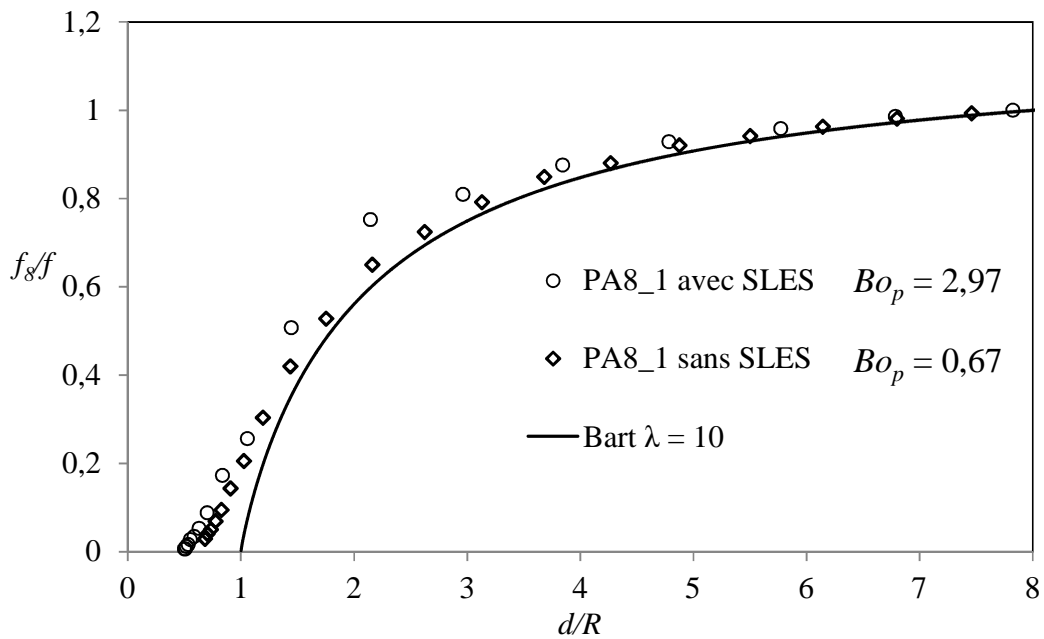
Figure IV.16 : Variations de l'inverse du coefficient de frottement réduit en fonction de la distance réduite – influence de Bo_p : points expérimentaux associés à la bille PA8 avec et sans SLES (resp. \beta = 0,37 et \beta = 0,45 ) et courbe théorique de Bart ( \lambda = 10 ).
