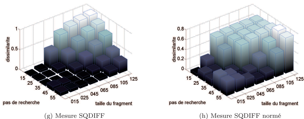
FIG. 4.9 – Erreur de similarité pour chacune des mesures.
