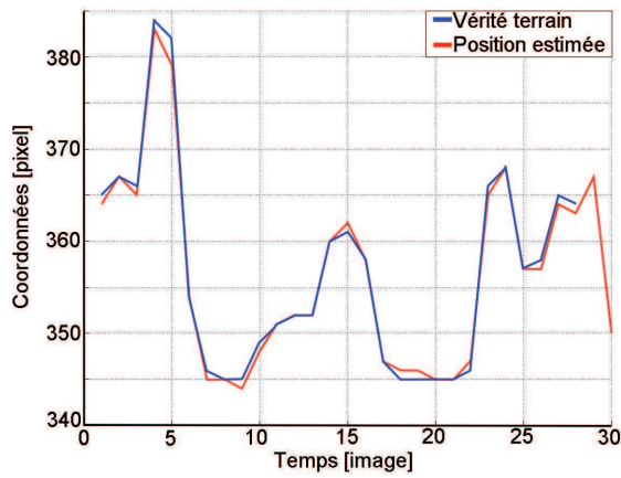
(a) Ecart entre position réelle et position estimée suivant l'axe des x.
