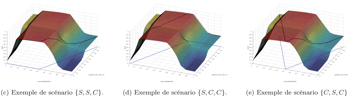
FIG. 3.6 – Mise en évidence de la variabilité de l'intérêt de la classe sang selon le temps opératoire et la situation opératoire.
