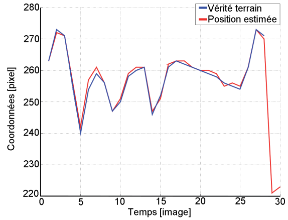
(b) Ecart entre position réelle et position estimée suivant l'axe des y.
