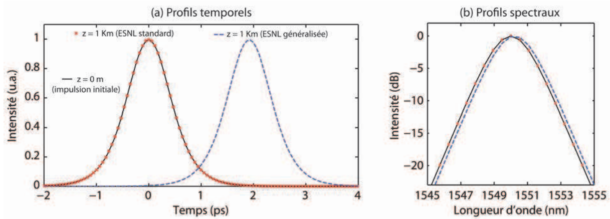
FIGURE 1.12 – Profil temporel (a) et spectral (b) initial d'un soliton fondamental (ligne noire) comparé aux profils obtenus après 1 km de propagation en considérant une intégration de l'ESNL standard (croix rouges) et de l'ESNL généralisée (ligne bleue pointillée).
