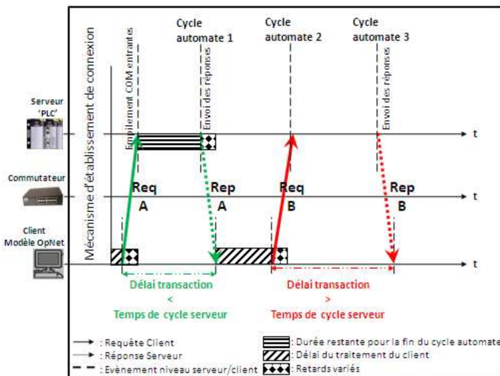
Figure 7.6 Mécanisme des échanges de communication entre les constituants de l'architecture Co-Simulées S_cR_rR_s
