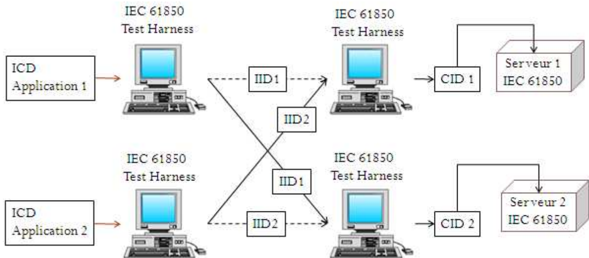
Figure 8.1 Configuration des applications IEC 61850 en passant par les fichiers IID
