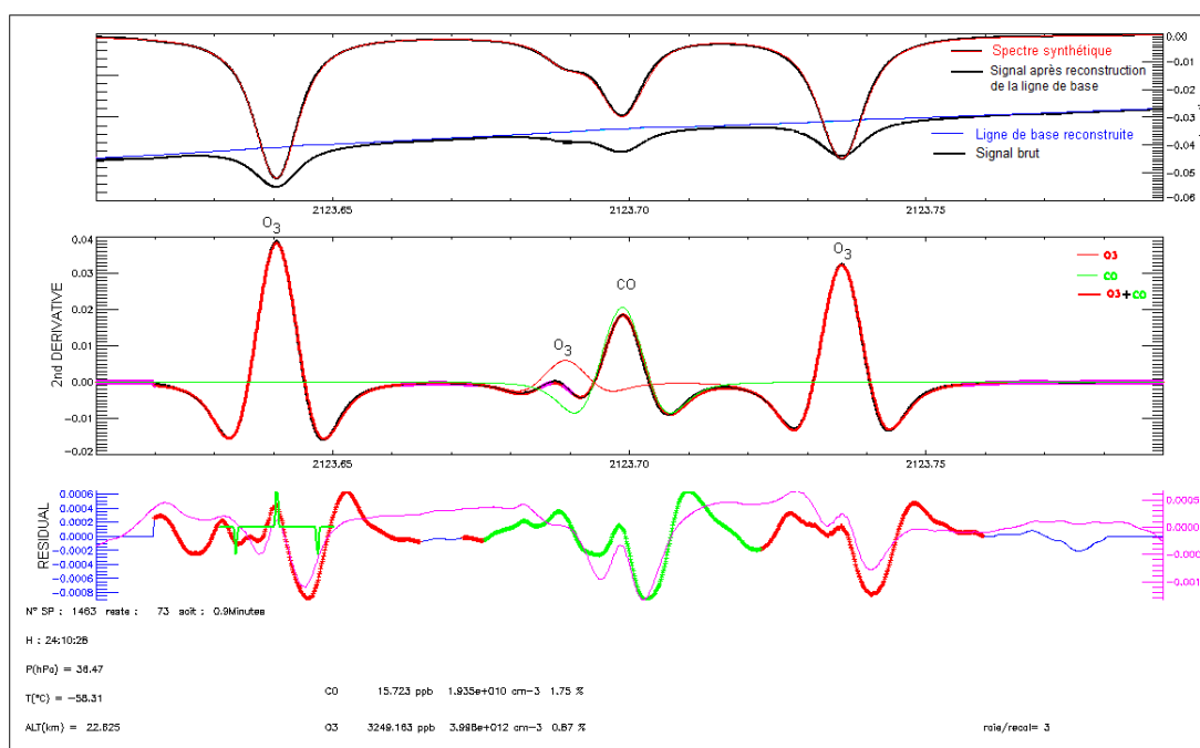
Figure 2-4 : Procédure d'extraction des données pour \text{CO} et \text{O}_3 entre 2123,61 \text{ cm}^{-1} et 2123,80 \text{ cm}^{-1} . Exemple pour SPIRALE à 22,8 km en 2008. En haut : spectres expérimental (« signal » en noir,) et simulé (« synthétique » en rouge) ; au milieu : Ajustement des dérivées secondes des spectres expérimental et simulé ; en bas : résidu de l'ajustement des dérivées secondes à une échelle environ 50 fois plus faible.
