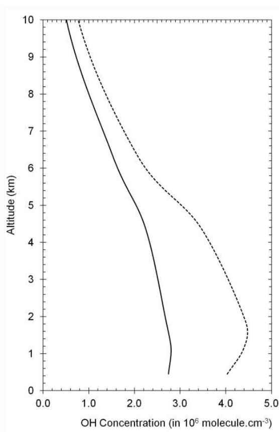
Figure 5-6 : Profils verticaux d'OH en molécules.cm -3 moyennés pour une simulation de 10 jours dans un milieu propre (ligne pleine) et dans un milieu pollué (ligne pointillées)
