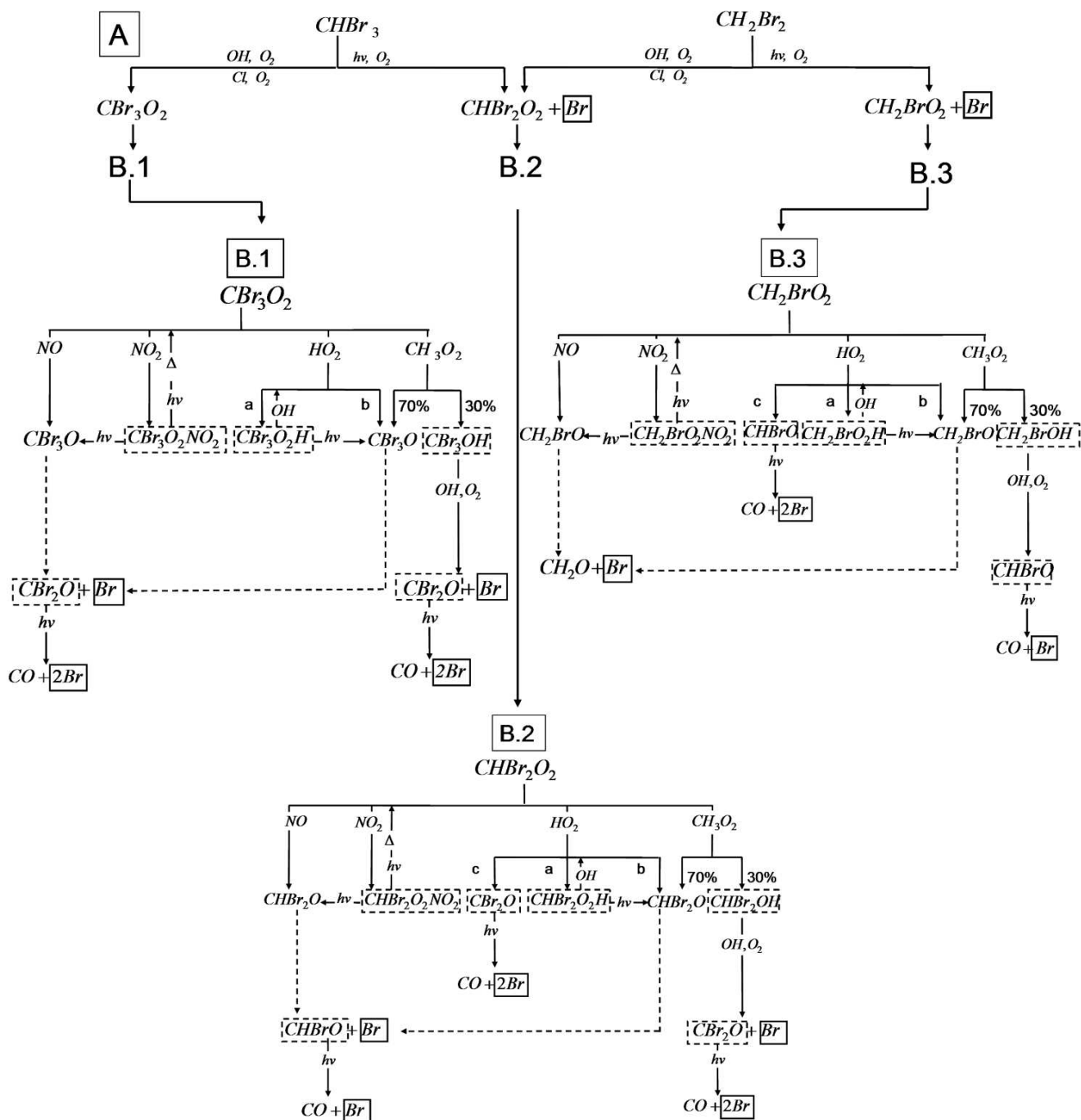
Figure 5-2: Schéma chimique de dégradation du bromoforme ( \text{CHBr}_3 ) et du dibromométhane ( \text{CH}_2\text{Br}_2 ). A : étape initiale (réaction avec OH, Cl et photolyse), B : réaction des intermédiaires peroxydes bromés, B.1 : \text{CBBr}_3\text{O}_2 , B.2 : \text{CHBr}_2\text{O}_2 (communs à \text{CHBr}_3 et \text{CH}_2\text{Br}_2 ) et B.3 : \text{CH}_2\text{BrO}_2 . Les intermédiaire stables sont encadrés en pointillés et les produits inorganiques finaux sont encadrés en ligne pleine. Les réactions de décompositions sont indiquées par des lignes pointillées.
