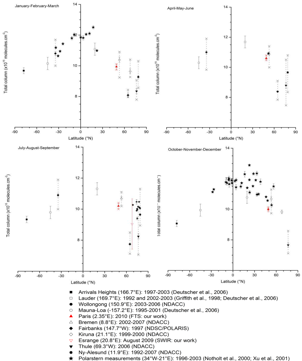
Figure 4-4: Moyennes pondérées par l'erreur de la colonne totale d'OCS avec les barres d'erreur (1 écart-type \sigma ) en fonction de la latitude (°N) pour différentes stations NDACC et pour Paris (STF du LPMAA) mesurées par FTIR. Le minimum et le maximum de chaque série sont représentés par des croix et une ligne en pointillée. En plus, les colonnes totales d'OCS avec les barres d'erreurs ( 1\sigma ) provenant : (1) des campagnes du Polarstern mesurées par l'interféromètre Bruker1 20M (Notholt et al., 2000 ; Xu et al., 2001), (2) de la campagne NDSC/POLARIS mesurée par l'interféromètre MkIV (Toon et al., 1991) et (3) de la campagne ballons StraPolEté mesurée par l'instrument SWIR-balloon.
