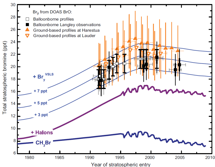
Figure 1-9 : Rapport de mélange du brome total inorganique Br_y (en pptv) dérivant d'observations par mesures ballons (carré noir ; Dorf et al., 2006) et à partir du sol au-dessus de Harestua ( 60^\circ N ) et Lauder ( 45^\circ S ) (triangle orange ; Hendrick et al., 2008). Le Br_y de la stratosphère est comparé aux mesures troposphériques de CH_3Br (ligne bleu en gras) et de CH_3Br + des Halons (ligne violette en gras) (Butler et al., 1999 ; Fraser et al., 1999). (source : Montzka et Reimann, WMO 2011).
