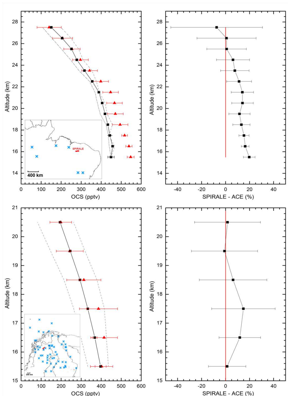
Figure 4-9: A gauche: Rapport de mélange (pptv) d'OCS mesuré par SPIRALE avec les barres d'erreurs (triangle rouge) comparé à la moyenne (pondérée par l'erreur) des profils mesurés par ACE-FTS avec les barres d'erreurs (erreur pondérée). Les profils en pointillés gris représentent le minimum et le maximum dans les profils d'ACE-FTS. A droite : Pourcentage de différence entre SPIRALE et ACE-FTS. Les figures du haut sont pour le vol de SPIRALE du 9 juin 2008 à Teresina et les figures du bas pour le vol du 24 août 2009 à Kiruna. Une carte, montrant les latitudes et longitudes des profils d'ACE-FTS utilisés, est indiquée.
