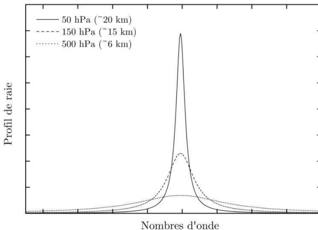
Figure 2-1: Profils de Voigt pour des raies d'intensités intégrées équivalentes pour des pressions et températures correspondant à 3 altitudes différentes : 50 hPa ( \sim 20 km) et 220 K (ligne pleine), 150 hPa ( \sim 15 km) et 215 K (ligne en tirets) et 500 hPa ( \sim 6 km) et 260 K (ligne en pointillées).
