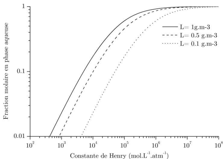
Figure 5-1: Fraction molaire en phase aqueuse en fonction de la constante de Henry à 298K pour 3 teneurs en eau du nuage : 1 \text{ g.m}^{-3} (ligne pleine), 0,5 \text{ g.m}^{-3} (ligne en tirets) et 0,1 \text{ g.m}^{-3} (ligne pointillée) (Reproduction de la figure de Seinfeld et Pandis (2006))
