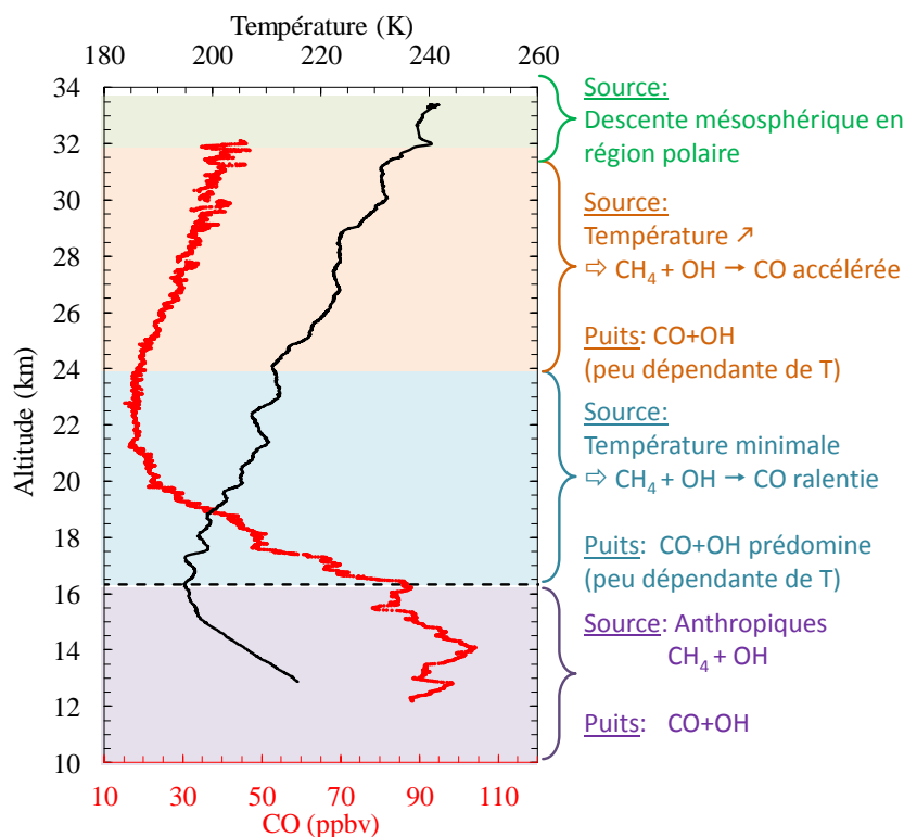
Figure 3-5 : Profils verticaux de CO et de la température au-dessus de Teresina au Brésil (5°S) en juin 2005 mesurés par SPIRALE. La prédominance des sources et puits de CO est résumée selon l'altitude.
