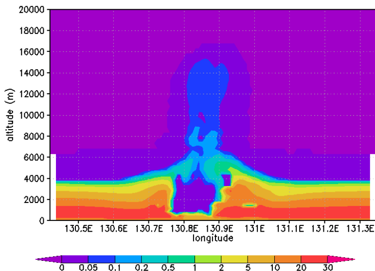
Figure 5-16 : Rapport de mélange de Br contenu dans HBr à 12,4^{\circ}\text{S} à t_0+30 min pour la simulation PERT (Marécal et al., 2012).
