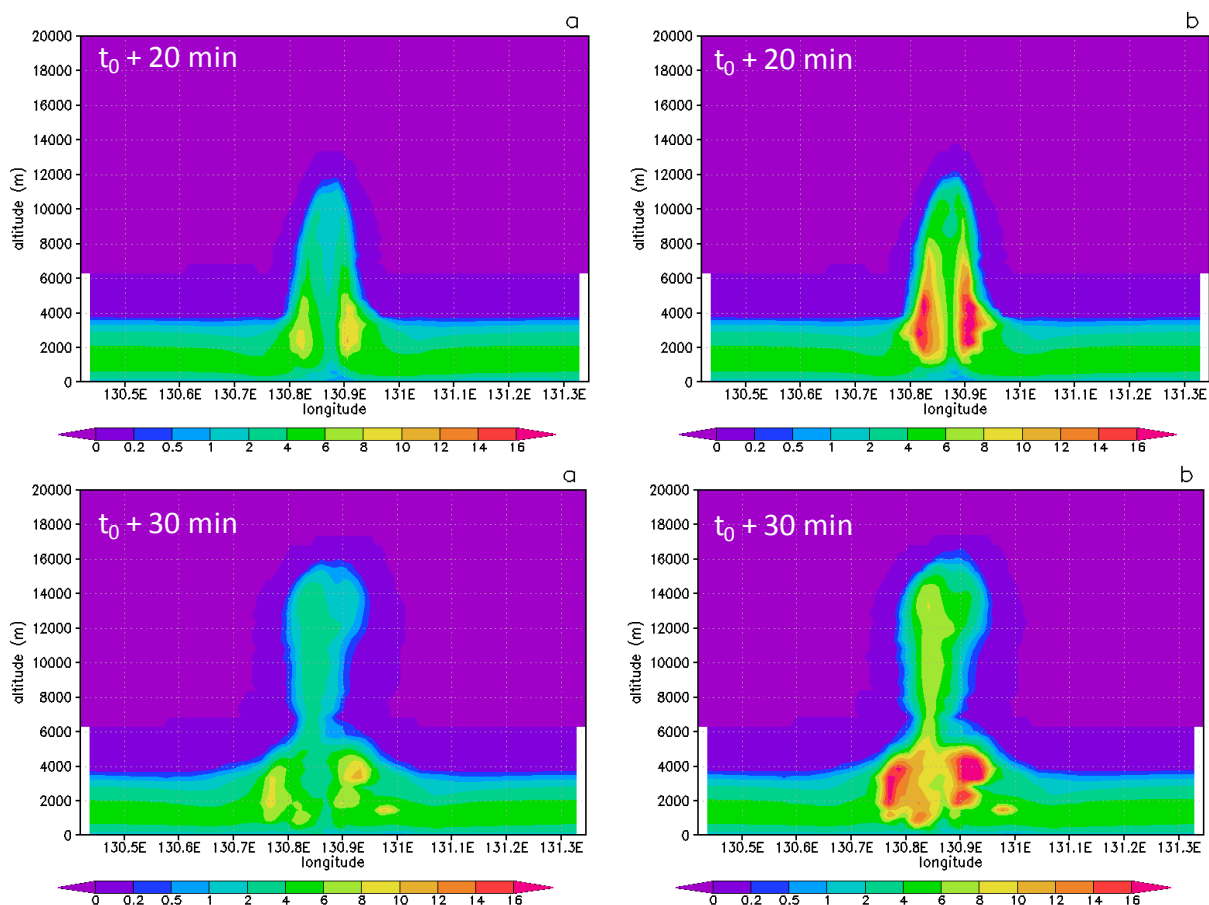
Figure 5-17 : Rapport de mélange de Br contenu dans \text{Br}_x ( \text{Br} + \text{BrO} + \text{HOBr} + 2 \times \text{Br}_2 ) à 12,4^\circ\text{S} à t_0+20 min (figures du haut) et t_0+30 min (figures du bas) pour la simulation PERT à \text{pH}=4 (a) et \text{pH}=5 (b) (Marécal et al., 2012).
