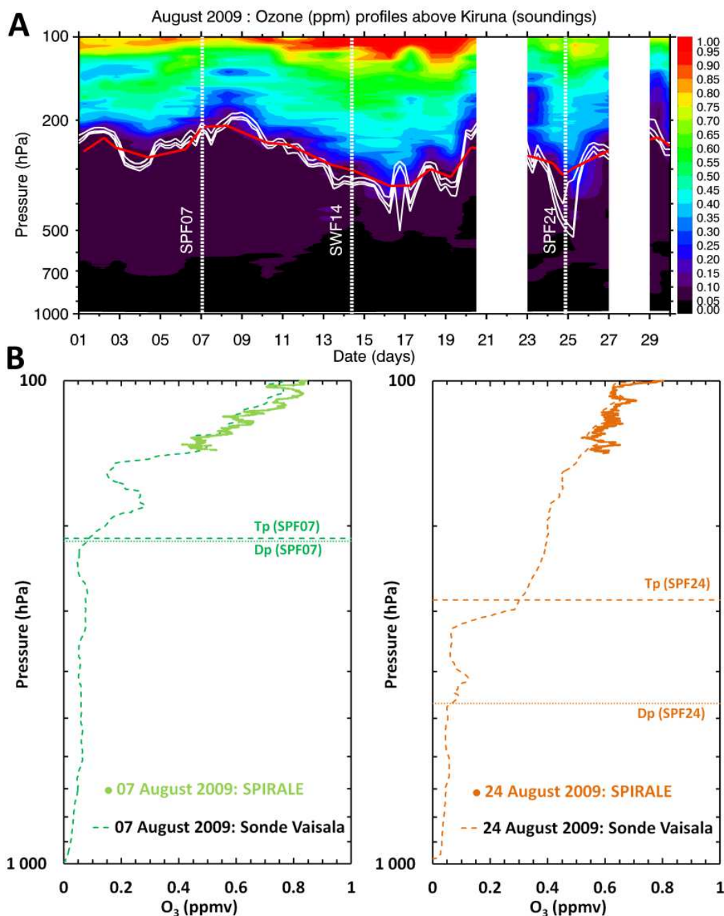
Figure 3-15 : A : Profils verticaux du rapport de mélange de l'ozone en ppmv au-dessus de Kiruna à partir de radiosondages (Vaisala Radiosonde RS92) pendant août 2009. Les vols de SPIRALÉ des 7 et 24 août 2009 et de SWIR le 14 août 2009 sont représentés en lignes pointillées. Les trois lignes blanches de bas en haut correspondent respectivement aux surfaces d'iso-vorticité de 1,5, 2 et 3 PVU calculées à partir des données d'ECMWF ERA-interim et indiquent la tropopause dynamique ( D_p ). La ligne rouge indique la tropopause thermique ( T_p ) calculée à l'aide des gradients de température en fonction de l'altitude des radiosondages selon la définition du WMO (1957). B : profils verticaux de l'ozone au-dessus de Kiruna mesurés par SPIRALÉ (trait plein) et par les sondes Vaisala (lignes pointillées) le 7 août 2009 (en vert) et le 24 août 2009 (en orange). La T_p (ligne horizontale en tirets) et la D_p à 2 PVU (ligne horizontale pointillée) sont représentées pour les deux vols.
