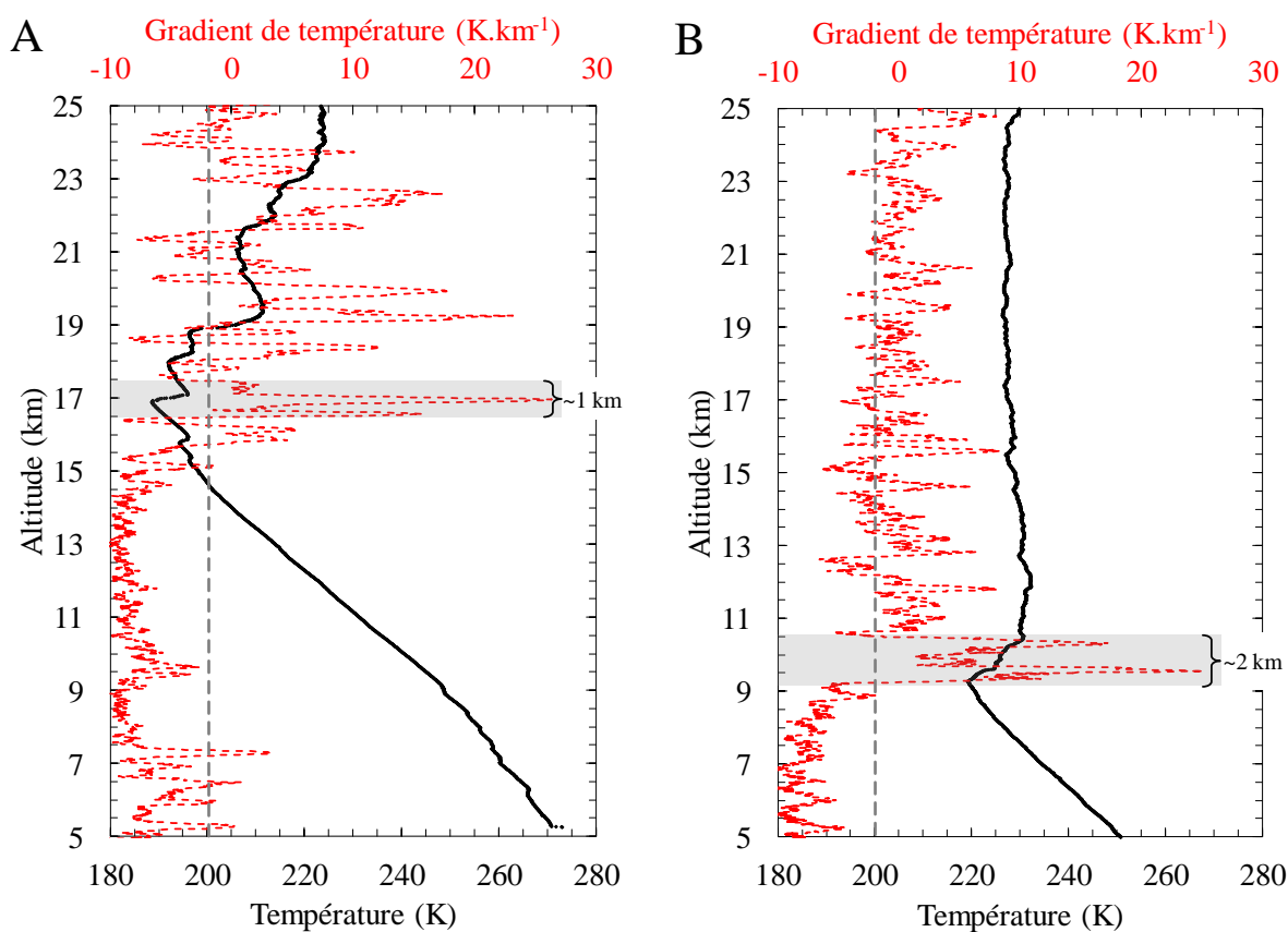
Figure 3-3 : Profils verticaux de la température (en K ; en noirs) et gradient de la température (en K.km^{-1} ; en rouges) ; A : au-dessus de Teresina au Brésil ( 5^{\circ}S ) en juin 2008 mesurés par SPIRALE et B : au-dessus de Kiruna en Suède ( 68^{\circ}N ) en août 2009 mesuré par une radiosonde Vaisala (type RS92).
