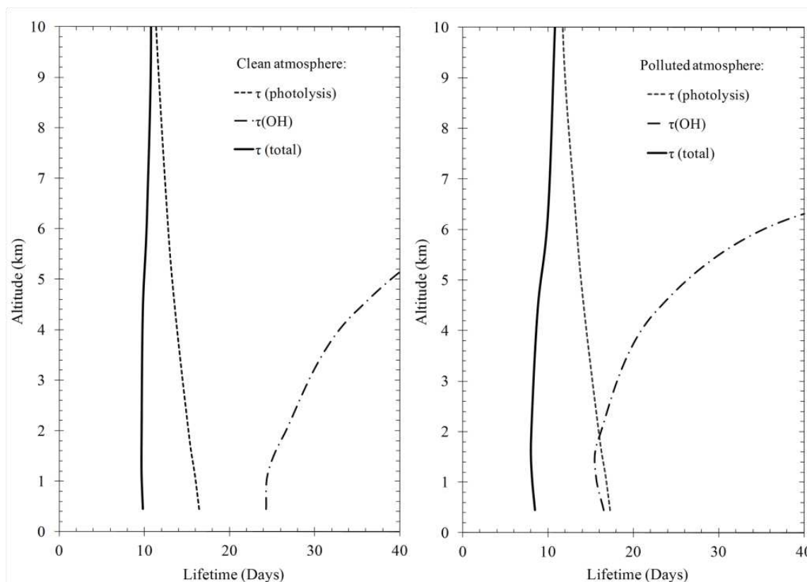
Figure 5-5 : Temps de vie total de CHBr 3 \tau_{\text{total}} (ligne noire en gras) dans tout le domaine de simulation influencé par la réaction avec OH (ligne en tiret-point) et par la photodissociation (ligne pointillée) pour une atmosphère propre (figure de gauche) et pour une atmosphère modérément polluée (figure de droite).
