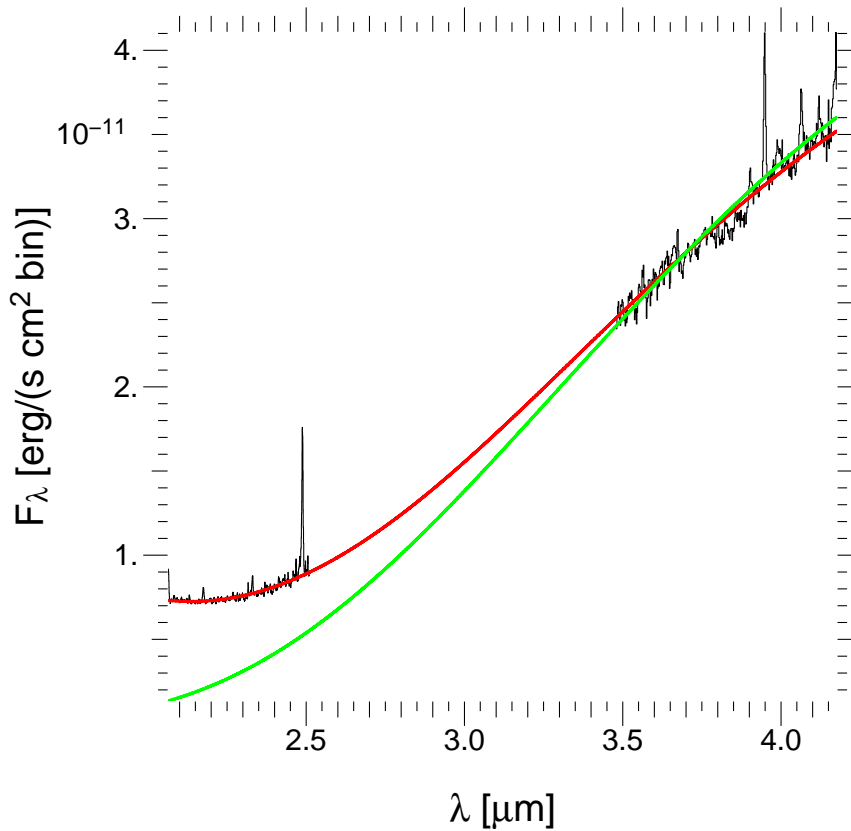
Figure 4.5: Spectre en bande Ks et L' ajusté par un corps noir à 500 K (vert) et par la somme d'un corps noir et d'un corps gris (rouge).
