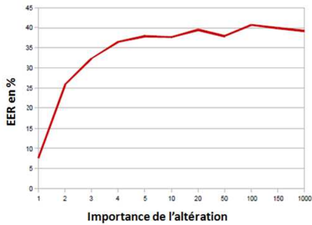
FIG. 2.4 – Evolution des valeurs de l'EER en fonction de la quantité des altérations.
