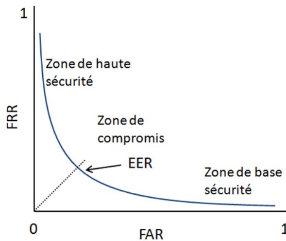
FIG. 2.2 – Exemple de la courbe ROC : Variation du FRR en fonction de FAR lorsque le seuil de décision varie.
