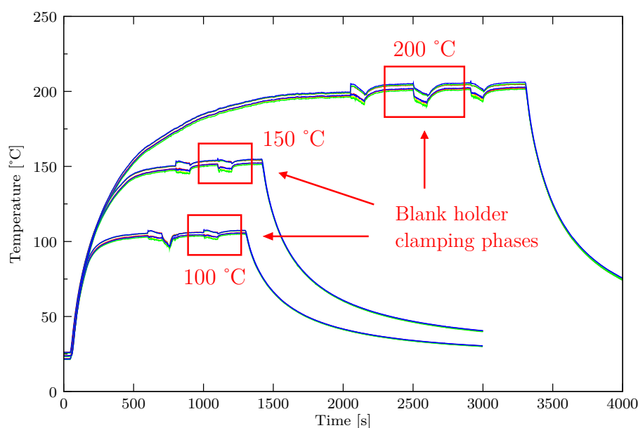
FIGURE 3.10 – Évolutions de la température des sept thermocouples serti sur le flan lors des essais de mise en chauffe à 100, 150 et 200 °C.
