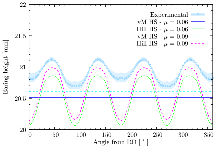
FIGURE 2.37 – Influence du critère de plasticité sur l'effet de corne (Maillage M2, élément SC8R-15pts et un écouissage de Hockett-Sherby).
