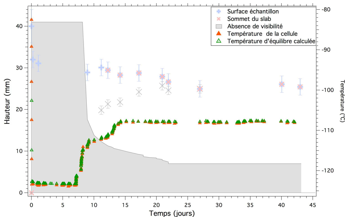
FIGURE 6.6 – Evolutions journalières des hauteurs de l'échantillon de neige et du slab de glace de CO 2 (A), et évolution des températures (B) dans la cellule. L'échantillon est mis en place à t=0 (jour 1). La température initiale à la base de la cellule est -123,5 °C. Avant le troisième jour le slab n'est pas visible à cause du givre sur la vitre latérale d'observation. La zone grisée sur le graphique B. repère l'absence de visibilité, par l'écart de 7 mm entre le fond et le bas de la fenêtre, et par le givre : jusqu'au 9 ème jour l'aire totale de la vitre en est recouverte, ensuite il disparaît progressivement depuis le centre. La température de la cellule est celle mesurée dans la base en cuivre, et température d'équilibre calculée est la valeur théorique associée à la pression mesurée dans la cellule. L'évolution aux premières heures est présentée plus précisément en Figure 6.12.
