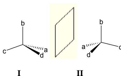
Figure 11: couple d'énantiomères
