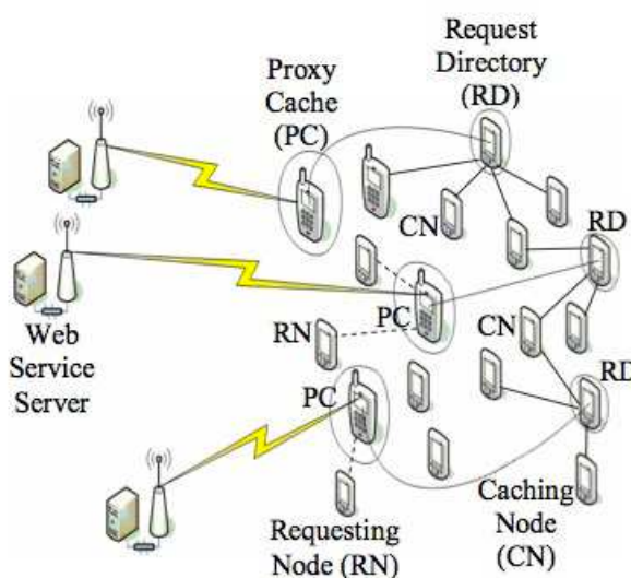
Figure 10 : Architecture du cache distribué proposé dans [91]
