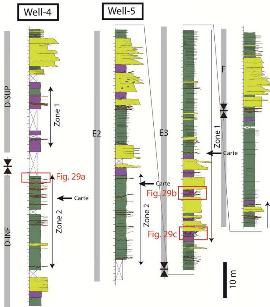
Fig. 6.27 : Logs du puits 4 et 5 interprétés en termes d'association de faciès grâce aux carottes et log d'images. Les limites d'unité des complexes E et D, ainsi que les zones à injectites décrites dans le texte, sont montrées sur la figure. La localisation de la figure 6.29 est également montrée.
