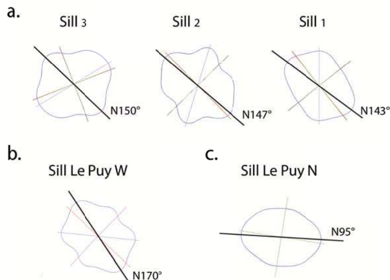
Fig. A5.12 : Orientations préférentielles des minéraux de cinq sills par la méthode des intercepts. (a) L'orientation des grains issus des trois niveaux de sill de l'affleurement du Ravin de la Beume donnent tous une direction proche de N145^\circ . (b) L'orientation des grains du sill/wing situé à l'Ouest de la colline du Puy est de N170^\circ . (c) L'orientation des grains du sill/wing situé au Nord de la colline du Puy est de N95^\circ . Voir figure A5.4 pour la localisation des affleurements.
