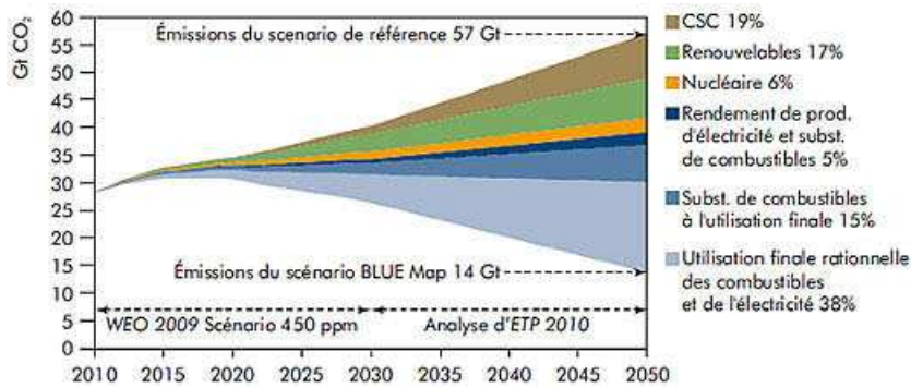
FIGURE 1.4 – Options de réduction des émissions de \text{CO}_2 , 2010-2050. Source : Ministère de l'écologie, du développement durable et de l'énergie - Données : AIE. Le scénario BLUE Map est comparé au scénario de référence.
