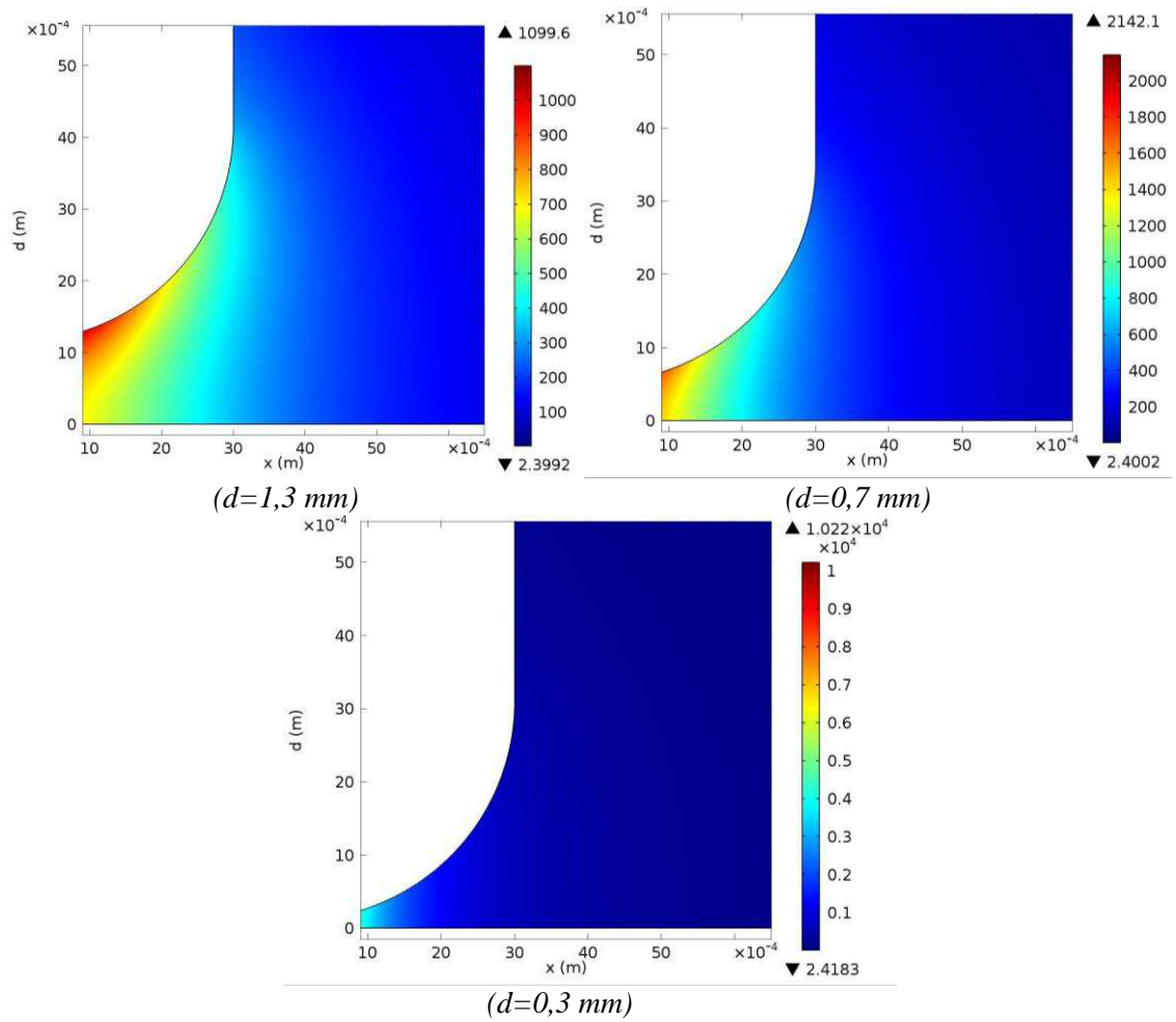
Figure 37. Des cartographies du champ en surface de la cathode en fonction du rayon de disque. Valeur de champ électrique local en \text{V.m}^{-1}
