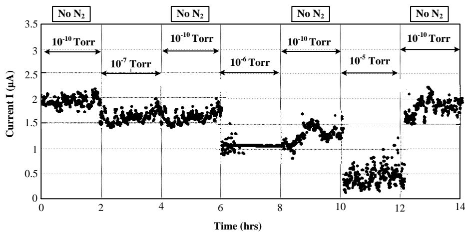
Figure 98. Effet de l'azote sur le courant noir [75]
