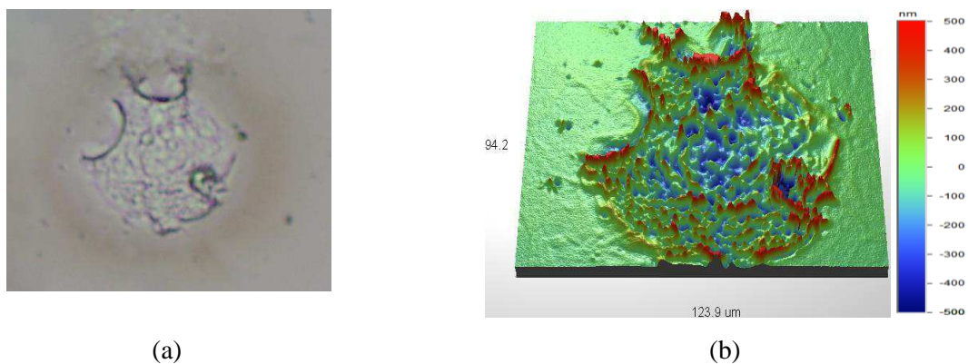
Figure 87. Cratère produit par un claquage : a) image prise par un microscope optique ( \times 50 ) b) profilé 3d pris par un profilomètre optique
