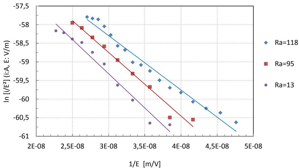
Figure 84. Tracé de Fowler-Nordheim à partir des données présentées dans la Figure 83. R_a est en nm
