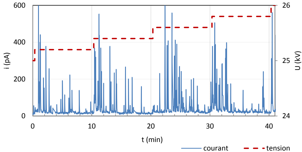
Figure 70. Résultat expérimental montre le conditionnement du courant pour d=500\mu\text{m} , p=3\times 10^{-6} Pa
