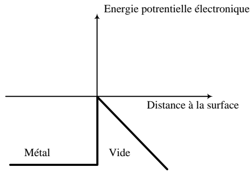
Figure 4. Exemple de forme de barrière de potentielle utilisée dans [5] : barrière « triangulaire »
