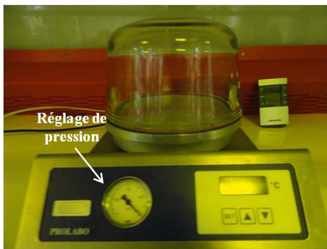
FIGURE 2.30 – Enceinte à vide utilisée dans le procédé de préparation du PDMS.
