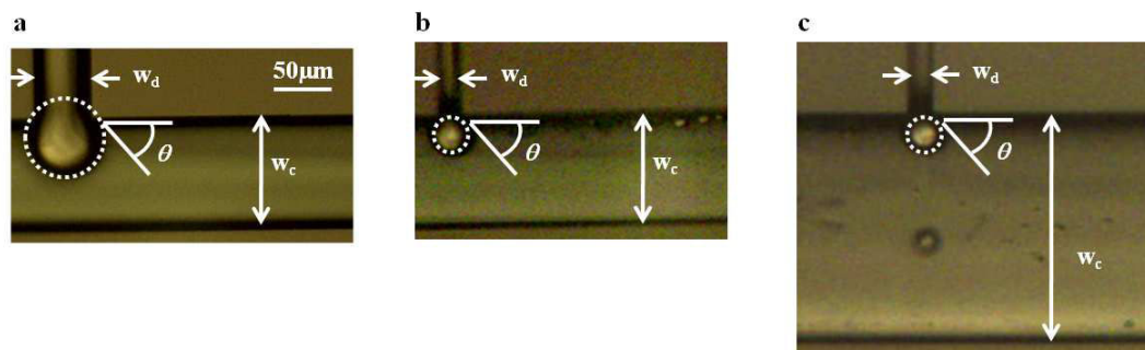
FIGURE 3.5 – Formation de la gouttelette dans le régime dripping : fin du stade I, avec : \bar{v}_d = 1,5\ \text{cm/s} , \bar{v}_c = 7,5\ \text{cm/s} , h = 46\ \mu\text{m} et w_d = 50\ \mu\text{m} , w_c = 100\ \mu\text{m} (a), w_d = 20\ \mu\text{m} , w_c = 100\ \mu\text{m} (b), w_d = 20\ \mu\text{m} , w_c = 200\ \mu\text{m} (c).
