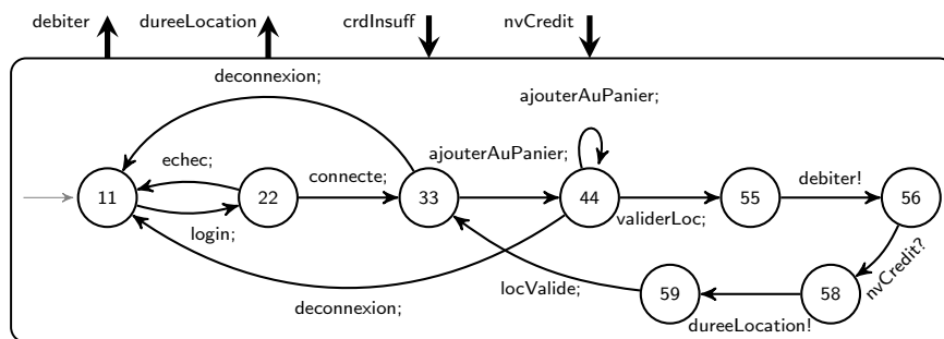
FIGURE 4.4 – Automate d'interface composite A_C || A_S
