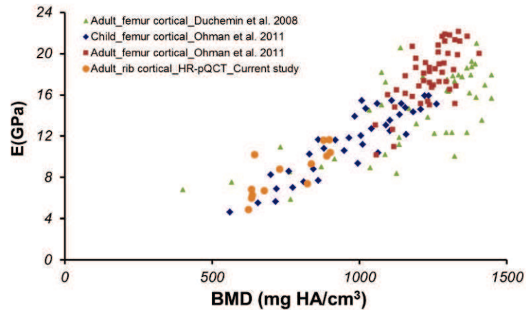
Figure A3.11: Les relations entre la DMO et les propriétés mécaniques (les données de Öhman et al., 2011 sont issues d'une combinaison des résultats de Öhman et al., 2011 et Kaneko et al., 2003).
