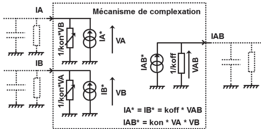
Figure 6.7 : Modèle conservatif du mécanisme de complexation.
