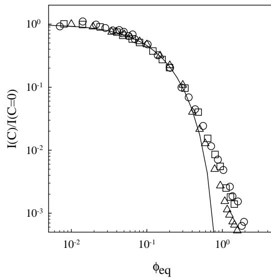
Figure 21 : Évolution de I(C)/I(C=0) en fonction de la fraction volumique effective \phi_{eq} pour les étoiles figées in situ ( \circ ) et les étoiles figées à 10 \text{ g.L}^{-1} ( \square ) et 300 \text{ g.L}^{-1} ( \Delta ). La ligne correspond à l'équation 1.
