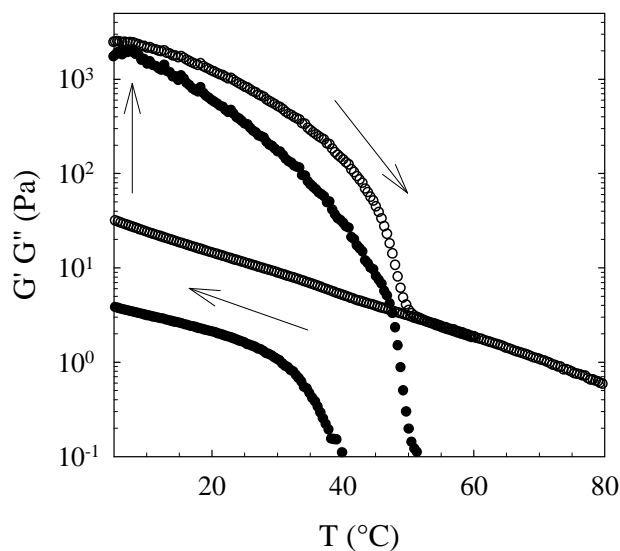
Figure 25 : Évolution des modules de conservation G' (●) et de perte G'' (○) en fonction de la température, pour des étoiles réticulées à 110\text{ g.L}^{-1} et mesurées à 250\text{ g.L}^{-1} , N_{ag} = 63 .
