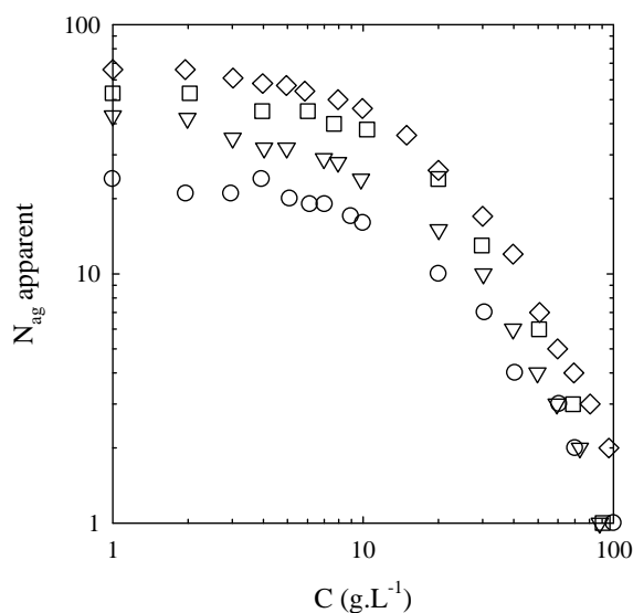
Figure 29 : Évolution du nombre d'agrégation apparent en fonction de la concentration pour des chaînes de copolymère avec : DP5 ( \circ ), DP7 ( \nabla ), DP10 ( \square ) et DP12 ( \diamond ).
