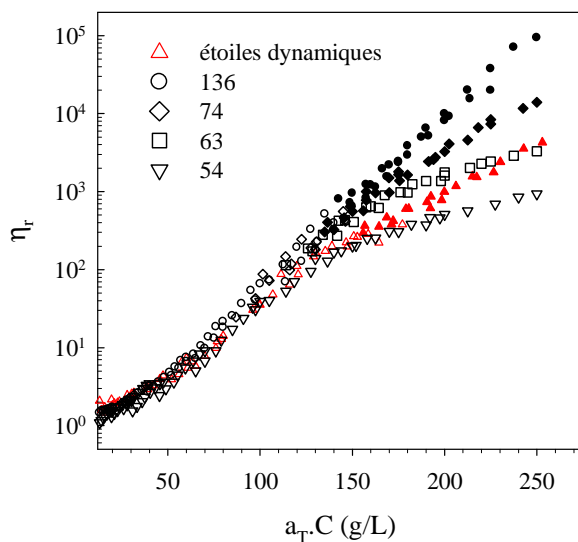
Figure 24 : Courbes maîtresses de la viscosité relative \eta_r en fonction de la concentration pour les différents systèmes étudiés. La température de référence choisie est 20^\circ\text{C} .
