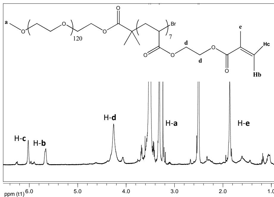
Figure 14 : Spectre RMN 1 H du copolymère dibloc amphiphile POE-b-PAME (solvant : DMSO-d6).
