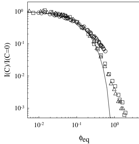
Figure 3 : Évolution de I(C) / I(C=0) en fonction de la fraction volumique effective pour les POE précurseurs ( \circ ), les étoiles dynamiques ( \Delta ) et les étoiles figées ( \square ). La ligne représente l'équation 1.
