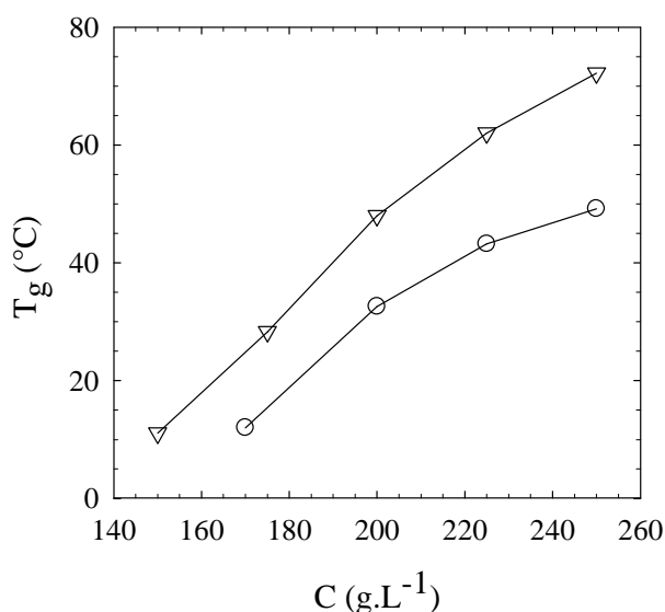
Figure 10 : Évolution de la température de solidification en fonction de la concentration pour des étoiles dynamiques (○) et des étoiles figées (▽) in situ.
