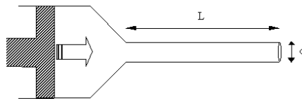
Figure 1-29 Viscosimètre de type extrusion
