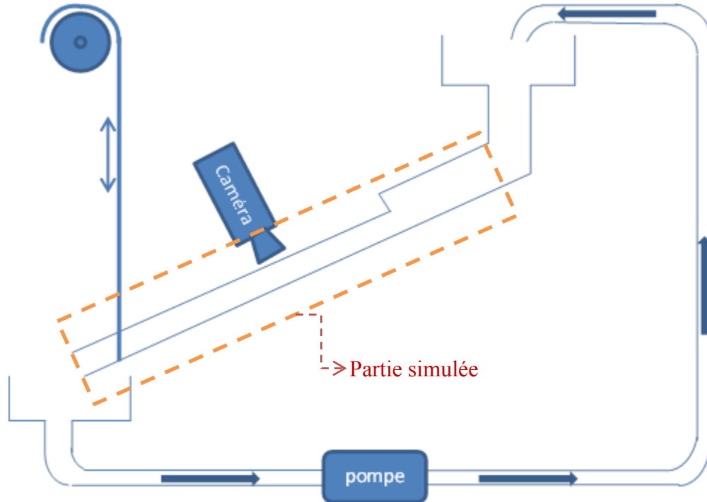
Figure 5-2 Partie simulée du système de pompage
