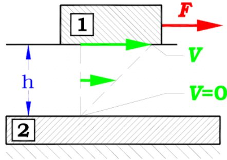
Figure 1-51 Cisaillement de la couche limite développée entre la paroi du cylindre (1) et le bloc de béton (2) dans un tribomètre (58consmeca.free.fr)
