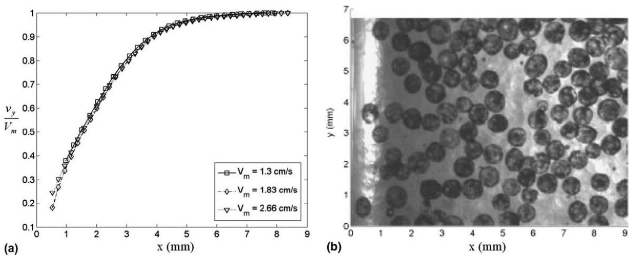
Figure 1-59 a) le profil de vitesse moyenne à travers le canal à différentes vitesses d'entrée pour une suspension de concentration de 45% et la taille des particules est de 650 \mu m. (b) Visualisation de la concentration à la surface libre montrant une concentration uniforme à travers le canal.(Singh, Nir et al. 2006)
