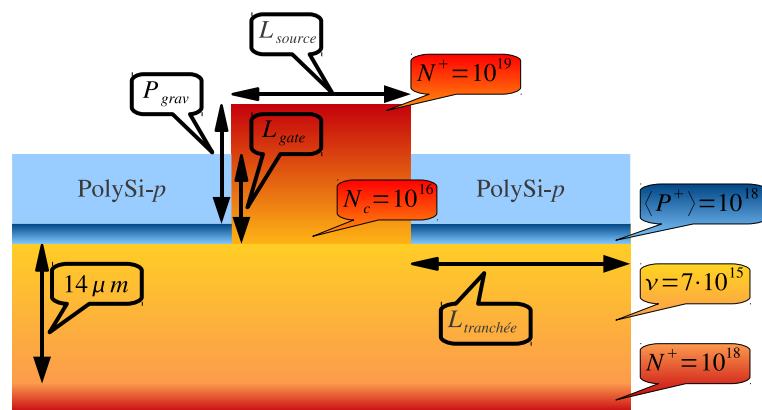
FIG. 4.3: Vue en coupe de la structure de JFET simple à canal vertical
