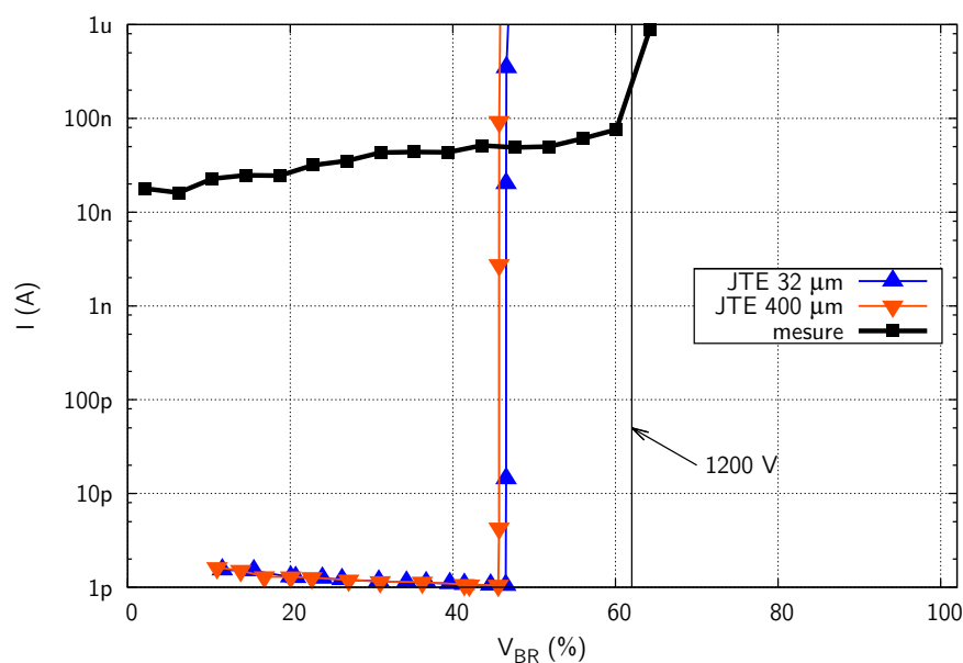
FIG. 2.20: Courbes I(V) de diodes protégées par une JTE courte et une JTE longue
