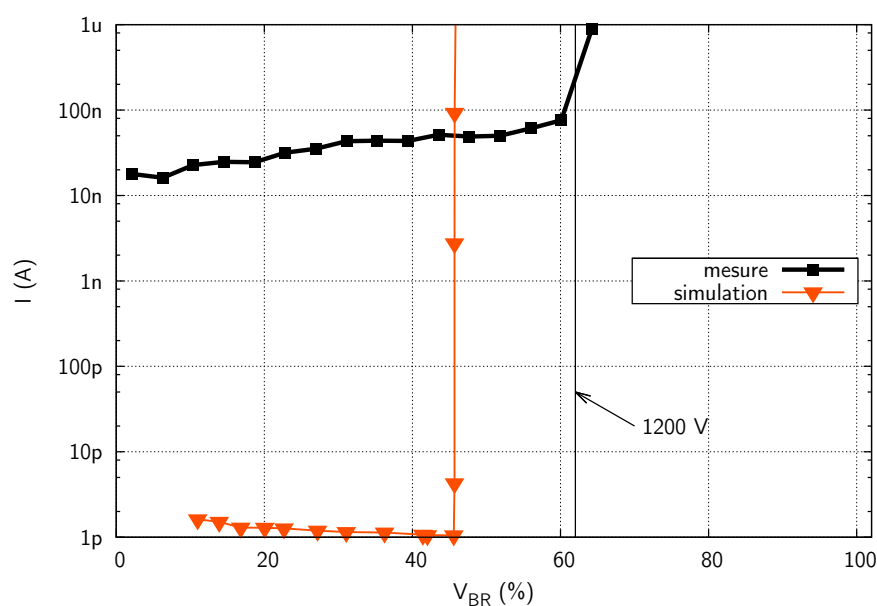
FIG. 2.21: Courbe I(V) de diodes JBS 1200 V de 2 \text{ mm}^2 protégées par une JTE de 400 \mu\text{m} implantée à une dose de 10^{13} \text{ cm}^{-2}
