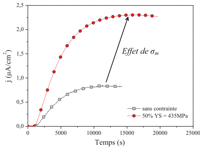
Figure V.18 – Mise en évidence de l'effet de la contrainte sur la courbe de perméation lorsque le AM-2 est soumis à une contrainte de 50% \sigma_{0,2\%} sous j_{ch}=20mA/cm^2 et T=20^\circ C .
