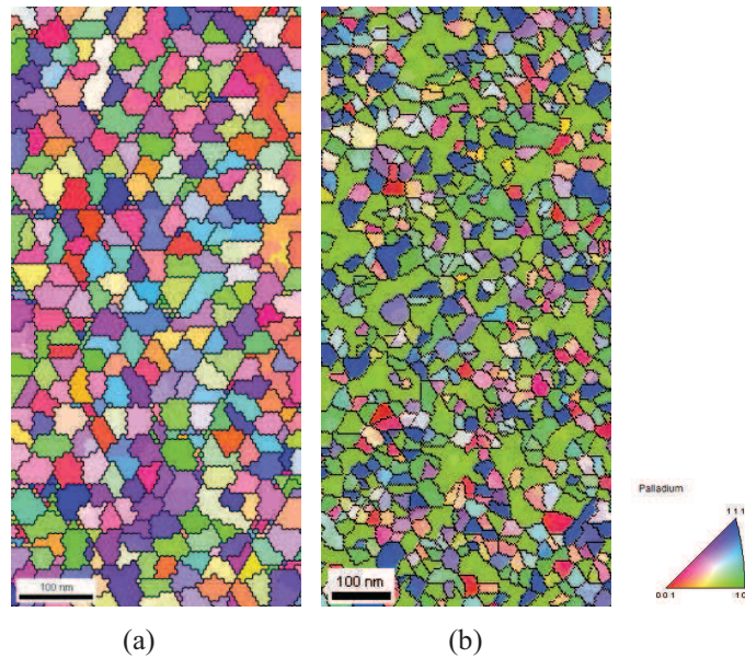
Figure IV.5 – Micrographies EBSD du dépôt de palladium obtenu par PVD magnétron (a) et par électrodéposition (b).
