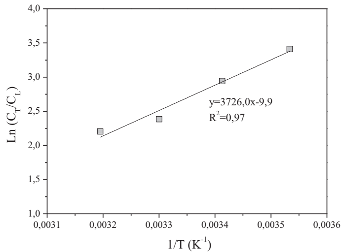
Figure III.21 - Evolution de \text{Ln}(C_T/C_L) en fonction de l'inverse de la température T pour la détermination de l'énergie de piégeage \Delta E_T .
