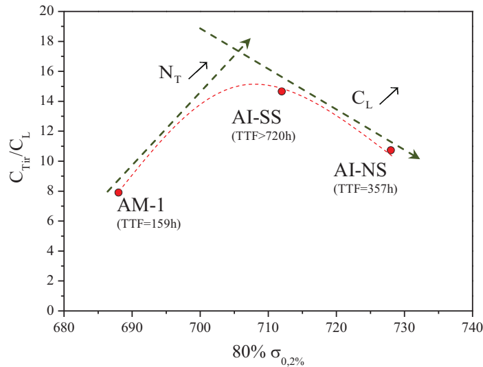
Figure 2 - Evolution de C_{Tir}/C_L en fonction de 80% \sigma_{0,2\%} pour les trois alliages étudiés en perméation sous contrainte.
