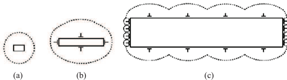
Figure V.11 - Représentation schématique de la cohérence des précipités. (a) Cohérent, (b) semi-cohérent avec un taux de désaccord cristallographique légèrement accommodé par les dislocations et (c) semi-cohérents avec un taux de désaccord cristallographique fortement accommodé par les dislocations dont les extrémités sont pratiquement incohérentes (pas de distorsion élastique) [Wei06].
