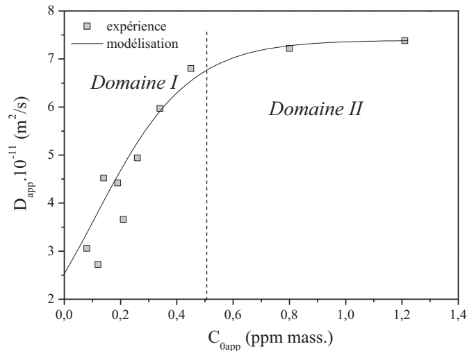
Figure III.14 - Evolution du coefficient de diffusion apparent en fonction de la concentration dans la membrane pour T=20^{\circ}\text{C} .
