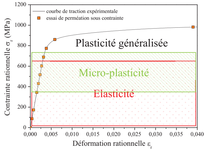
Figure V.2 – Courbe de traction expérimentale et les contraintes appliquées en perméation sous contrainte concernant l’alliage modèle AM-1.
