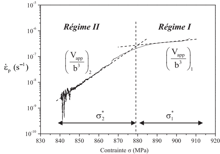
Figure II.17 - Représentation de la vitesse de déformation plastique en fonction de la contrainte pour la détermination du volume d'activation ( b étant la norme du vecteur de Burgers) lors d'un essai à déformation totale constante pour l'AM-1 sous une contrainte maximale de 908 MPa, T=20^\circ\text{C} .
