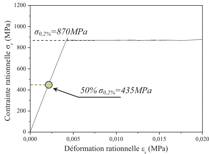
Figure V.17 - Début de la courbe de traction pour l'alliage modèle AM-2.
