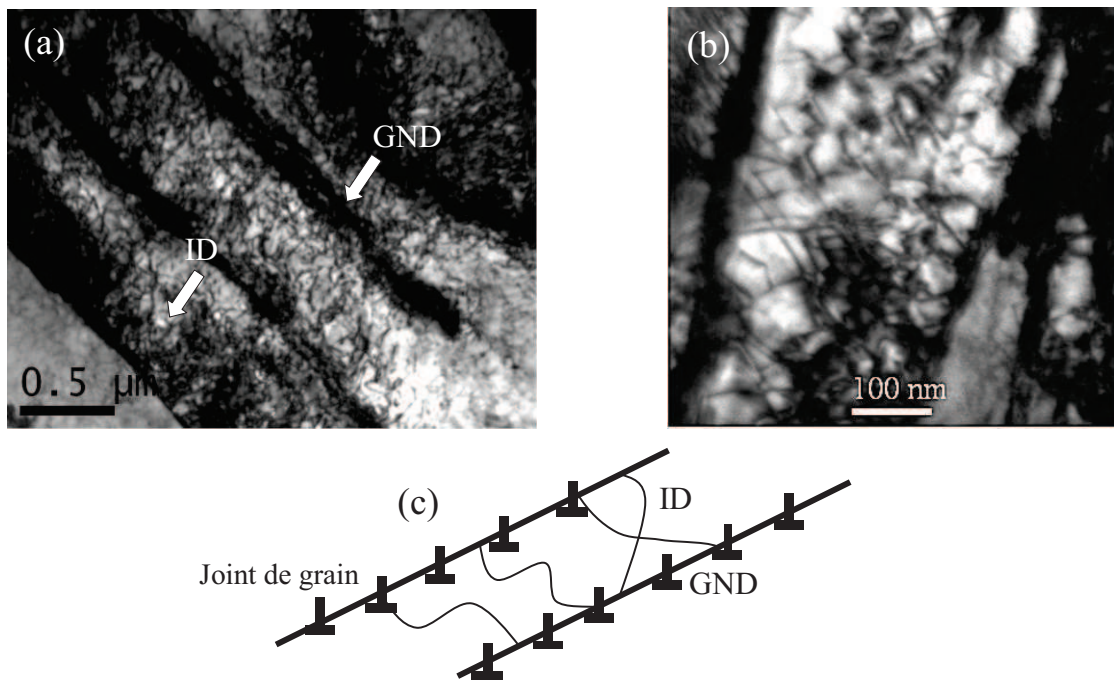
Figure II.9 - Micrographie MET mettant en évidence les dislocations intra-latte dans les cas du AM-2 (a) et du AI-NS (b) et une représentation schématique des dislocations intra-latte et géométriquement nécessaires (c).
