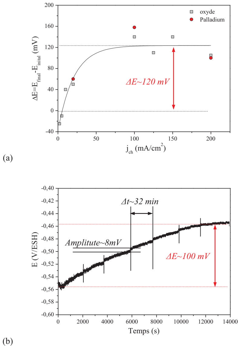
Figure III.11 - Evolution du potentiel de la face d'entrée au cours de l'étape de chargement pour le AM-2 à différentes densités de courant de chargement (a) et dans le cas du AI-SS sous j_{ch}=20\text{mA/cm}^2 et 20^\circ\text{C} (b).
