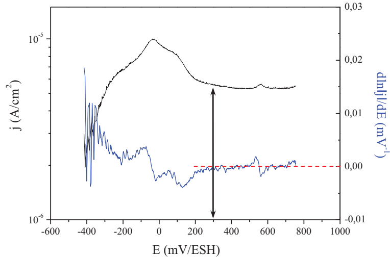
Figure III.6 - Evolutions de la densité de courant anodique j et de la pente de la courbe de polarisation (\frac{\partial \ln|j|}{\partial E})_T en fonction du potentiel E dans 0,1mol/L NaOH sur le AM-2 à 20°C et de surface exposée 1cm 2 .
