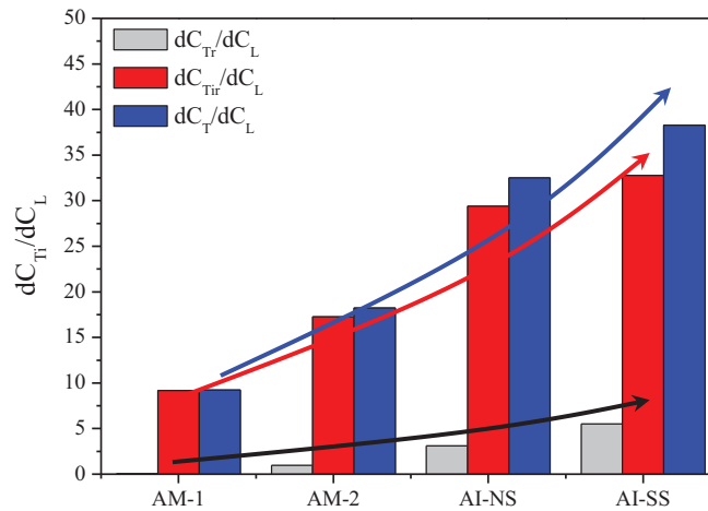
Figure IV.17 - Evolutions des rapports des concentrations C_T , C_{Tr} et C_{Tir} par rapport à C_L (a) et des dérivées des concentrations C_T , C_{Tr} et C_{Tir} par rapport à C_L (b) pour une concentration C \approx 0,6 ppm massique (tous les résultats expérimentaux en annexe 10) .
