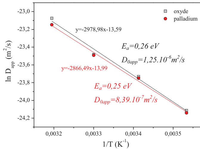
Figure IV.13 – Evolution du logarithme du coefficient de diffusion apparent en fonction de l'inverse de la température ajustée avec une loi d'Arrhenius sous chargement cathodique pour une membrane oxydée ou revêtue de palladium.
