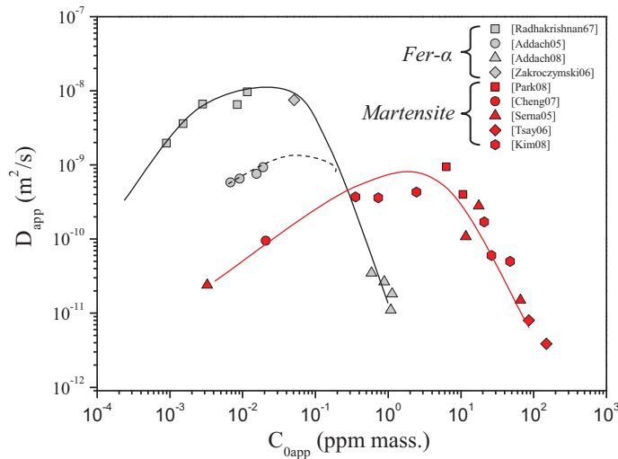
Figure I.22 - Evolution du coefficient de diffusion apparent D_{app} en fonction de la concentration d'hydrogène en sub-surface C_{0app} pour le fer- \alpha et des aciers martensitiques (données issues du tableau en annexe 3).
