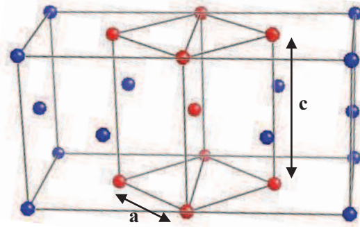
Figure I.1 – Relation de Bain entre un cristal CFC et CC - Maille cristalline tétragonale centrée TC de la martensite, Maille bleue : austénite \gamma (CFC), Maille rouge : martensite (TC), a et c les paramètres de maille
