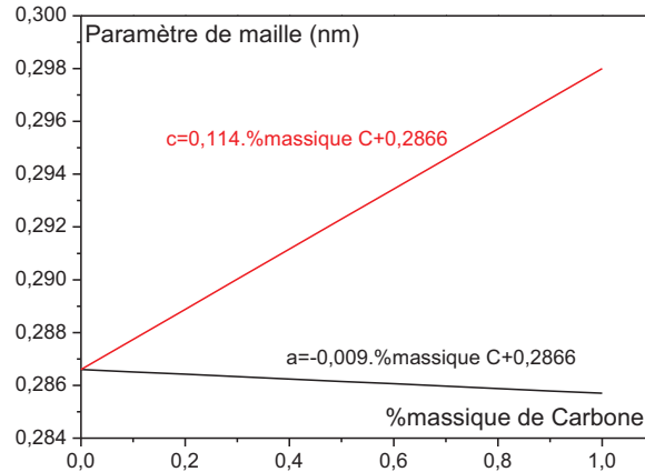
Figure I.4 – Variation des paramètres de maille a et c en fonction de la teneur massique en carbone [Bénard84].
