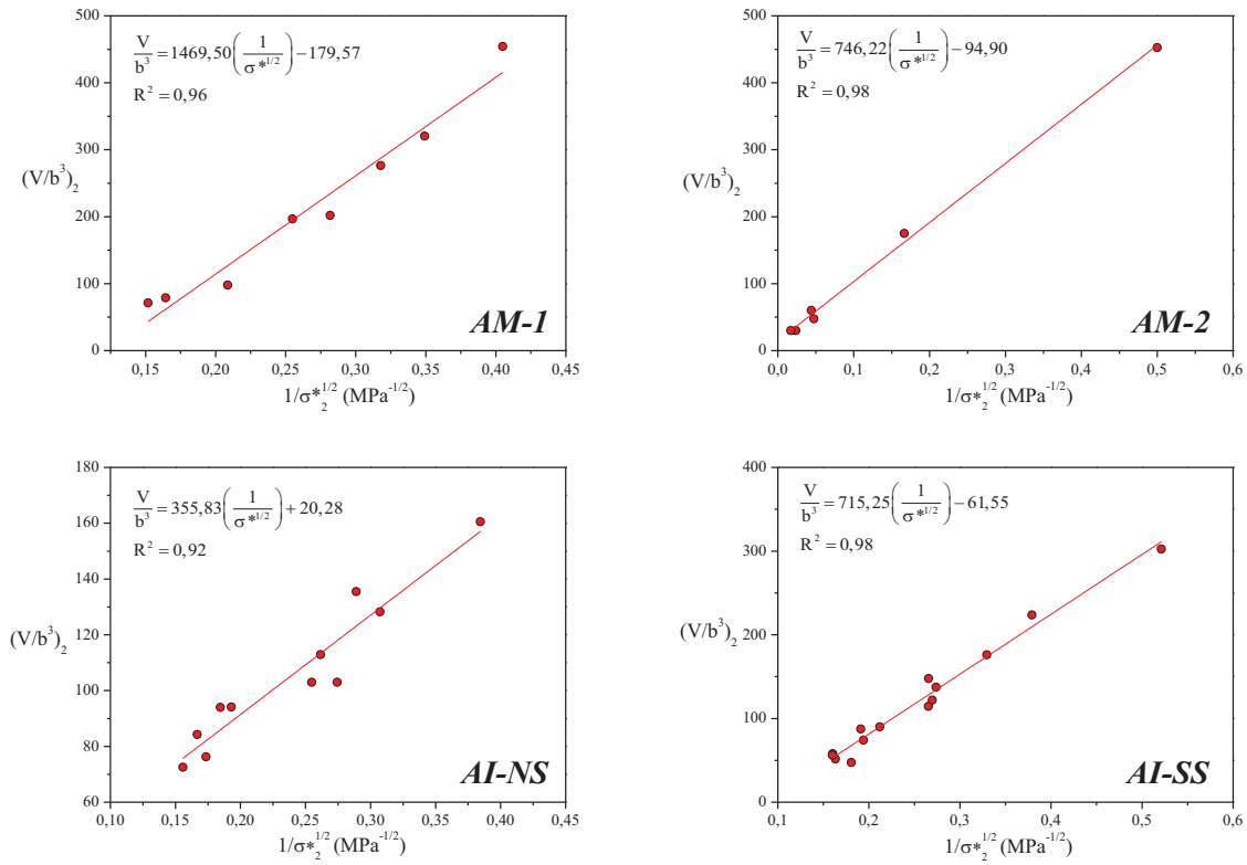
Figure II.20 - Volume d'activation normalisé V/b^3 avec 1/\sigma^{*1/2} du Régime II.
