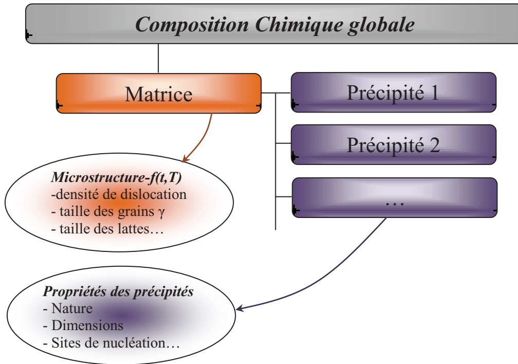
Figure 3 - Architecture utilisée pour la simulation de la précipitation [Kozeschnik04].
