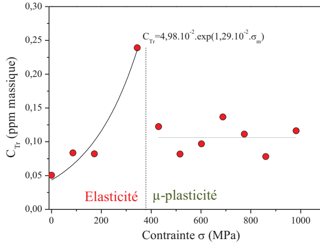
Figure V.10 - Evolution de la concentration en hydrogène piégé réversiblement C_{Tr} en fonction de la contrainte appliquée pour le AM-1 sous 20mA/cm^2 et T=20^\circ C .
