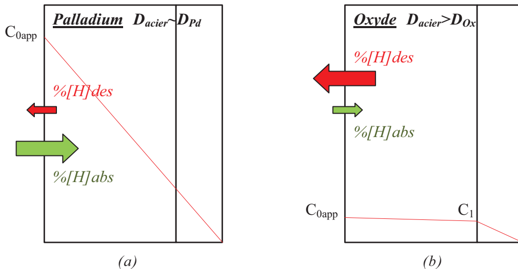
Figure IV.7 - Profil de concentration dans une membrane métallique revêtue d'un film de palladium (a) ou d'un film d'oxyde (b).
