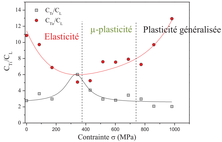
Figure 15 - Evolutions des rapports C_{Tir}/C_L et C_{Tr}/C_L en fonction de la contrainte appliquée pour le AM-1 sous j_{ch}=20mA/cm^2 et T=20^\circ C .
