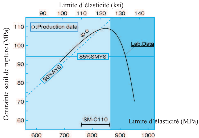
Figure 3 - Evolution de la contrainte seuil de susceptibilité à la SSC en fonction de la limite d'élasticité d'un matériau qualifié Sour Service. Méthode NACE A, solution A, 25°C (AYS=Actual Yield Strength, SMYS=Specified Minimum Yield Strength) [Sumitomo09].
