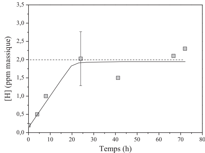
Figure IV.28 - Evaluation de la concentration d'hydrogène en fonction du temps de chargement pour l'alliage AM-2.
