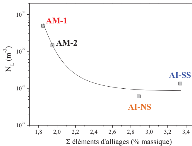
Figure IV.22 – Effet des éléments d'alliage sur l'évolution du nombre de sites interstitiels en considérant les quatre aciers étudiés.
