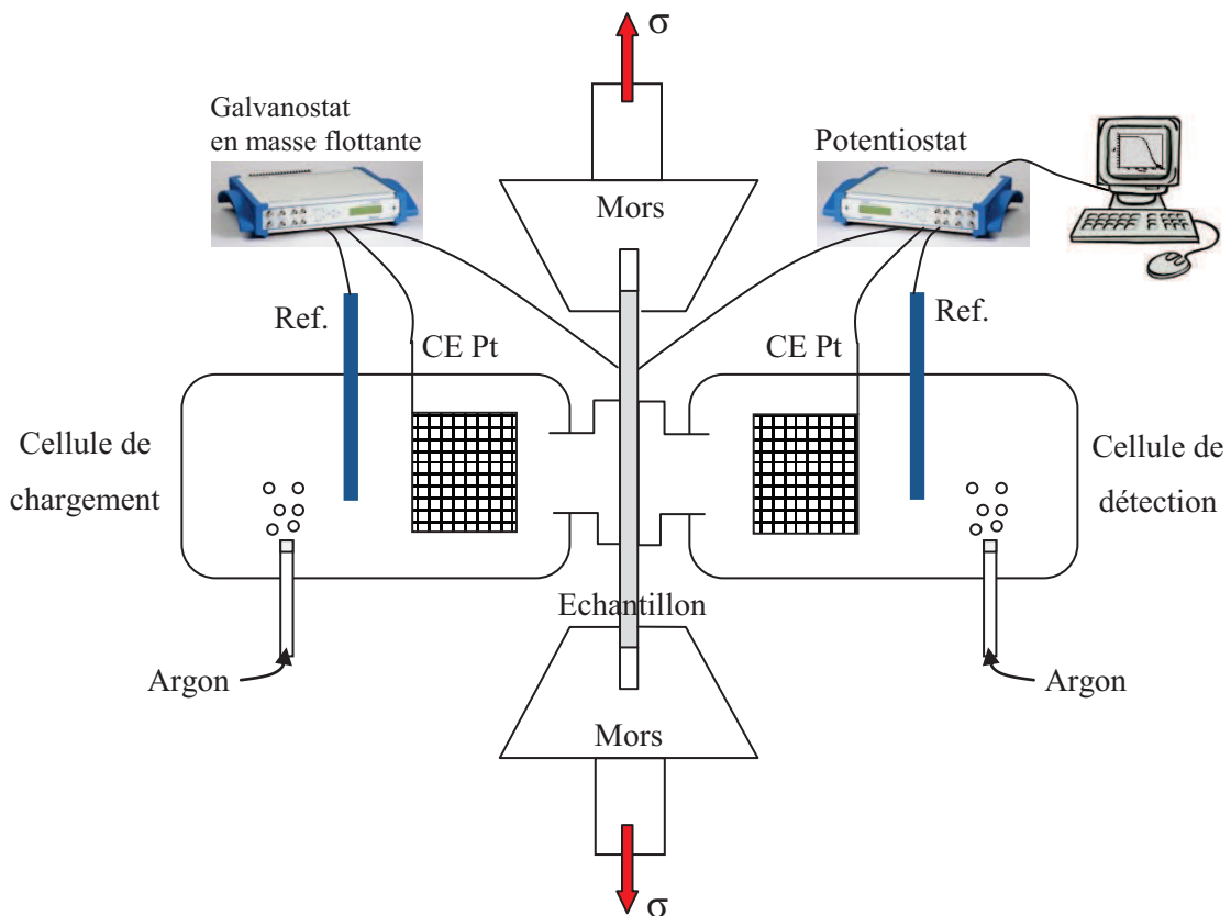
Figure V.1 - Montage expérimental et schéma simplifié de la perméation électrochimique in-situ sous un état de contrainte.
