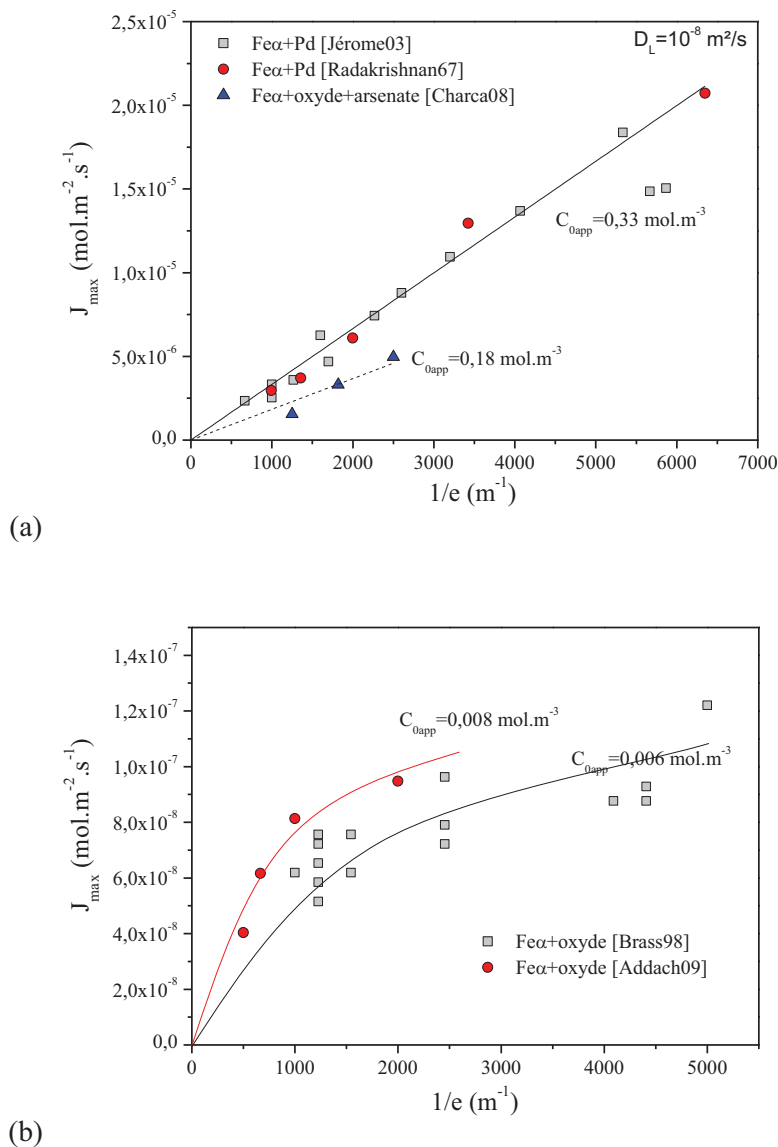
Figure I.17 - Evolution du flux maximale J_{\max} en fonction de l'inverse de l'épaisseur, 1/e pour des membranes palladiées ou oxydées et dopées (a) et oxydées (b).
