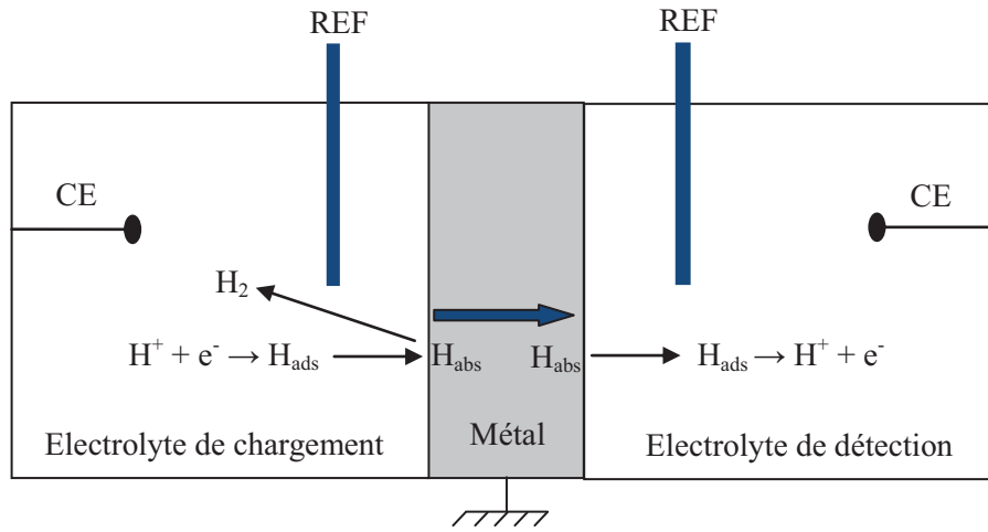
Figure I.13 - Schéma de principe de la perméation électrochimique (REF : électrode de référence, CE : contre-électrode).
