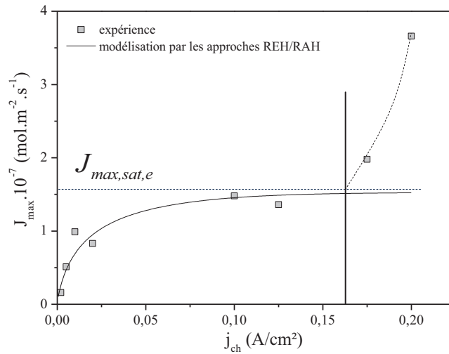
Figure IV.2 - Influence de l'épaisseur pour j_{ch}=20\text{mA/cm}^2 (a) et de la densité de courant cathodique de chargement pour une épaisseur de 1mm (b) sur le flux stationnaire de perméation à 20°C pour l'alliage AM-2.
