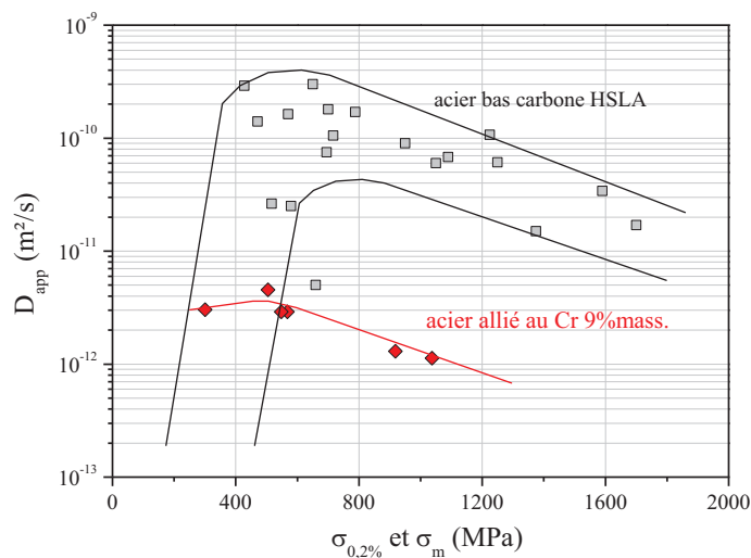
Figure I.24 - Evolution du coefficient de diffusion en fonction de la limite d'élasticité et de la contrainte maximale dans le cas d'aciers bas carbone ou faiblement alliés [Luppo91, Parvathavarthini99, Mendez02, Brass04, Dietzel06, Lunarska08, Dong09].
