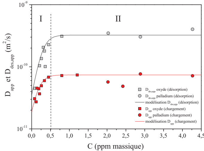
Figure IV.11 - Evolution du coefficient de diffusion apparent de désorption D_{des,app} et de chargement D_{app} en fonction de la concentration moyenne d'hydrogène dans la membrane C sous chargement cathodique avec et sans dépôt de palladium.
