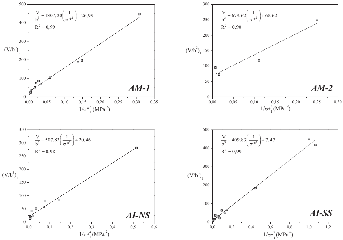
Figure II.19 - Volume d'activation normalisé V/b^3 avec 1/\sigma^{*2} du Régime I.
