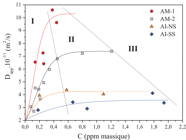
Figure IV.16 - Evolution du coefficient de diffusion apparent D_{app} en fonction de la concentration moyenne d'hydrogène C pour chaque alliage d'étude.
