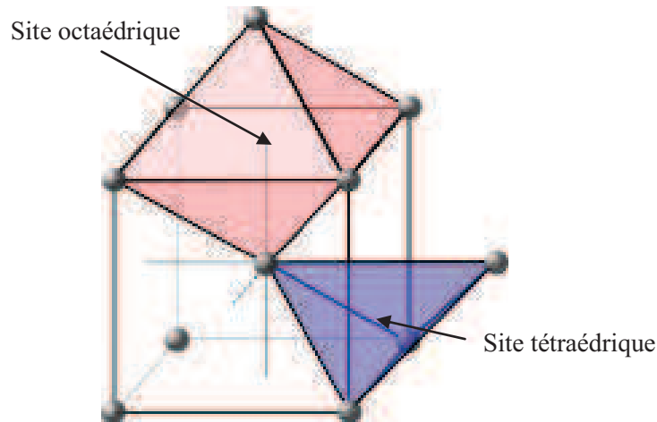
Figure I.3 – Représentation d'un site octaédrique (en rouge) et d'un site tétraédrique (en bleu) dans une maille c.c.
