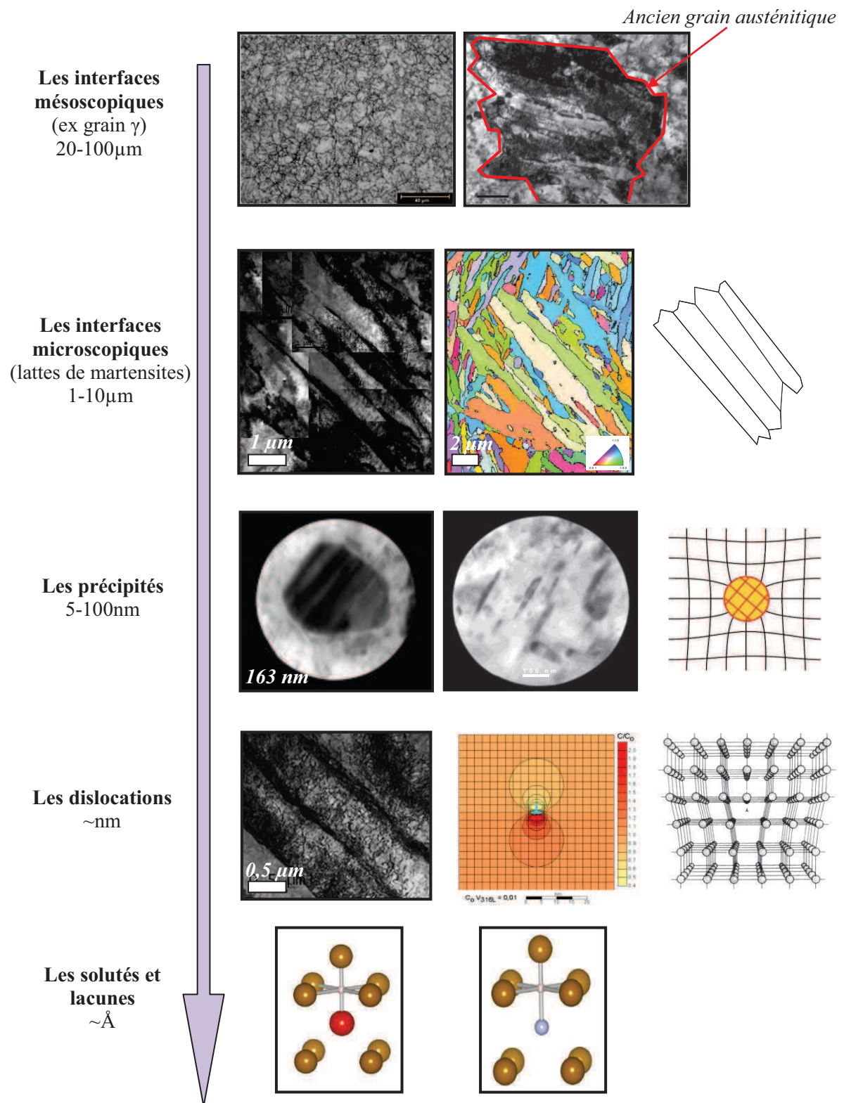
Figure I.10 - Récapitulatif des échelles d'hétérogénéités microstructurales.
