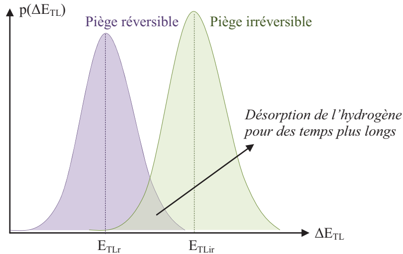
Figure IV.27 - Représentation schématique des probabilités de dépiégeage p(\Delta E_{TL}) en fonction de l'énergie de piégeage afin de mettre en évidence l'effet cinétique du phénomène de dépiégeage.
