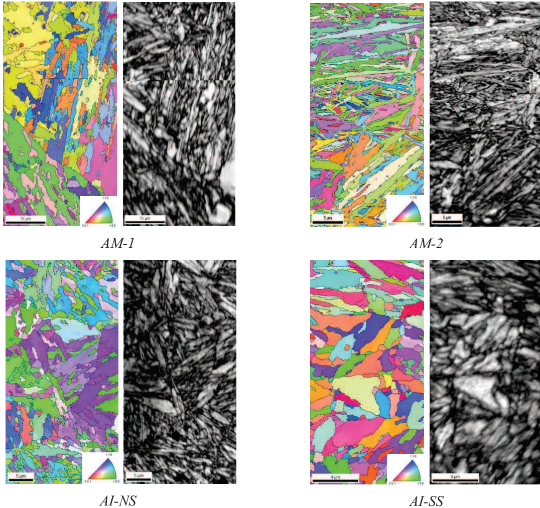
Figure II.2 - Micrographies EBSD des quatre alliages mettant en évidence une diminution des dimensions des lattes de martensite.
