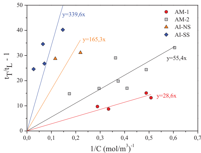
Figure IV.18 - Détermination du nombre de sites de piégeage N_T en suivant t_T/t_L - 1 en fonction de l'inverse de la concentration C pour tous les alliages étudiés.
