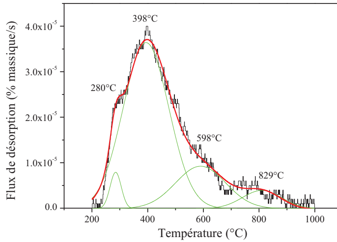
Figure IV.25 - Spectre de désorption thermique et sa modélisation sur le AM-2 chargé cathodiquement à 100\text{mA}/\text{cm}^2 pendant 24h et pour une vitesse de balayage de 114 K/min.
