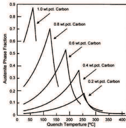
Figure 1.2 - Prédiction de la teneur en austénite résiduelle à partir de différentes teneurs en carbone [Gerdemann04].
