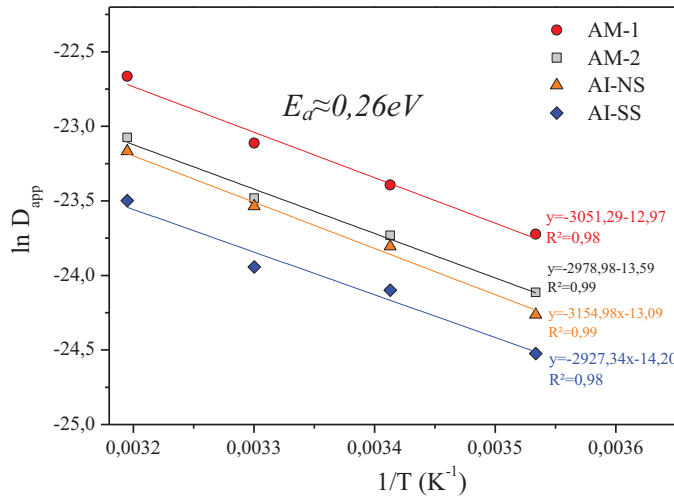
Figure IV.20 – Evolution du coefficient du logarithme du coefficient de diffusion apparent en fonction de l'inverse de la température pour la comparaison de la microstructure.
