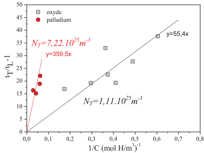
Figure IV.10 - Détermination du nombre de sites de piégeage N_T en suivant t_T/t_L-1 en fonction de l'inverse de la concentration C .
