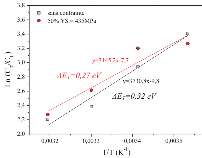
Figure V.21 – Evolution de \ln(C_T/C_L) en fonction de l'inverse de la température T pour la détermination de l'énergie de piégeage \Delta E_T sous j_{ch}=20\text{mA/cm}^2 et T=20^\circ\text{C} pour une contrainte de 50% \sigma_{0,2\%} .
