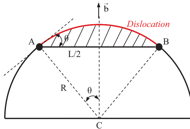
Figure 2 - Représentation d'une dislocation ancrée sur un obstacle.
