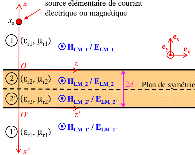
Figure D-1 : Lamme de métamatériau excitée par une source élémentaire de courant infinie suivant \mathbf{e}_y et placée en x = x_s et z = 0 . Les milieux 1' et 2' sont la symétrie des milieux 1 et 2 respectivement par le plan de symétrie (ligne pointillée).
