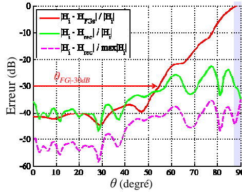
Figure G-1 : Erreur de recomposition observée à r_{obs} = 2.r_0 , en faisant rayonner uniquement les FGs ou en faisant rayonner à la fois les FGs et les CESs. r_{dec} = r_0 .
