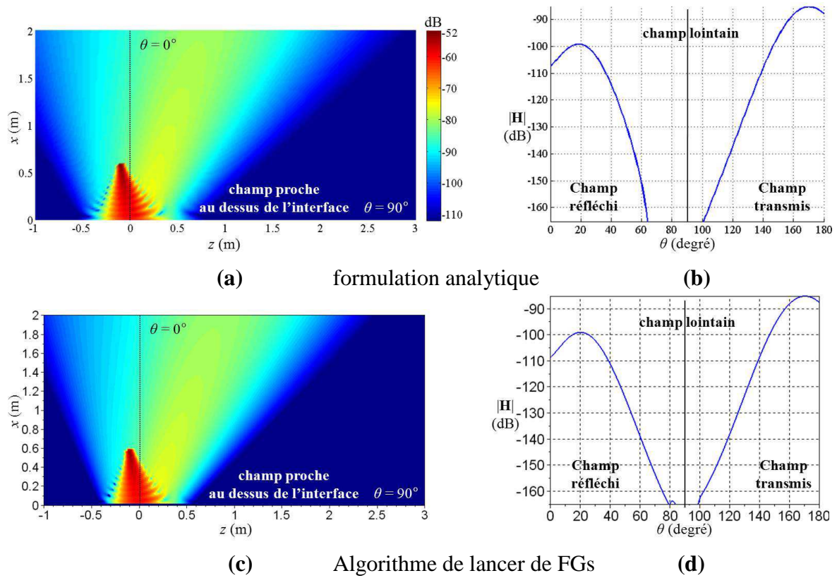
Figure IV-5 : Cas d'un FG incident à \theta_s = -10^\circ sur une lame de diélectrique ( \epsilon_{r2} = 5 , d = 4 cm). (a) et (b) champs obtenus avec notre formulation analytique ; (c) et (d) champs obtenus avec l'algorithme de lancer de FGs.
