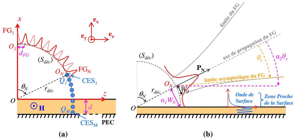
Figure V-3 : (a) Décomposition du champ incident en utilisant à la fois des FGs et des CESs ; Zoom sur la position de O_N , le centre du dernier FG, en fonction de \alpha_1 W_0 , \theta_N , r_{déc} et \alpha_2 \theta_x .
