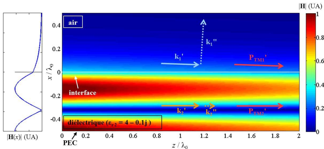
Figure I-25 : Amplitude du champ magnétique et grandeurs caractéristiques d'un mode de surface TM sur une lame de diélectrique sur métal parfait (PEC). UA = Unité Arbitraire.
