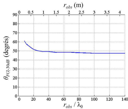
Figure G-4 : Evolution du domaine angulaire de validité des FGs seuls en fonction de r_{obs} , la distance de décomposition. r_{dec} = r_0 .
