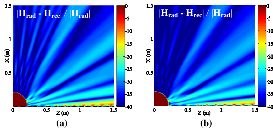
Figure H-4 : Erreurs relatives de recomposition, obtenues avec un pas de maillage en CESs de (a) \lambda/5 et (b) \lambda/8 . r_{dec} = r_0 = 7\lambda_0 , (\alpha_1, \alpha_2) = (1.5, 1) et \kappa = 0.9 .
