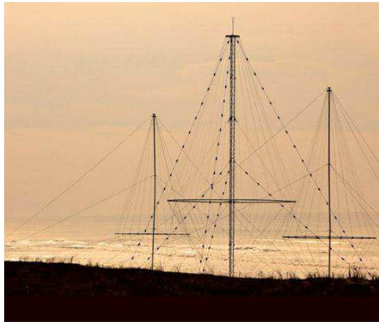
Figure I-2 : Photographie des antennes d'un radar à ondes de surface développé par l'Onera – The French Aerospace Lab. (Crédit photo www.onera.fr )
