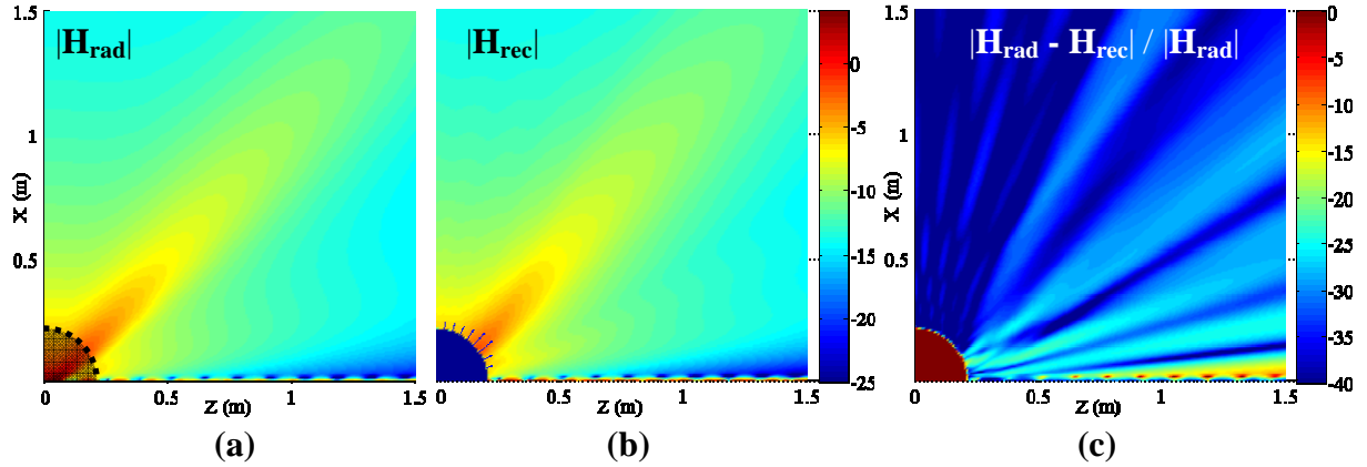
Figure V-6 : Amplitude (en dB ) de (a) le champ de référence et (b) le champ recomposé, normalisés par rapport à \max(|\mathbf{H}^i|) , l'amplitude maximale du champ sur la surface de décomposition ; (c) erreur relative de recomposition. r_{\text{déc}} = r_0 = 7.\lambda_0 , (\alpha_1, \alpha_2) = (1.5, 1) et \kappa = 0.9 .
