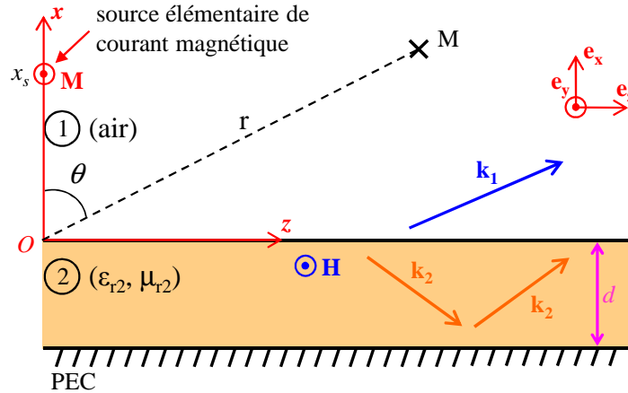
Figure II-11 : lame de métamatériau sur métal parfait (PEC) excitée par une source élémentaire de courant magnétique infini suivant \mathbf{e}_y et placée en x = x_s et z = 0 .
