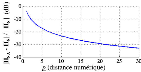
Figure II-7 : Validité de H_{SA} en fonction de la distance numérique.
