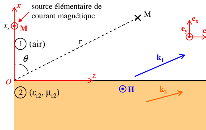
Figure II-3 : Dioptre air-métamatériau excité par une source élémentaire de courant magnétique infinie suivant \mathbf{e}_y et placée en x = x_s et z = 0 .
