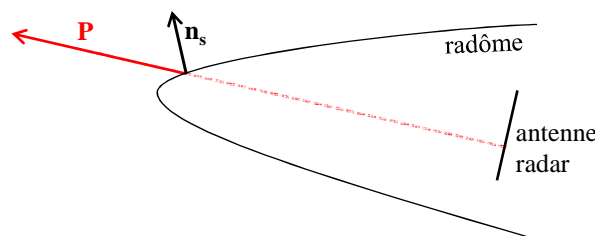
Figure III-6 : Schéma d'un radôme de pointe effilé. Illustration du problème lié à la décomposition d'un champ sur une surface sous forte incidence. Le champ se propage suivant son vecteur de Poynting \mathbf{P} et rencontre la surface en un point où la normale à la surface est \mathbf{n}_s .
