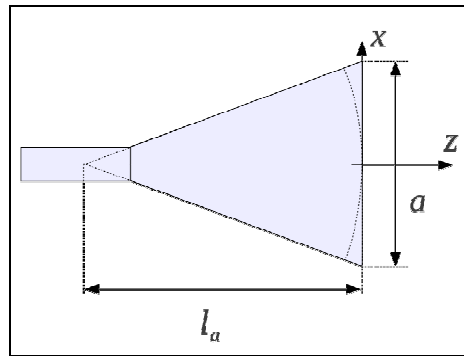
Figure III-9 : Cornet 2D (d'après K. Elis 2012 [122]).
