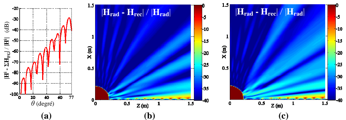
Figure H-2 : (a) Erreur de décomposition en FGs et (b) erreur relative de recombposition, obtenues avec W_0 calculé numériquement ; (c) erreur relative de recombposition, obtenue avec W_0 calculé analytiquement. r_{dec} = r_0 = 7.\lambda_0 , (\alpha_1, \alpha_2) = (1.5, 1) et \kappa = 0.9 .
