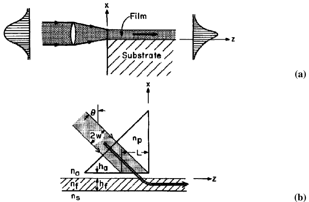
Figure II-1 : Couplage d'un faisceau laser avec une onde de surface dans une lame de matériau en utilisant un coupleur (a) longitudinal et (b) transversal par prisme (d'après T. Tamir, 1979 [80])
