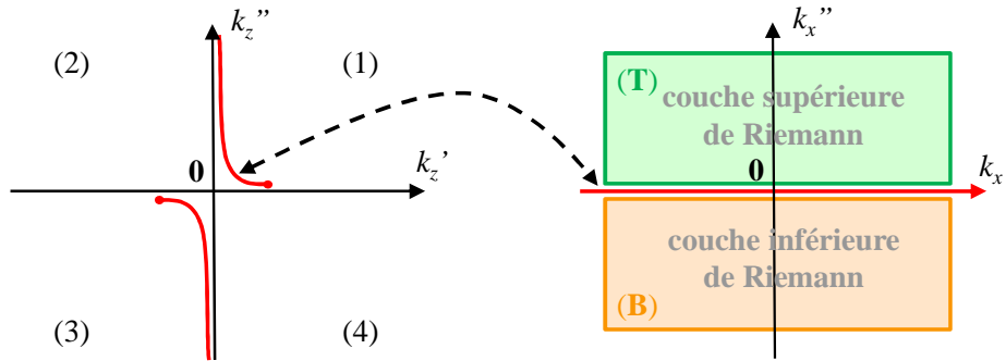
Figure II-4 : Représentation des deux branches de coupure dans le plan complexe k_z ; représentation des deux couches de Riemann dans le plan complexe k_x et lien avec la notion de branche de coupure. On rappelle que k_{x/z} = k_{x/z}' - j \cdot k_{x/z}'' , avec k_{x/z}' et k_{x/z}'' des réels.
