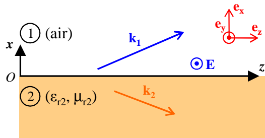
Figure B-1 : Représentation des deux Onde Plane Inhomogène (OPI) constituant une onde de surface TE sur un dioptre air-métamatériau.
