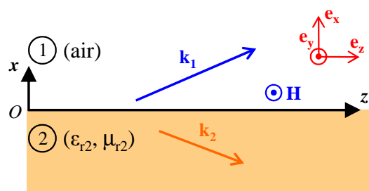
Figure I-14 : Représentation des deux OPI constituant une onde de surface TM sur un dioptre air-métamatériau
