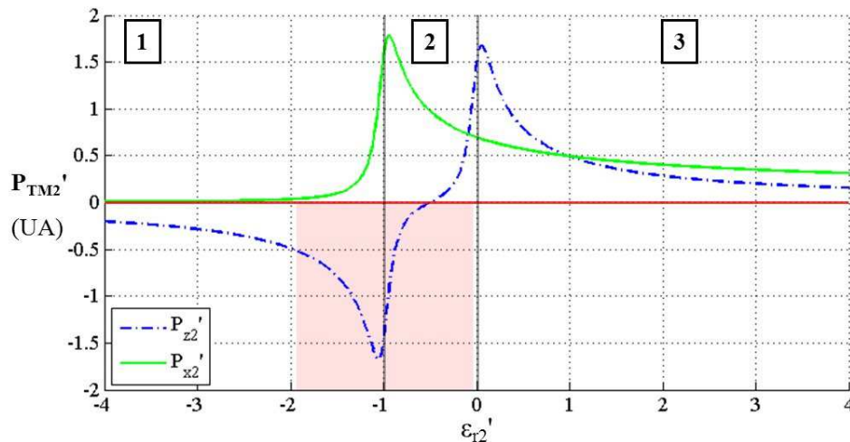
Figure I-18 : Composantes de \mathbf{P}_{\text{TM}2}' (la partie réelle du vecteur de Poynting dans le milieu 2) en fonction de \epsilon_{r2}' (la partie réelle de la permittivité du milieu 2). \epsilon_{r2}'' = 0.1 (pertes modérées). Unité arbitraire.
