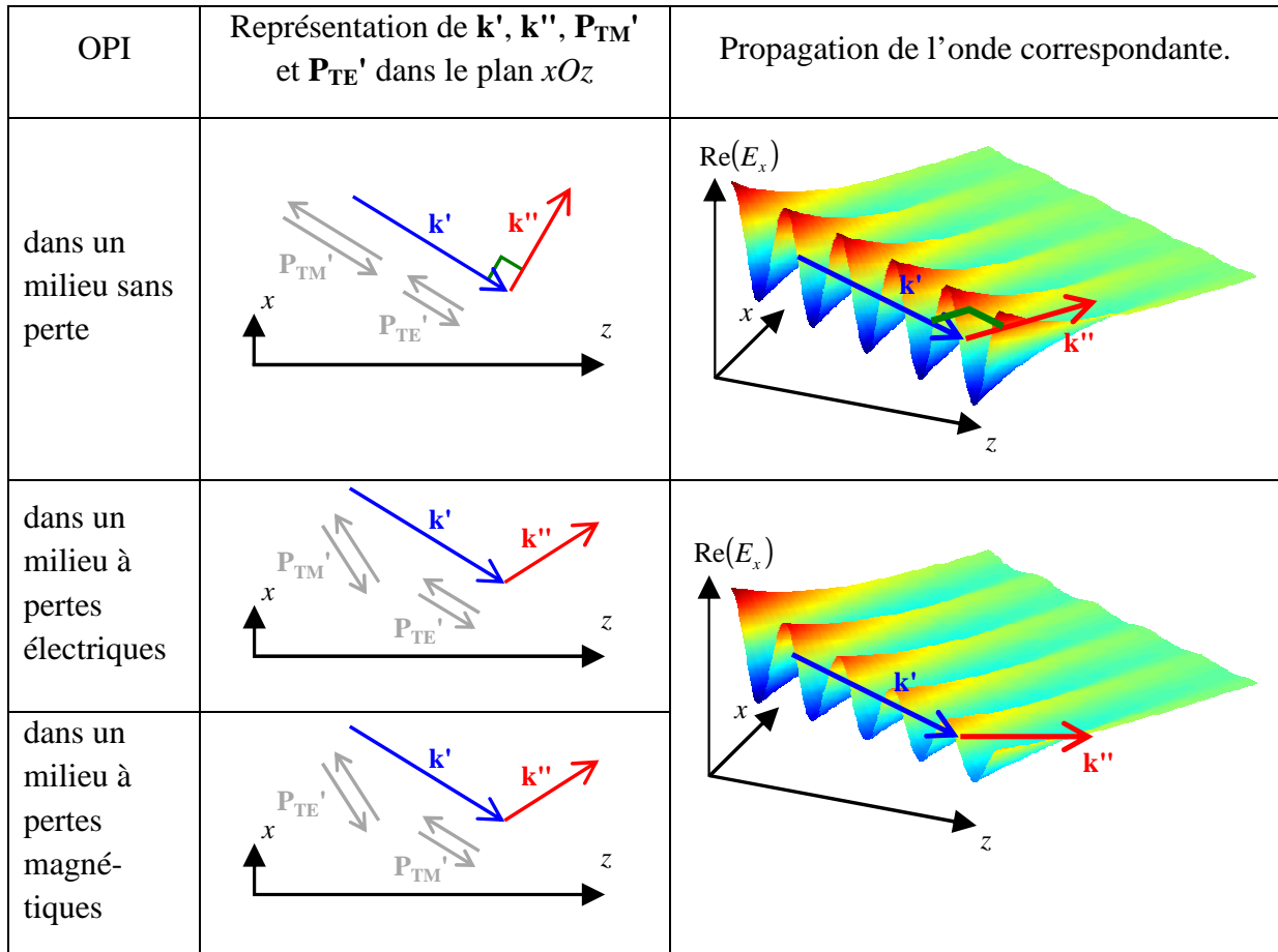
Figure I-7 : Relations angulaires entre les composantes réelle et imaginaire du vecteur d'onde et la composante réelle du vecteur de Poynting pour une OPI dans différents milieux.
