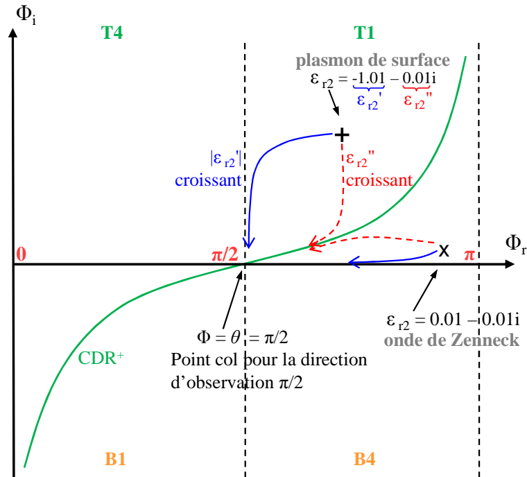
Figure II-9 : Position des pôles \Phi_p correspondant aux plasmons de surface et aux ondes de Zenneck se propageant suivant z_+ , en fonction de la permittivité \epsilon_{r2} du milieu 2 ( \mu_{r2} = 1 ).
