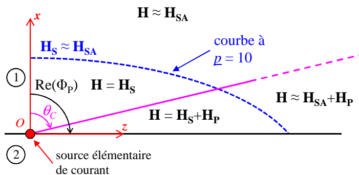
Figure II-8 : Domaines d'existence de H_S et H_P et les domaines de validité de H_{SA} , dans le cas du dioptre.
