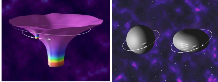
FIGURE 3.6 – Vue d’artiste d’une EMRI. La figure de gauche représente les déformations de l’espace-temps dans le cas d’une EMRI (figure Kip Thorne©), celle de droite l’orbite d’un objet près de l’horizon du trou noir supermassif dans le cas d’un trou noir sans spin (gauche) et avec spin (droite) (figure Don Davis basé sur un dessin de Kip Thorne).
