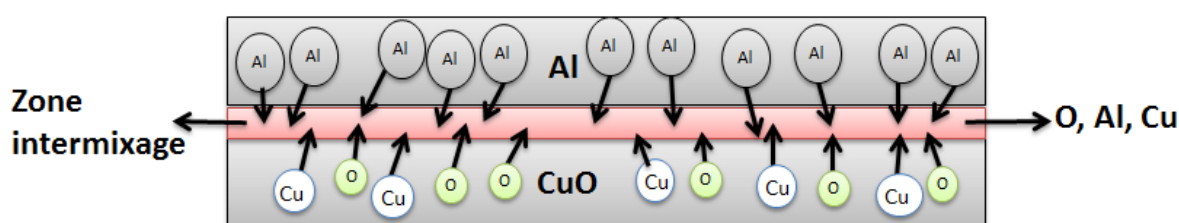
Figure 32. Schéma illustrant la diffusion des atomes Al, Cu et O entre deux couches Al et CuO
