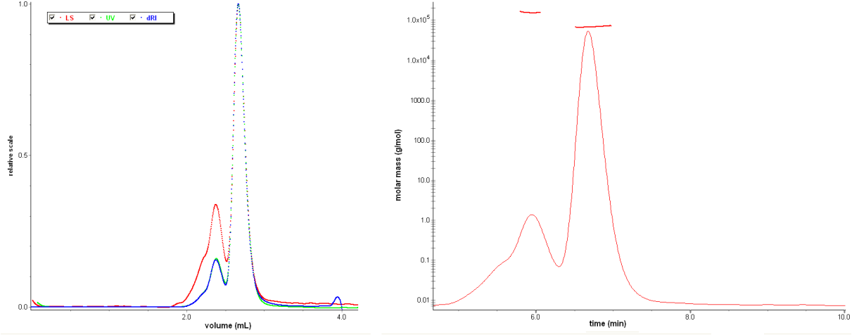
Figure 2.7 – Analyse SEC-MALS de la BSA. Le graphique de gauche montre les profils en sortie de colonne d'exclusion stérique vus par le détecteur de diffusion de lumière (LS), le spectromètre (UV) et le réfractomètre (dRI). Le graphique de droite présente les masses (lignes horizontales) des composés de chaque fraction.
