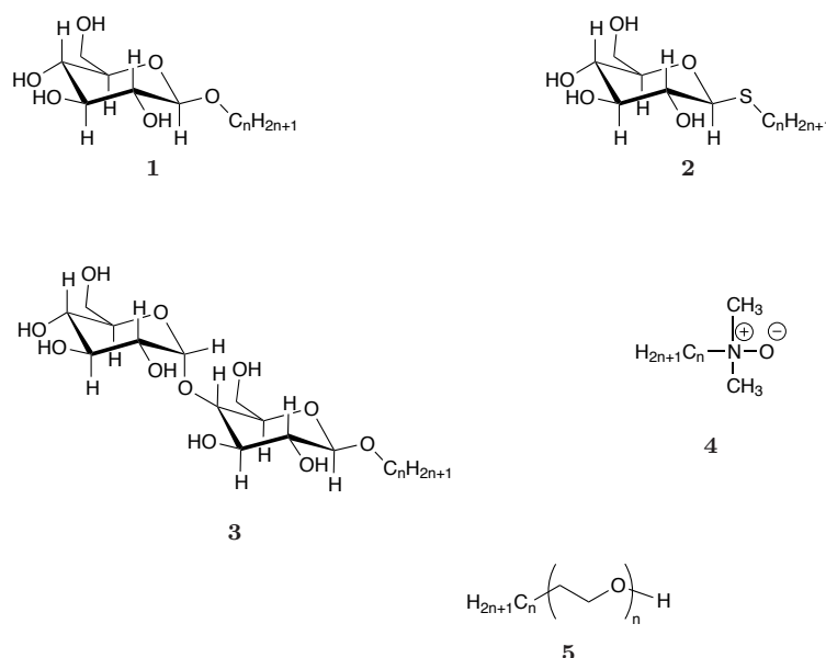
Figure 6 – Structures des détergents classiques
