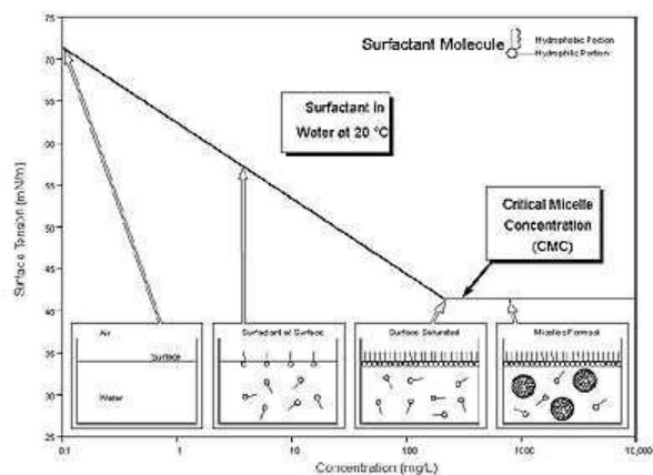
Figure 2.2 – Détermination de la CMC à partir de la courbe de tension superficielle en fonction de la concentration en tensioactif. Image reprise du site www.kruss.de .
