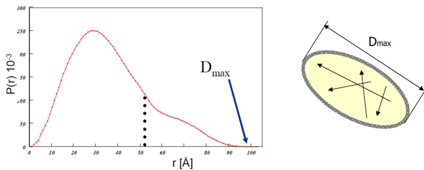
Figure 2.10 – La fonction de distribution des distances
