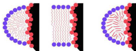
Figure 1.14 – Comparaison schématique des contacts formés à l’interface de la région transmembranaire d’une protéine [114]. A gauche : les chaînes alkyles du tensioactif sont peu ordonnées, il y a une forte interaction entre la protéine et le tensioactif. Au milieu : les chaînes alkyles des lipides de la membrane s’organise de façon parallèle. A droite : les parties rigides du PCC-malt impose un plus grand degré d’organisation que la chaîne alkyle mais moins de contact à l’interface.
