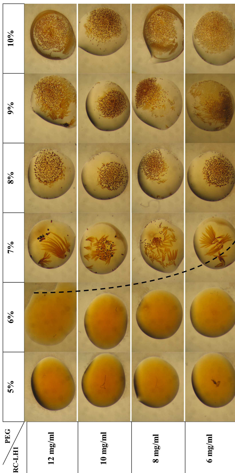
Figure 5.8 – Morphodrome du RC-LH1-puf X en PCC-malt en fonction de la concentration en protéine et en PEG. Technique de la goutte suspendue.
