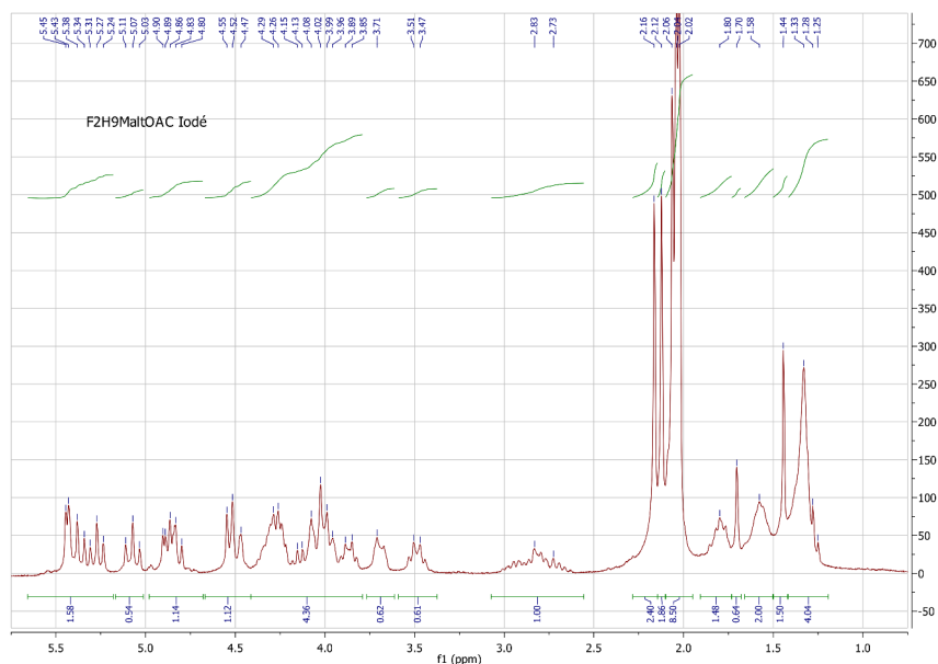
Figure 1.30 – Spectre ^1\text{H} -RMN du composé 25 . Le signal à 2,75 ppm est caractéristique du proton de -\text{CHI} . L'interprétation complète du spectre est donné dans la partie expérimentale.
