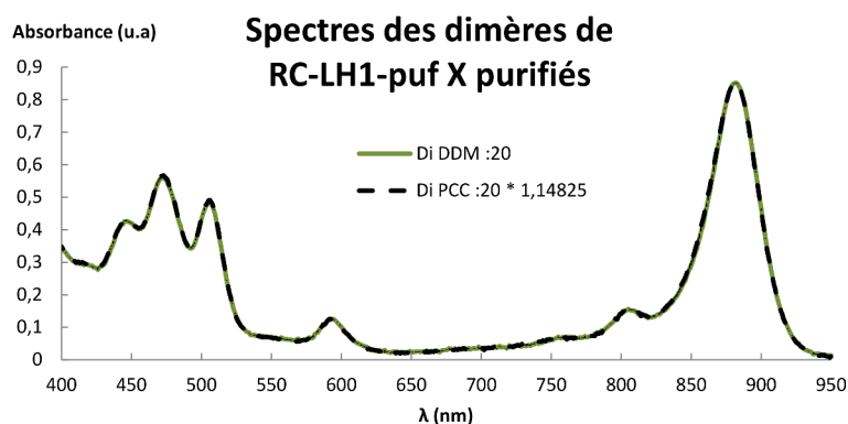
Figure 4.13 – Spectres d’absorbance du complexe RC-LH1-puf X solubilisé en DDM et PCC-malt, après purification sur colonne. Les spectres sont normalisés à la concentration pour une meilleure comparaison des signaux.
