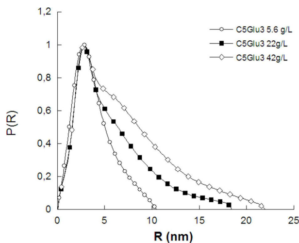
Figure 2.23 – fonction de distribution de paire du C5Glu3 à différentes concentrations
