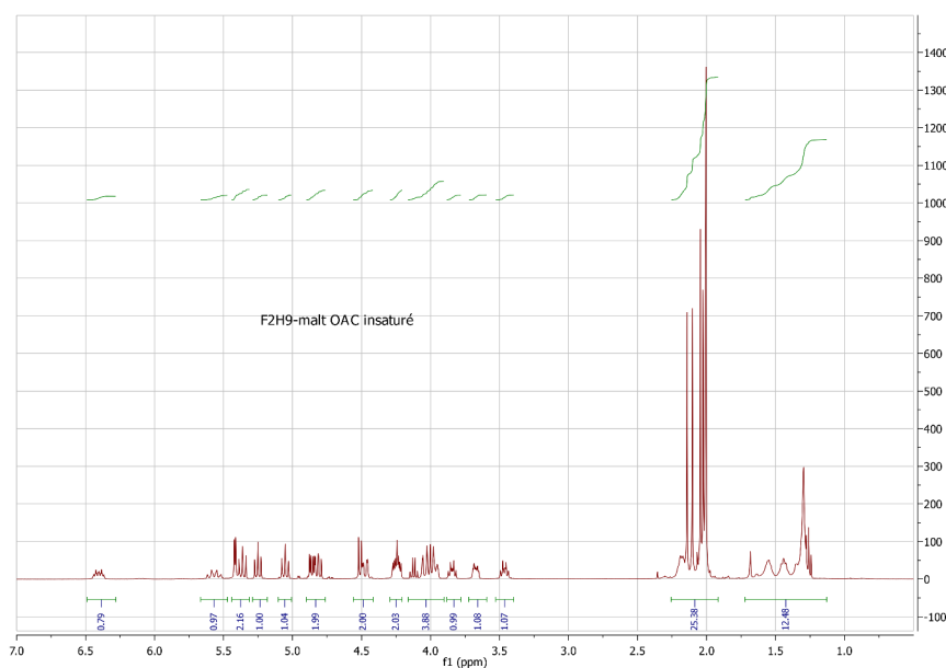
Figure 1.31 – Spectre ^1\text{H} -RMN du composé 26 . Les multiplets à 6,4 et 5,5 ppm sont caractéristique de la double liaison de la chaîne. L'interprétation complète du spectre est donné dans la partie expérimentale.
