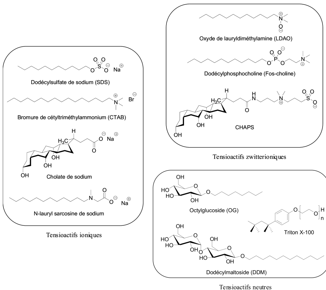
Figure 1.1 – Les différentes classes de tensioactifs : quelques exemples de structures de tensioactifs classées selon la nature de la tête polaire
