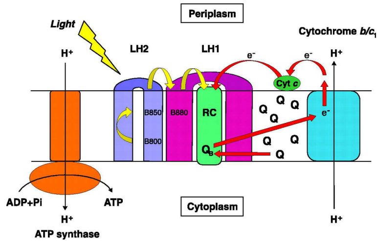
Figure 19 – Schématisation de la chaîne photosynthétique. Extrait [72]. Voir texte pour explication.
