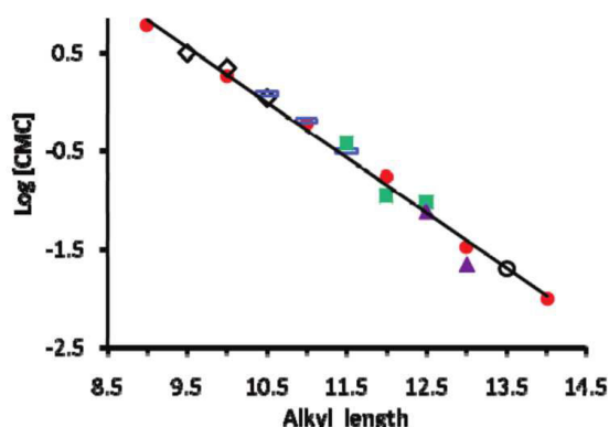
Figure 1.2 – Évolution de la CMC des composés maltoside en fonction de la longueur et de la ramification de la chaîne : le \log[\text{CMC}] (CMC en mM) est tracé en fonction du nombre de carbones dans la chaîne linéaire (cercles pleins) ou ramifiés, en comptant que un carbone de la ramification équivaut à 0,5 carbone de la chaîne principale. Les losanges correspondent aux tensioactifs ramifiés dont la chaîne principale compte 9 carbones, 10 carbones pour les rectangles, 11 pour les carrés, 12 pour triangles et 13 pour le cercle blanc [98].
