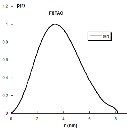
Figure 2.27 – Fonction de distribution de pair du F_8TAC
