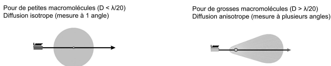
Figure 2.6 – La diffusion statique de la lumière
