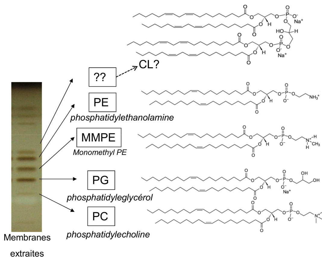
Figure 4.7 – Identification des bandes de lipides sur plaque HPTLC. Profil d'élué HPTLC d'extraits de membranes de Rb. blasticus . Phase mobile : chloroforme/méthanol/acide acétique/eau (30/5,2/3,6/1,6 : v/v/v/v).
