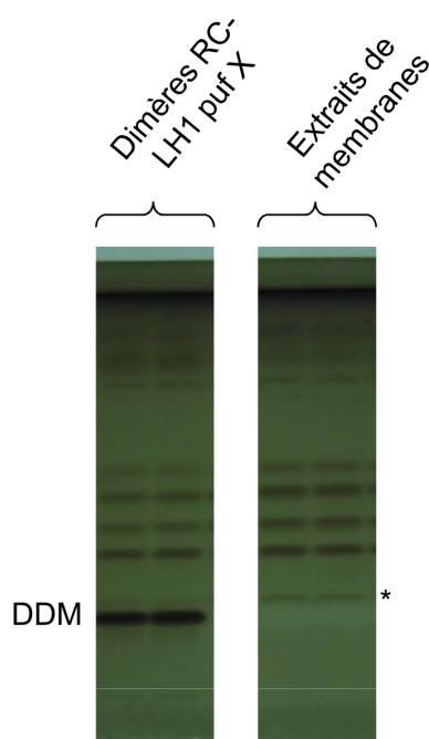
Figure 4.3 – Plaque HPTLC de l’analyse des lipides chez Rb. blasticus . Profils d’élution HPTLC d’extraits de dimères RC-LH1 pufX purifiés (gauches) et de membranes après cassage des cellules (droite). Phase mobile : chloroforme/méthanol/acide acétique/eau (30/5,2/3,6/1,6 : v/v/v/v)
