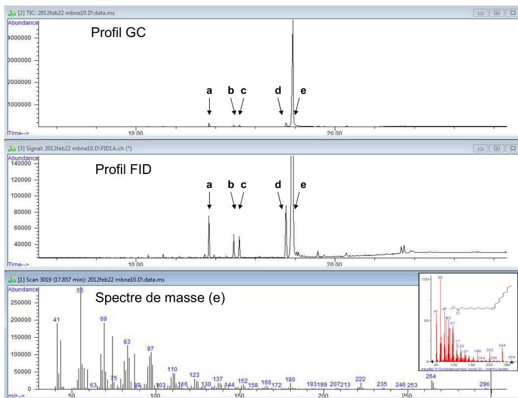
Figure 4.4 – Résultats de l’analyse GC-MS. Le profil d’élution en sortie de colonne de chromatographie gazeuse (haut), et le profil de détection par FID (milieu) indiquent la présence de 5 composés notés de a à e, qui peuvent être identifiés par fragmentation en spectrométrie de masse (bas) et comparaison à la base de donnée (spectre dans l’insert). Les composés sont des méthylesters en C15:0 (a), C16:0 (b), C16:1 (c), C18:0 (d) et C18:1 (e).
