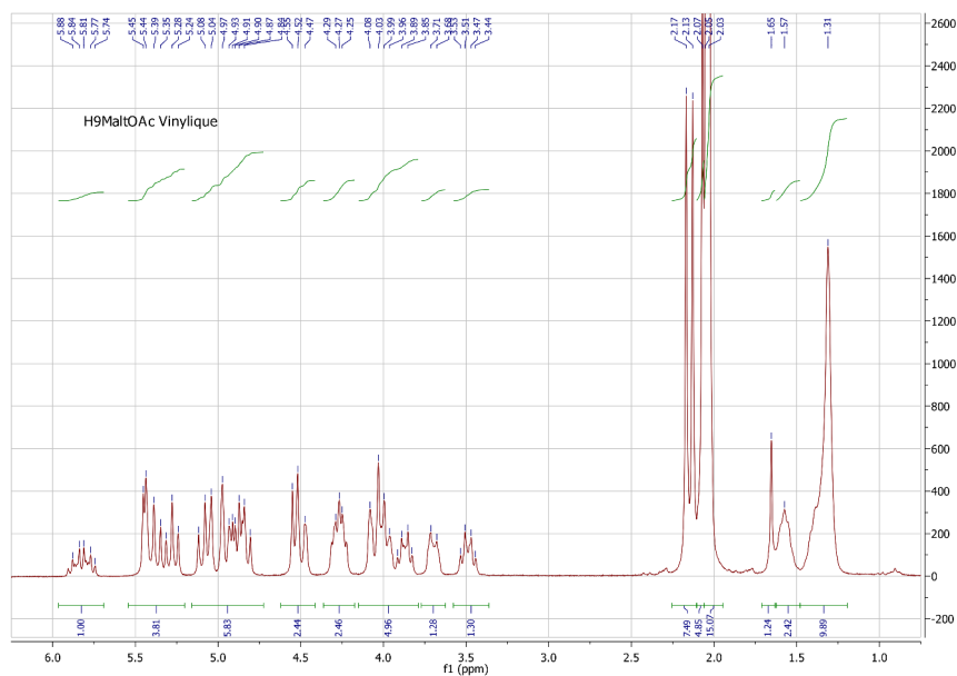
Figure 1.29 – Spectre ^1\text{H} -RMN du composé 23 . Le proton \text{H}_1 est axial, ( \delta=4,521\text{-}4,501 ppm, J(\text{H}_1\text{-H}_2)=8 Hz sur RMN 400 MHz), le composé 23 est \beta . Le signal à 5,5 ppm est caractéristique de la fonction vinyle. L'interprétation complète du spectre est donné dans la partie expérimentale.
