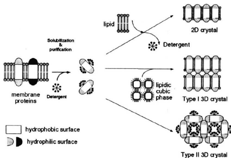
Figure 7 – Cristallisation des protéines membranaires. Extrait de [15]
