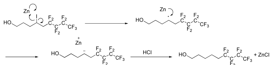
Figure 1.25 – Mécanisme de réduction de l'iodure.
