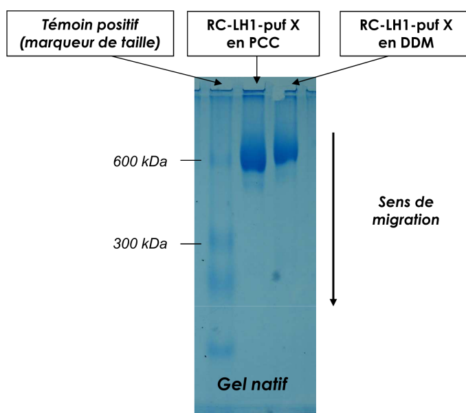
Figure 4.14 – Gel natif du RC-LH1 puf X en DDM et en PCC-malt. Le complexe protéique solubilisé en PCC-malt (piste du milieu) est plus petit que le complexe protéique avec une bouée de DDM
