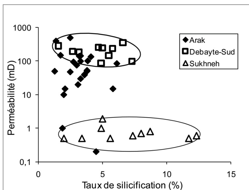
Figure III.36 : Perméabilité vs. taux de silicification des grès carbonifères du bassin des Palmyrides-Sud.
