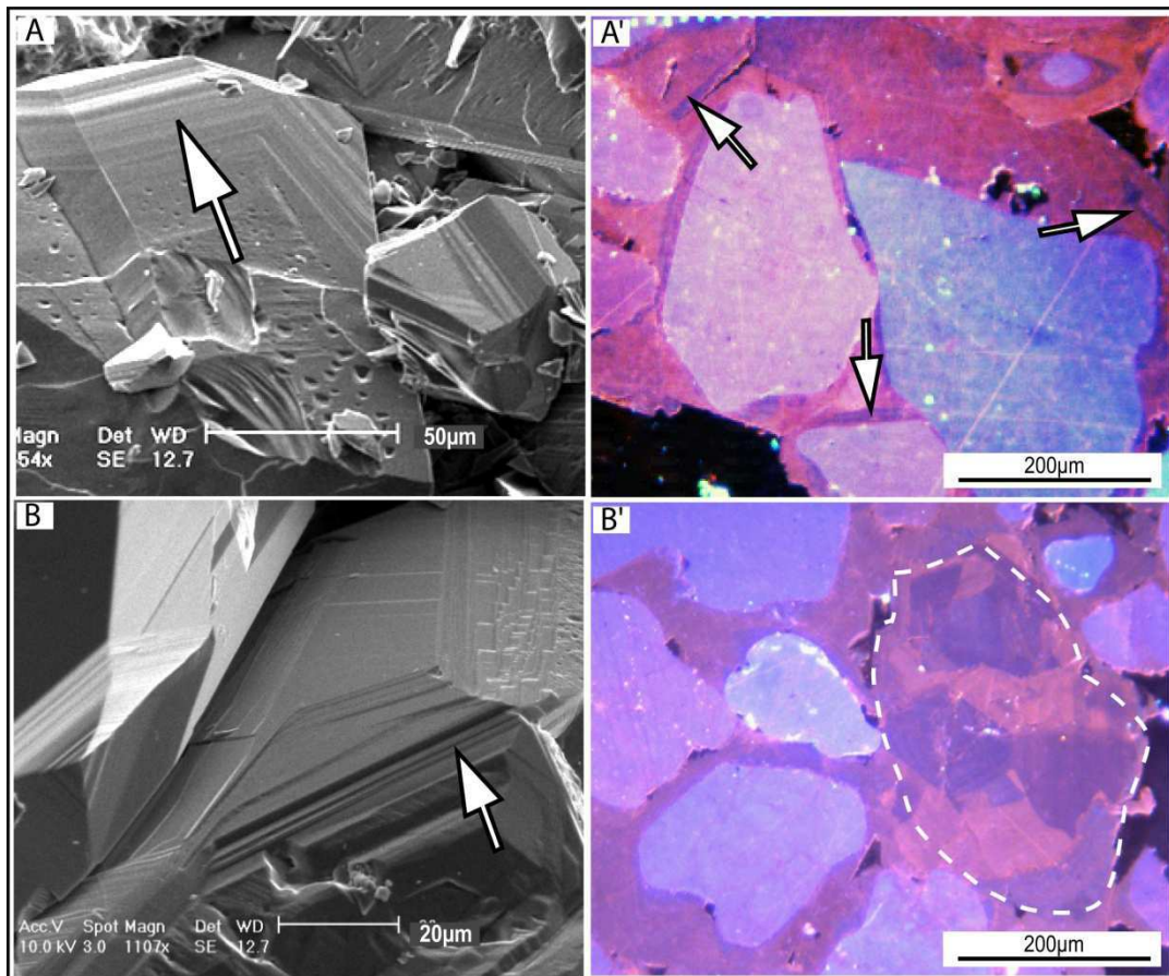
Figure V.24 : Zonalité et zones de croissance en escaliers dans la base de la paléozone à gaz. (A) Puits ODZ6 à 2442,8m (MEB), zonalité concentrique observée dans une section d'une auréole de la silicification et distinguée par l'alternance des bandes grises sombres et claires (flèche blanche). (A') Puits ODZ6 à 2442,8m (CL), partielle zonalité chimique dans les auréoles de silicification (flèches blanches). (B) Puits ODZ6 à 2442,8m (MEB), zones de croissance en escaliers développées sur une face cristalline (flèche blanche). (B') Puits ODZ6 à 2442,8m (CL), occurrence de troisième phase Q3 de ciment de quartz (ligne pointillée) en remplissage de la porosité résiduelle. Une variation de luminescence a eu lieu au cours de croissance de Q3.
