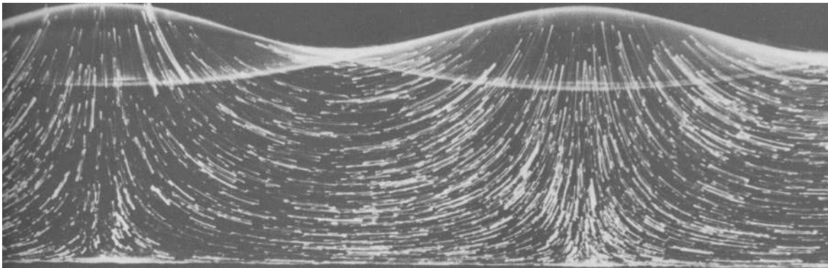
FIGURE 1.5 – Mouvement des particules de fluide dans une onde plane stationnaire en eau peu profonde. Les orbites sont d'aire nulle dans la description linéaire d'après Van Dyke [14].
