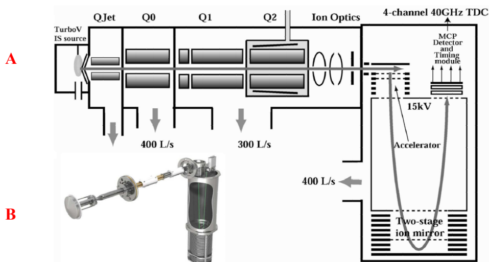
Figure 94 : (A) Illustration détaillée de l'instrument Triple TOF 5600 (AB SCIEX) (B) Image de la machine
