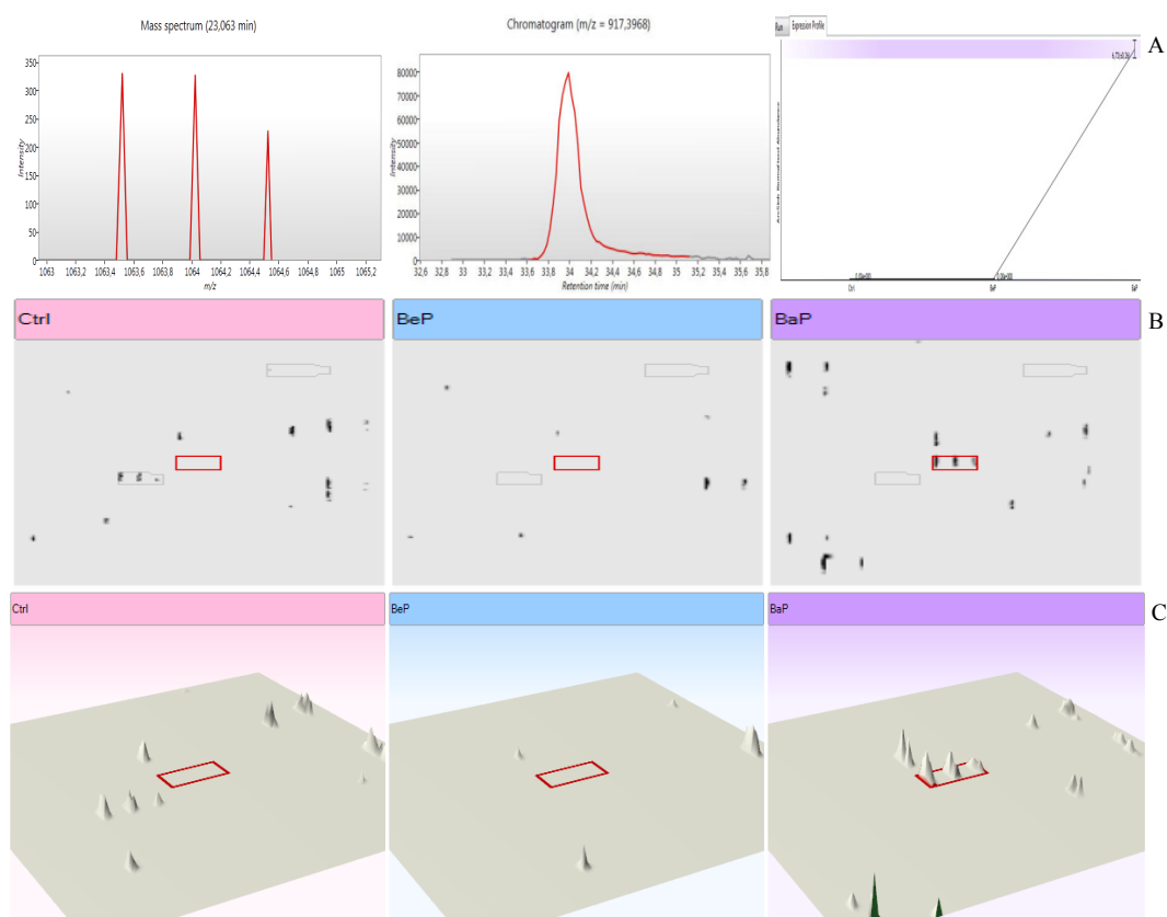
Figure 75 : Représentation schématique du XIC : (A) 1D, (B) 2D, (C) 3D
