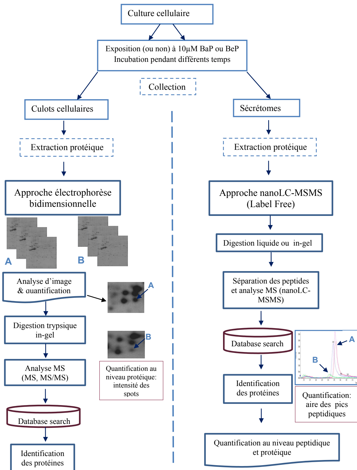
Figure 96 : Approches protéomiques développées
