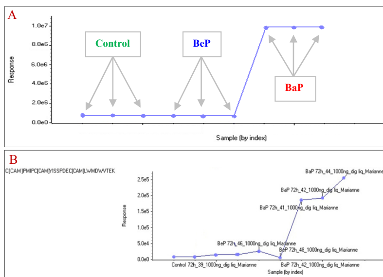
Figure 60 : Exemple de profil de régulation (appelé plot profile) tel que ceux générés dans MarkerView : A = profil caractéristique d'un peptide ou protéine qui ne serait exprimé(e) que dans la condition BaP; B = profil obtenu pour le peptide C*PMIPC*YISSPDEC*LWMDWVTEK de la protéine TIMP2_HUMAN et très proche du profil attendu décrit dans la partie A
