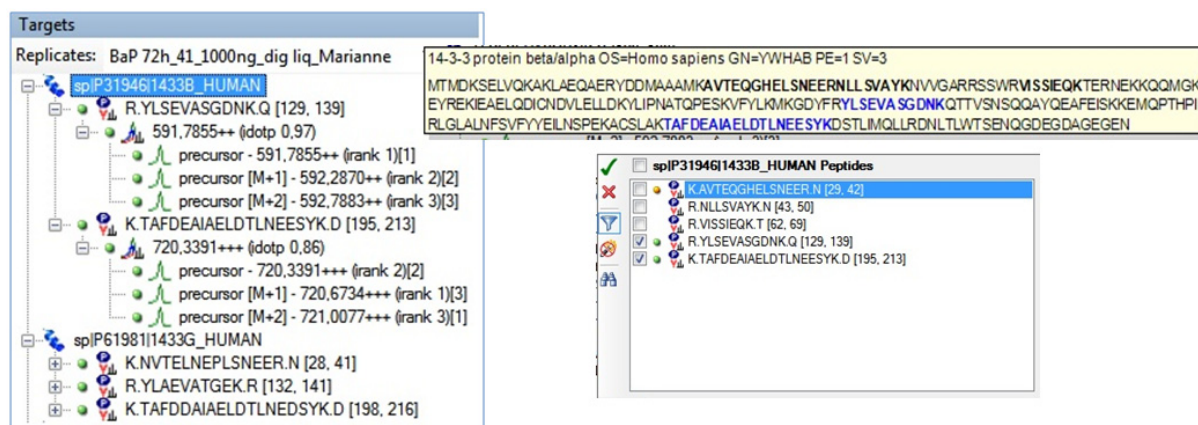
Figure 66 : Arborescence générée par l'import du fichier .fasta dans Skyline. Exemple de la protéine 1433B_HUMAN : 2 peptides présents de la librairie ( m/z 591.7855 et m/z 720.3391), 2 et 3 fois chargés respectivement/ La description de la protéine et le positionnement des résidus identifiés est visualisable dans une première fenêtre pop-up. Les autres peptides répondant aux critères de filtre sont mentionnés dans une seconde fenêtre pop-up (ils ne sont cochés que s'ils sont détectés dans la librairie).
